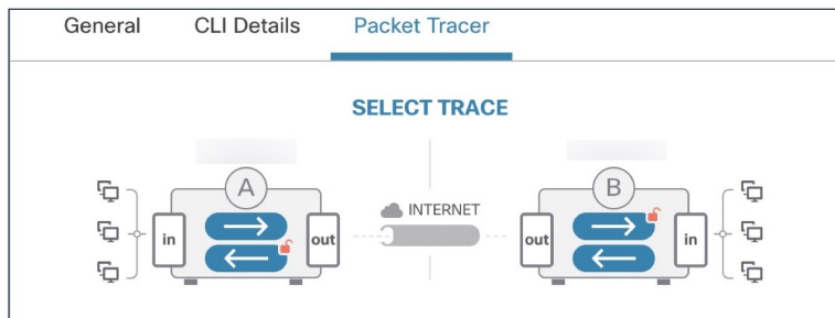
图 2: Packet Tracer
