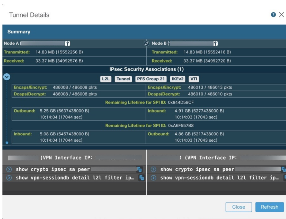
图 1:隧道状态 > 查看 > CLI 详细信息
