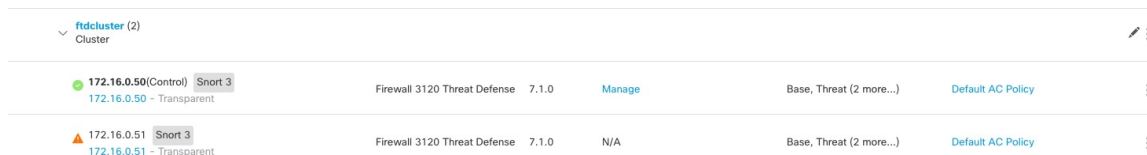
图 4: 集群管理
