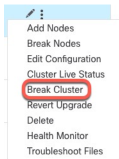
图 19: 中断集群
