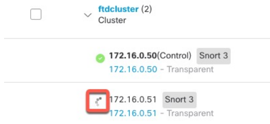
图 5: 节点注册
