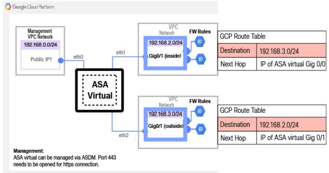
图 55: GCP 上的 ASA Virtual 部署示例
