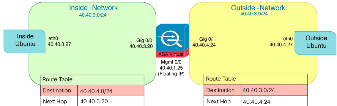
图 65: OpenStack 部署上的 ASA Virtual 示例
