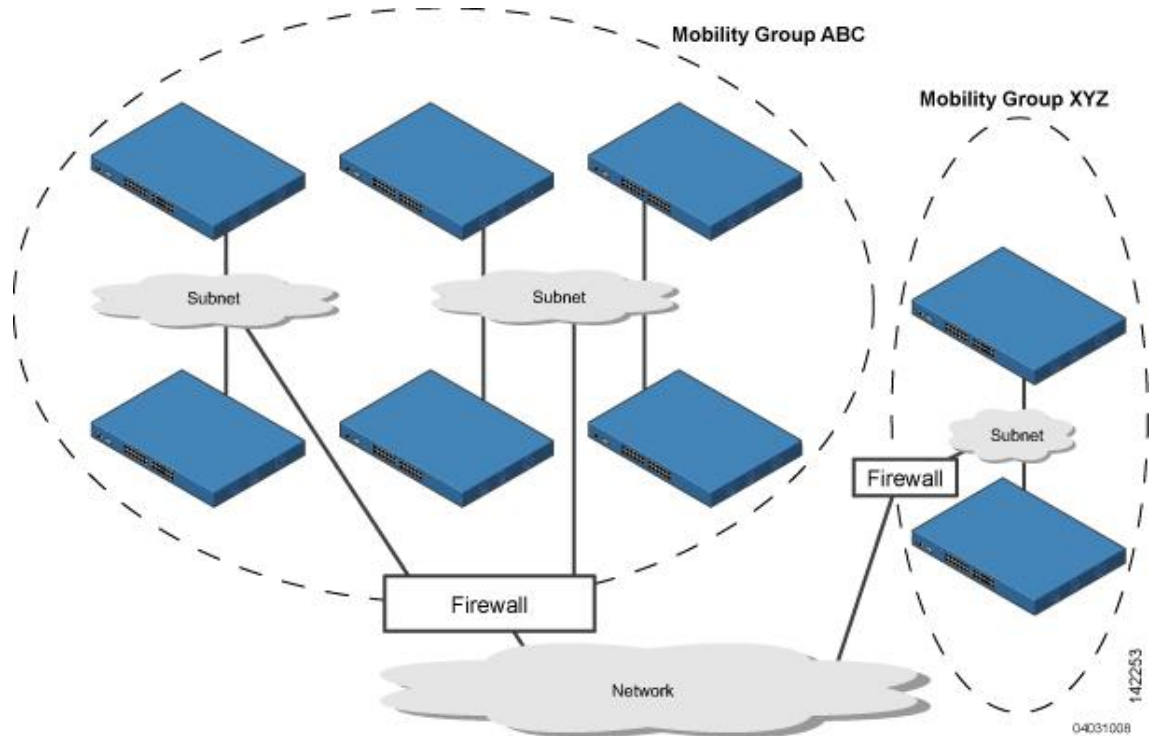
図 77: 2つのモビリティグループ
