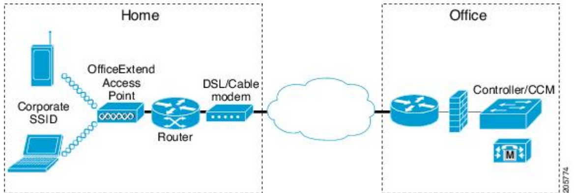
図 53: 一般的な OfficeExtend アクセス ポイント セットアップ
