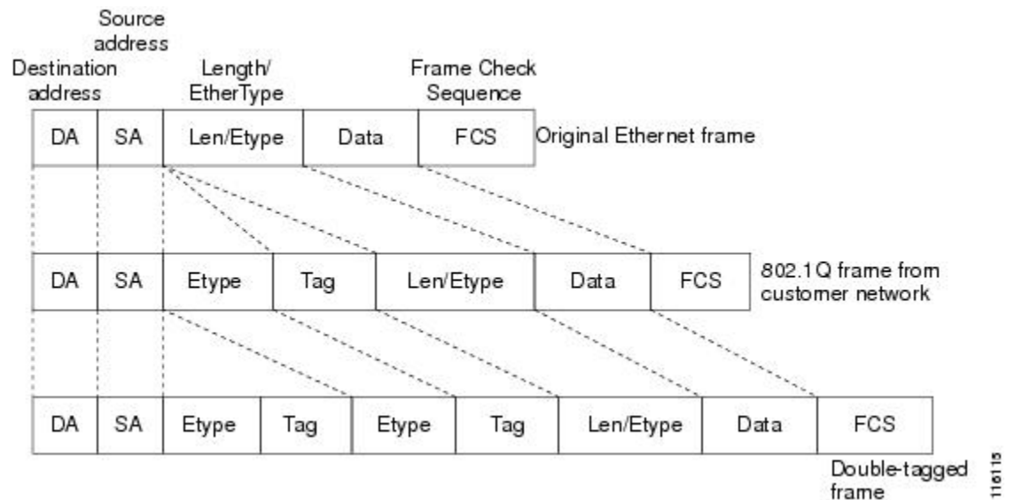
図 50: タグなし、802.1Q タグ付き、および 802.1Q-in-Q タグ付きのイーサネット フレーム
