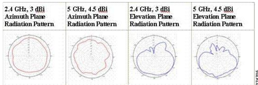
図 34 : OfficeExtend アクセスポイントの放射パターン
