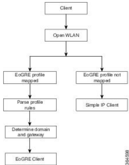
図 25: オープン認証ベースの WLAN の EoGRE ワークフロー
