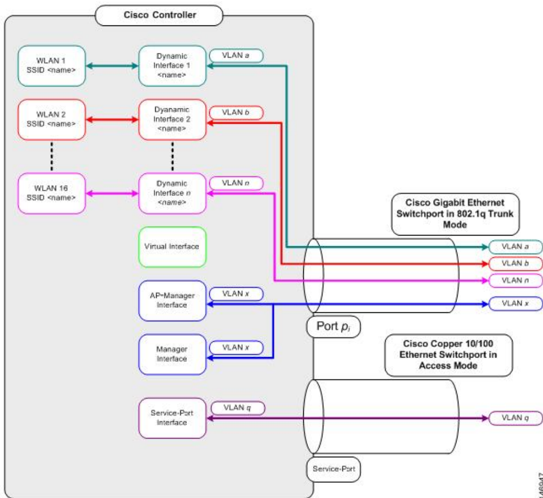
図 36: ポート、インターフェイス、および WLAN の関係
