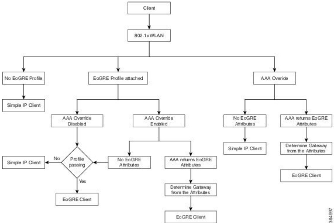
図 24 : 802.1X 認証ベースの WLAN の EoGRE ワークフロー
