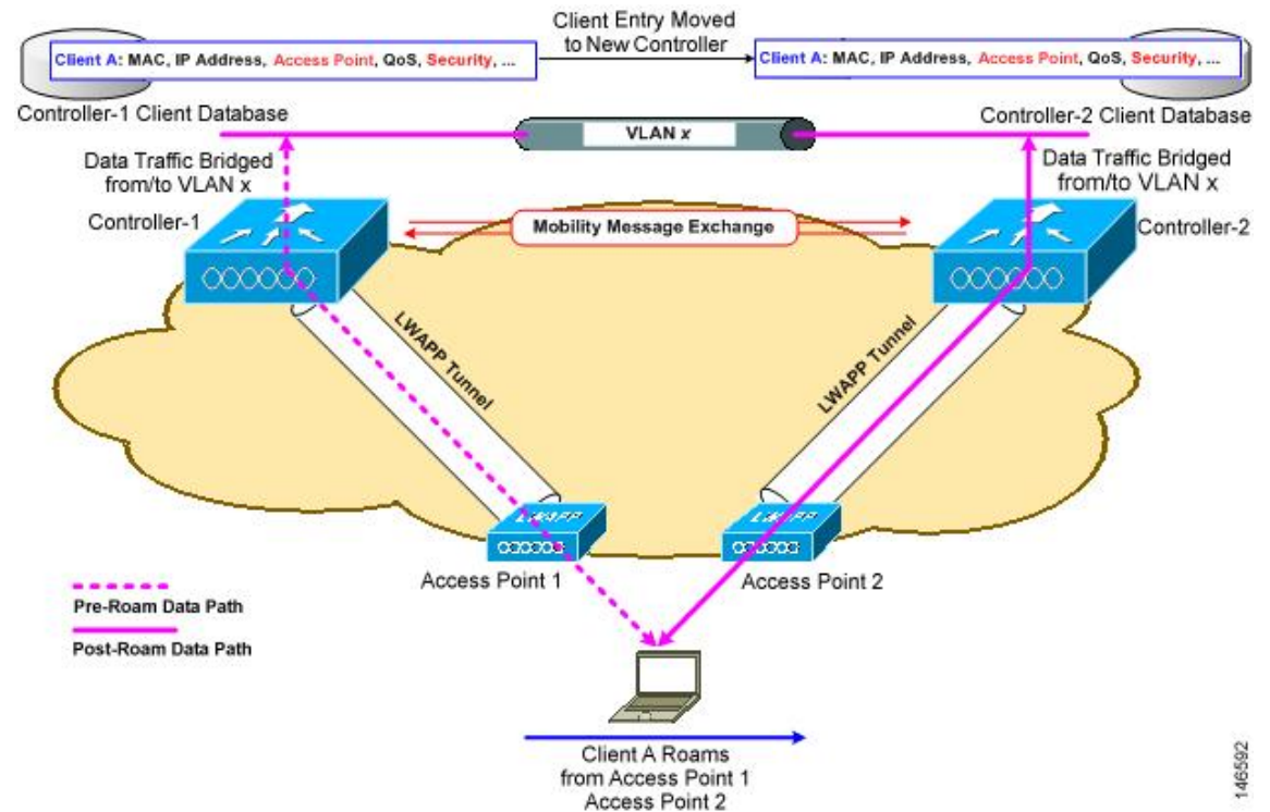
図 74: コントローラ間ローミング
