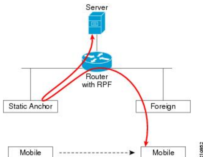
図 78: シンメトリック モビリティ トンネリングまたは双方向性トンネリング
