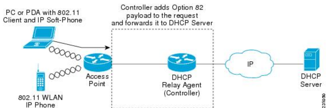
図 45: DHCP オプション 82
