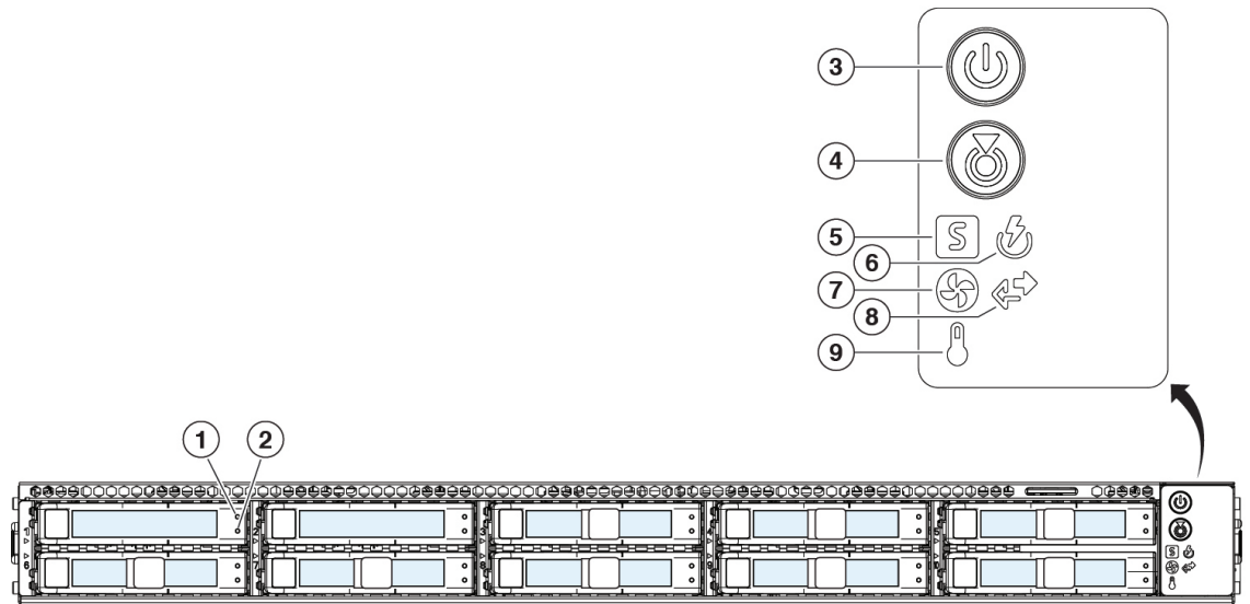
図 9: 前面パネル LED
