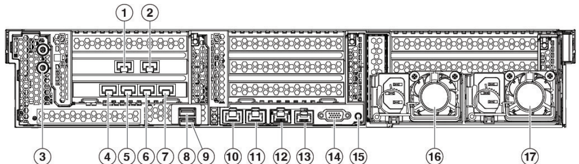
図 12: Cisco Secure Web Appliance S696F の背面パネル
