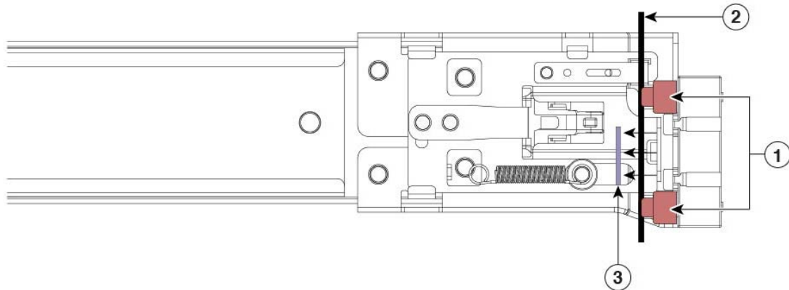
図 35: 前端的内側の前面固定のメカニズム
