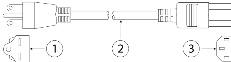
図 29: 北米 (CAB-N5K6A-NA)
