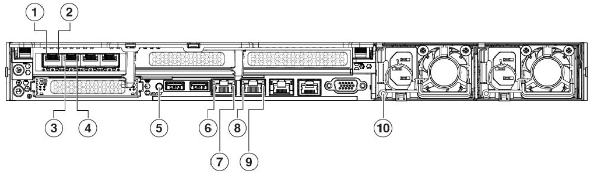
図 13: 背面パネル LED
