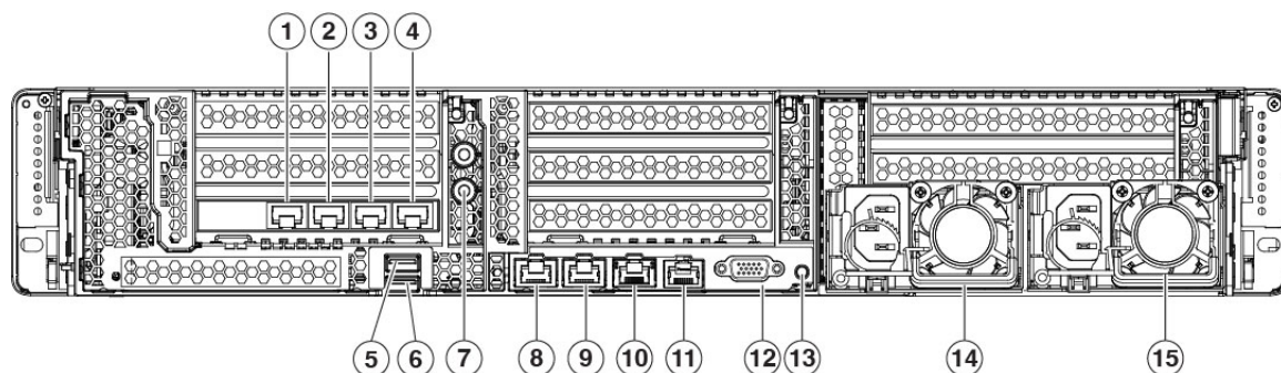
図 11 : Cisco Secure Web Appliance S696 の背面パネル
