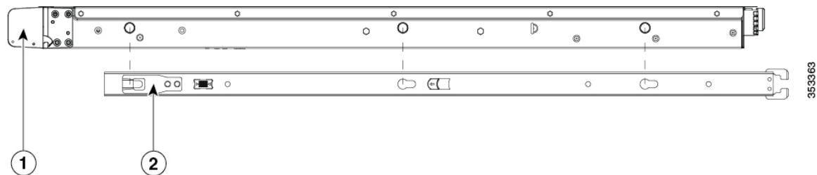
図 34: シャーシ側面への内側レールの取り付け
