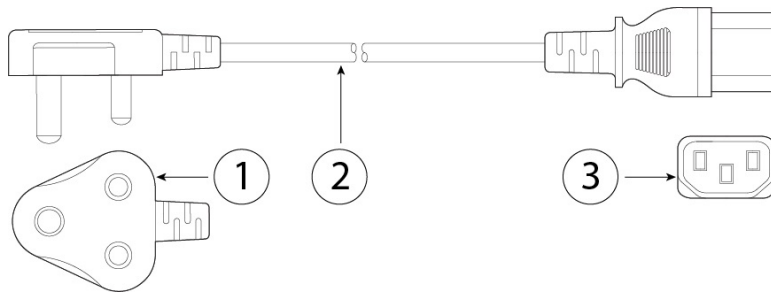
図 22: インド (CAB-250V-10A-ID)
