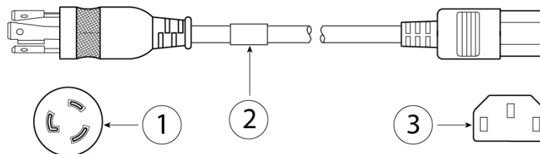
図 30: 北米 (CAB-AC-L620-C13)
