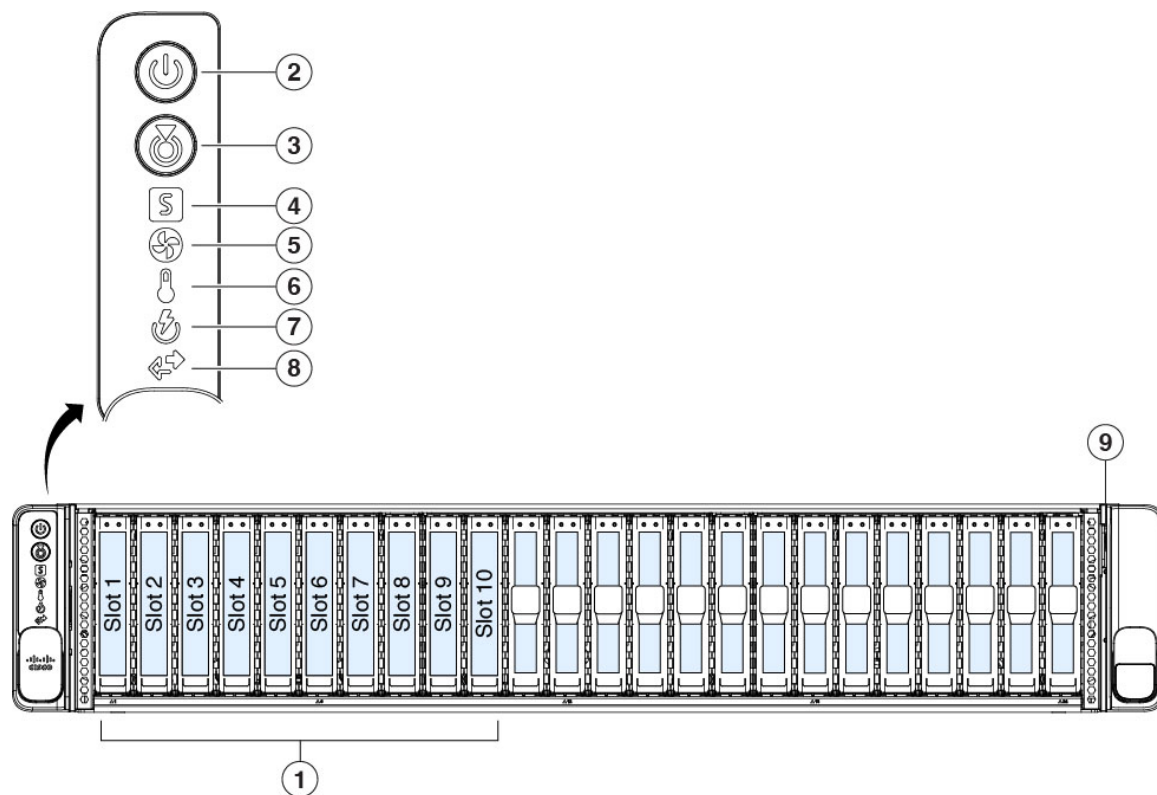
図 8: Cisco Secure Web Appliance S696 および S696F の前面パネル
