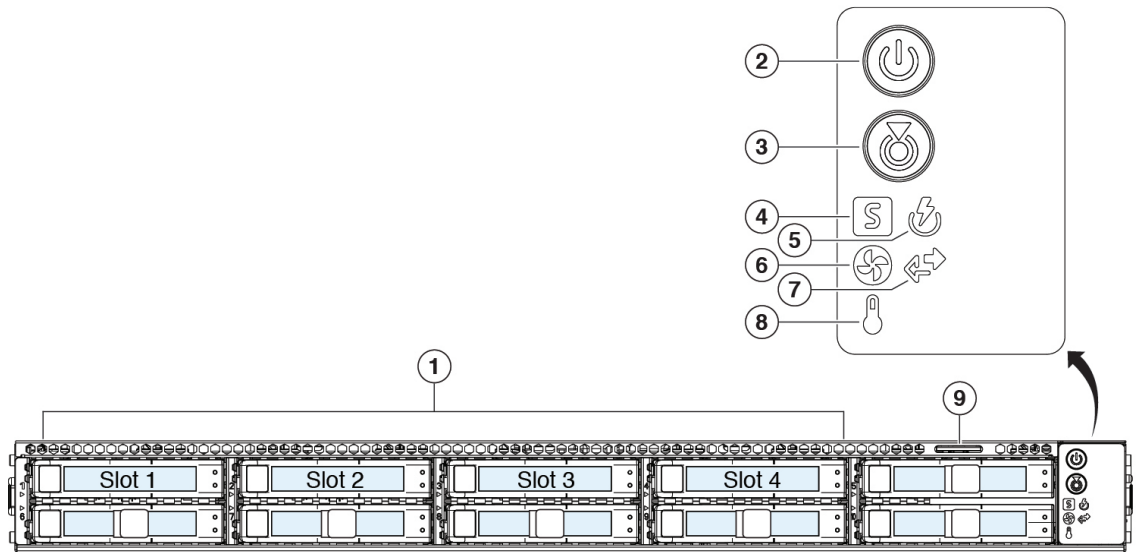
図 7: Cisco Secure Web Appliance S396 の前面パネル
