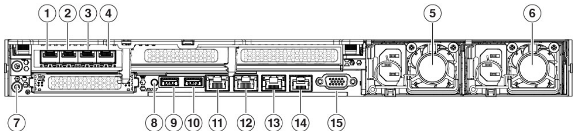
図 10: Cisco Secure Web Appliance S196 および S396 の背面パネル
