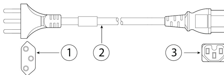
図 31: スイス (CAB-9K10A-SW)
