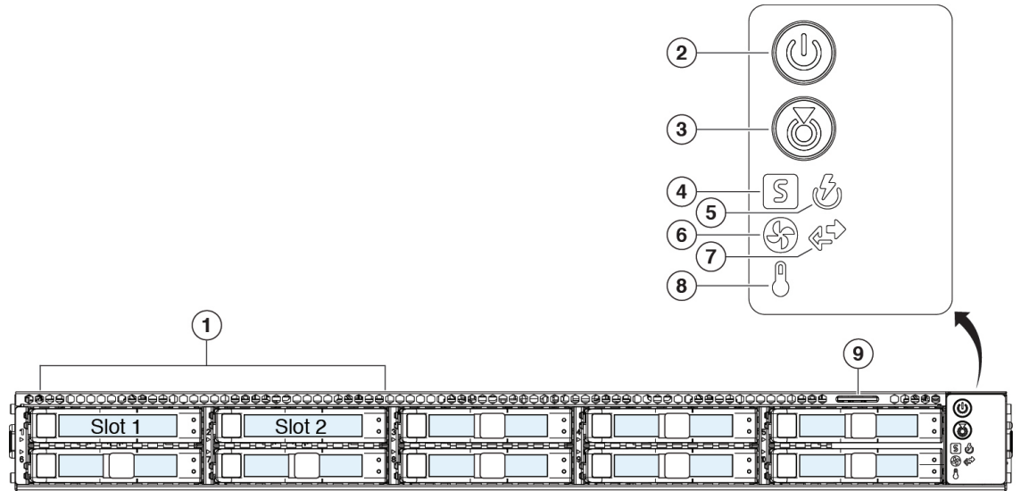
図 6: Cisco Secure Web Appliance S196 の前面パネル
