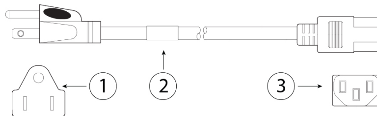
図 32: 台湾 (CAB-ACTW)
