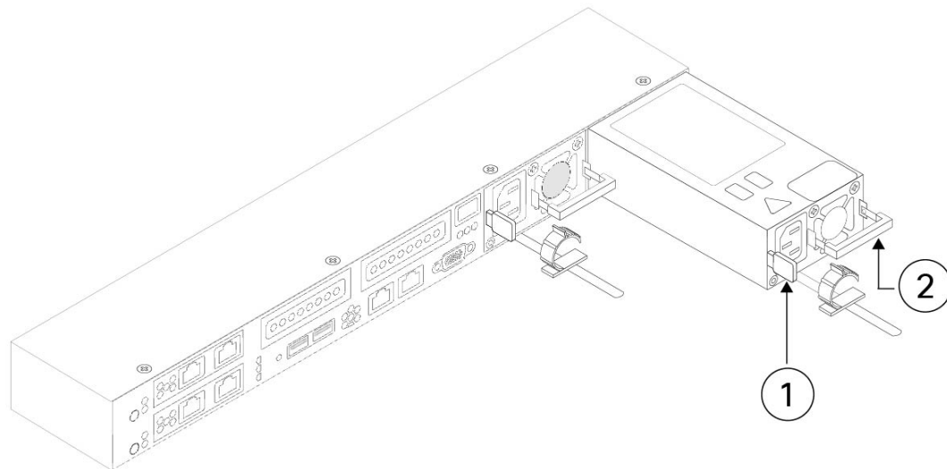
図 36: AC 電源装置の取り外しと交換
