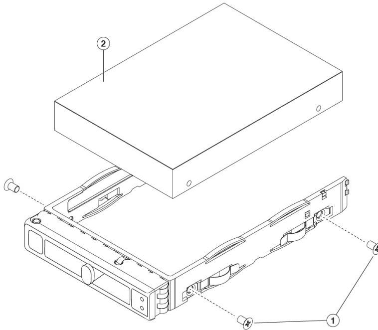
図 35: ドライブトレイの取り外し
