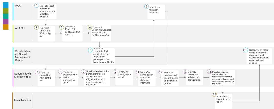
図 1: CDO の Firewall 移行ツールを使用した ASA から FTD への移行に関するエンドツーエンドの手順
