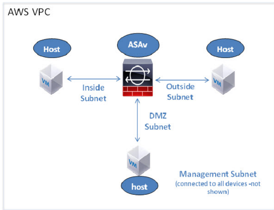
図 4: AWS への ASA の導入例
