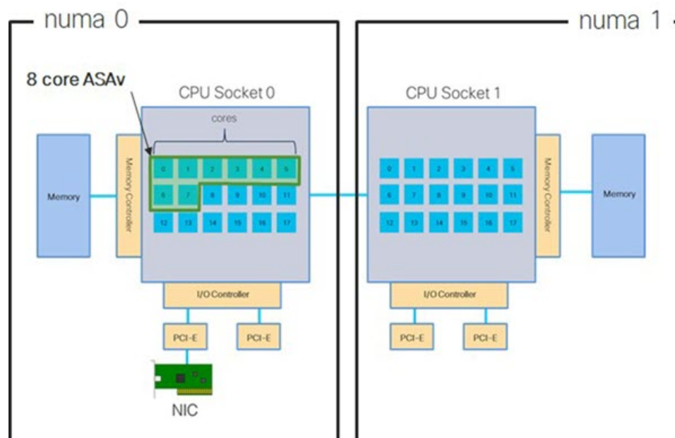
図 2: 8 コア ASA NUMA アーキテクチャの例
