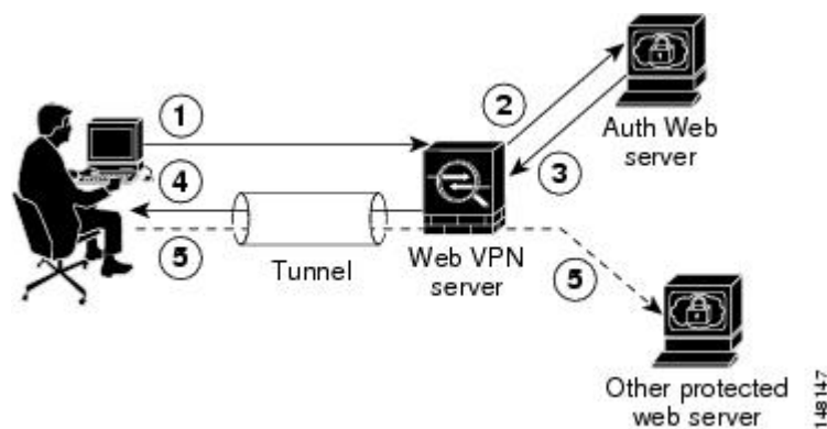
図 10: HTTP Form を使用した SSO 認証
