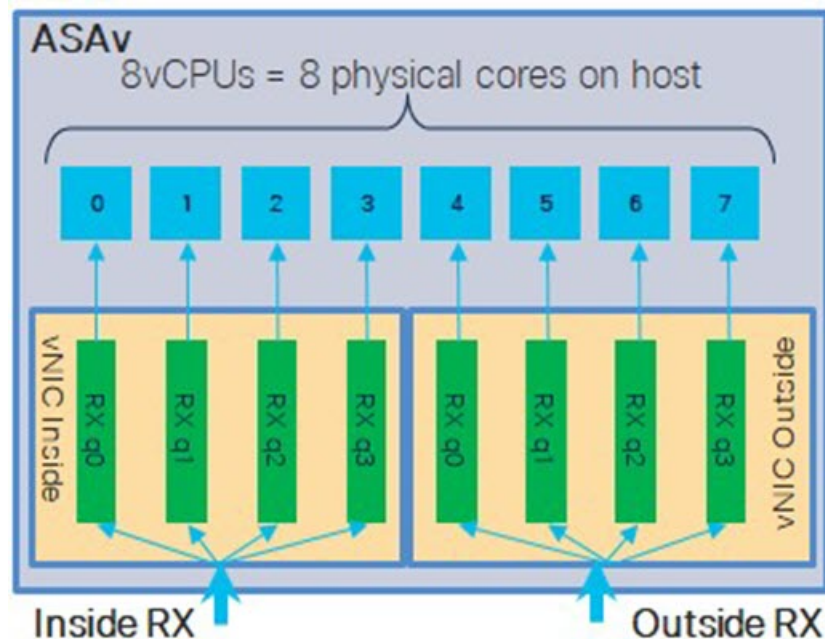
図 4: 8 コア ASA RSS RX キュー
