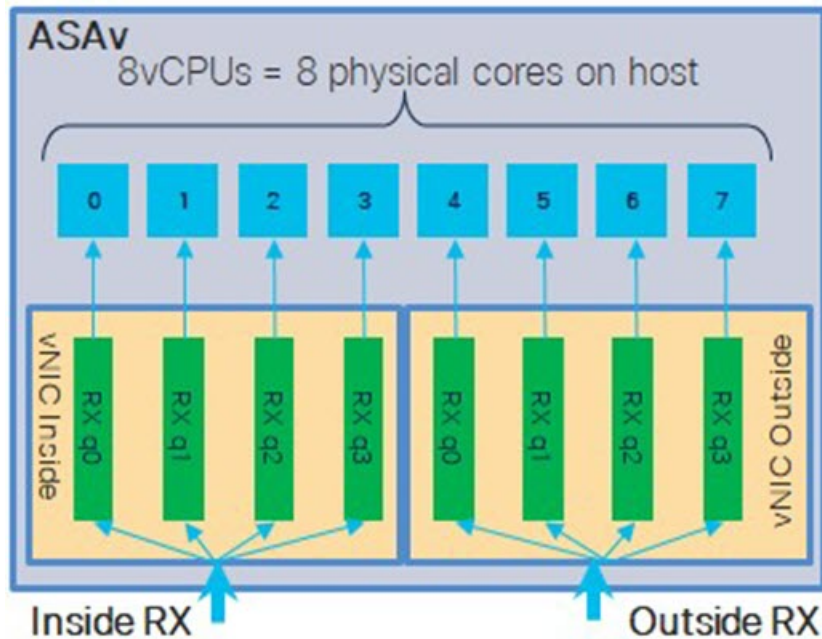
図 3: 8 コア ASAv RSS RX キュー
