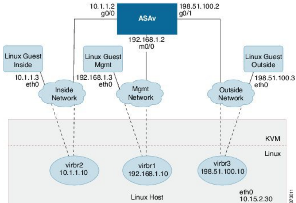
図 4: KVM を使用した ASA の導入例
