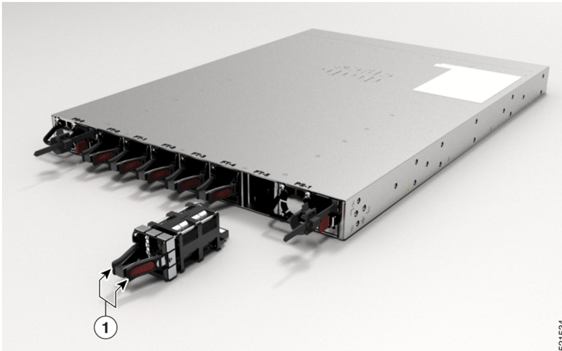
図 111: NCS 57B1 シャーシからのファンモジュールの取り外し
