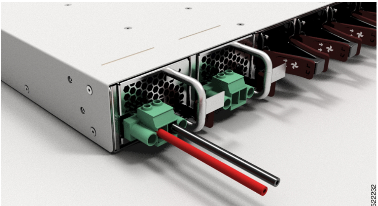
図 95: NCS-57C1 - DC 電源ケーブルの接続
