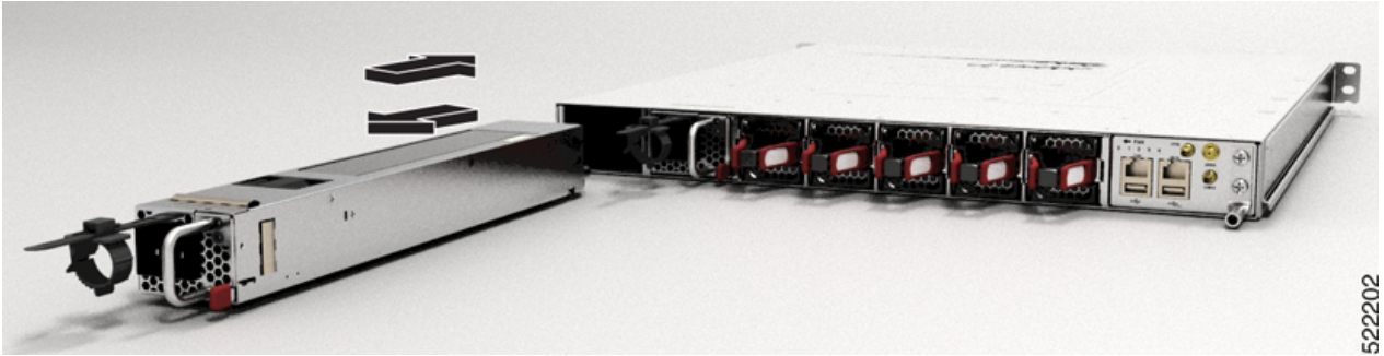
図 121: NCS-57C3-MOD - AC 電源モジュールの取り付け
