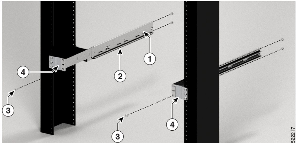
図 39: 23インチ2支柱ラックのラックマウントスライダアセンブリ
