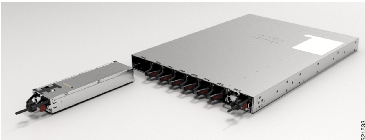
図 119: NCS-57B1 - AC 電源モジュールの取り付け
