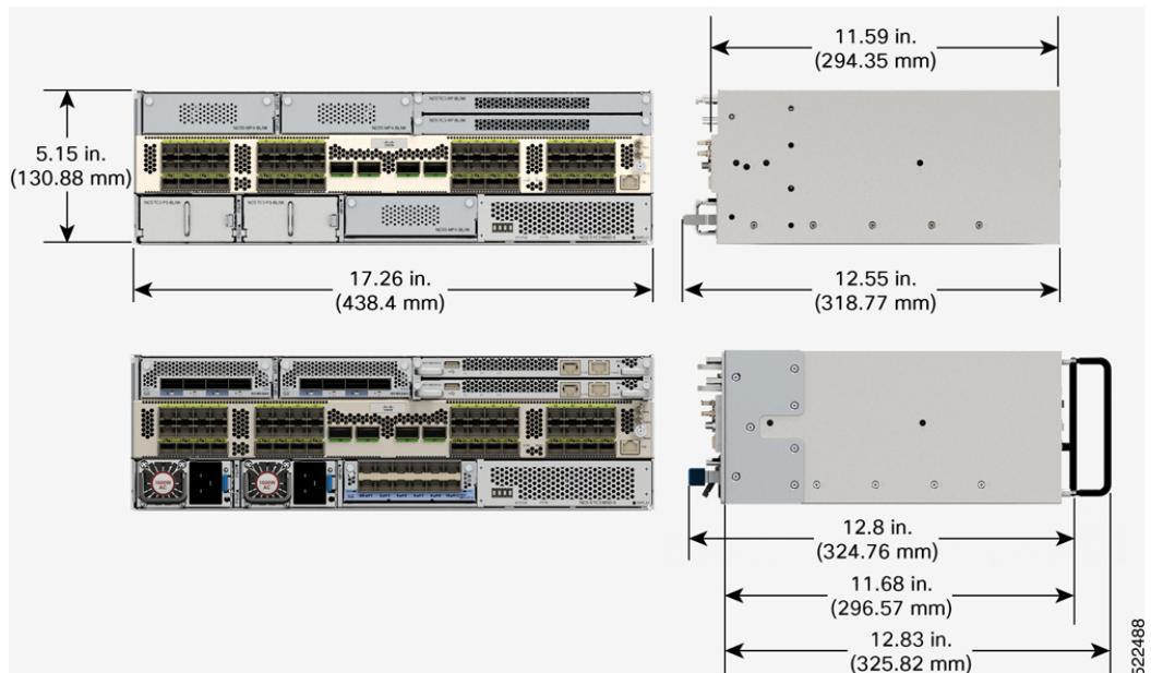
図 1: NCS-57C3-MOD の寸法
