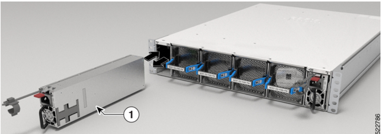
図 122: NCS-57D2 - AC 電源モジュールの取り付け
