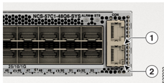
図 132: NCS-57C1 管理ポートの LED
