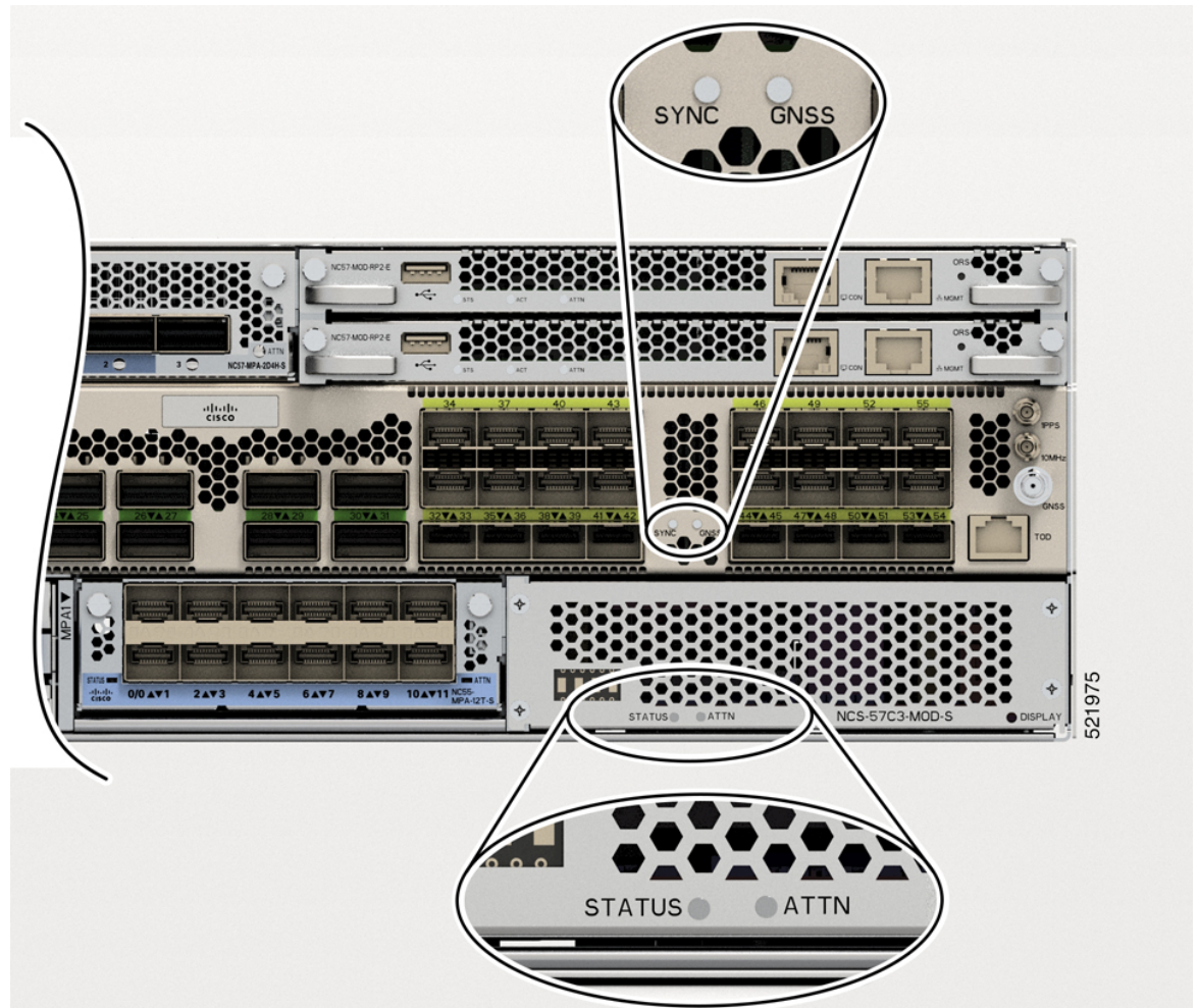
図 126: NCS-57C3-MOD シャーシの LED
