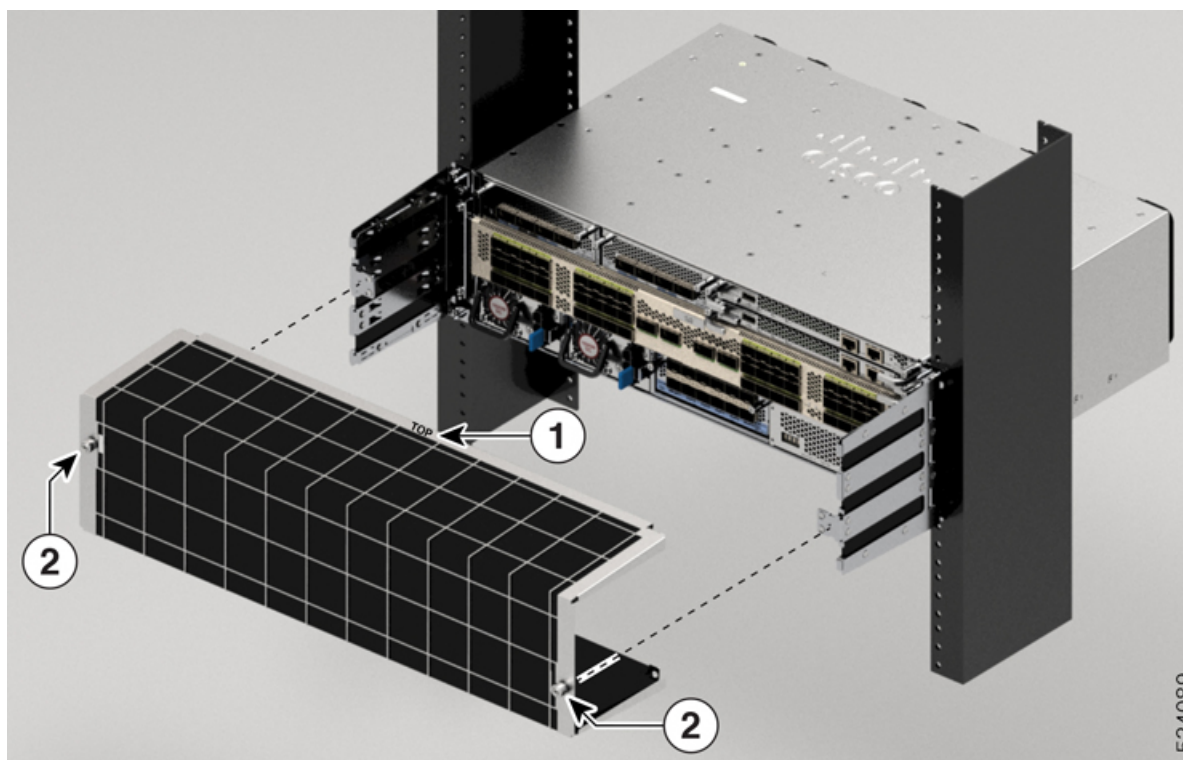
図 83: エアーフィルタの取り付け
