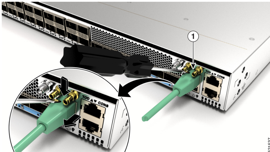
図 96: タイミングポートの間へのドライバの挿入
