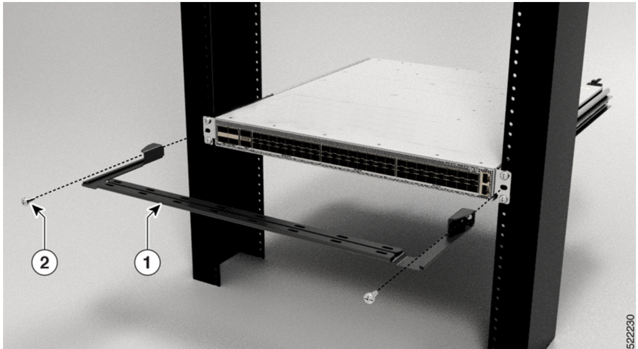
図 84: NCS-57C1 シャーシへのケーブル管理ブラケットの取り付け
