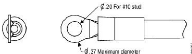
図 90: DC 入力電源ケーブル用端子
