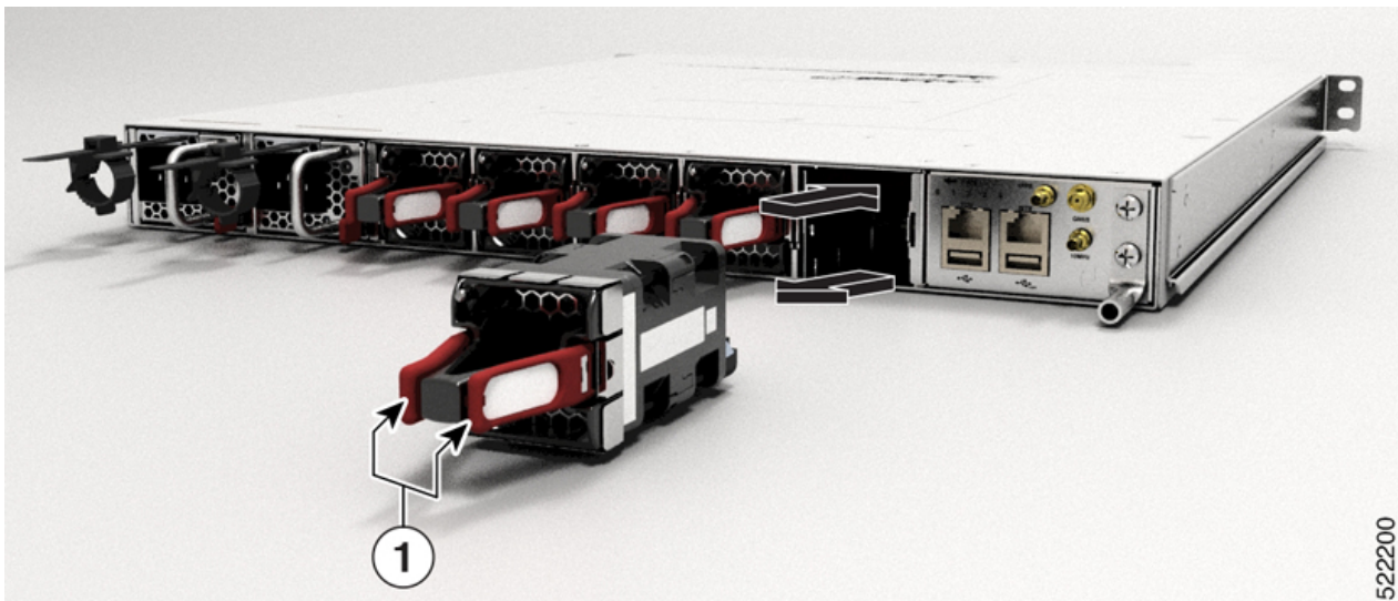
図 112: NCS-57C1 シャーシからのファンモジュールの取り外し
