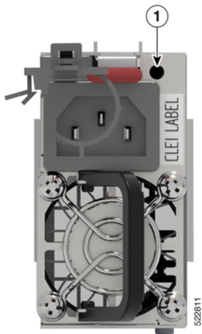
図 138: NCS-57D2 DC 電源モジュール
