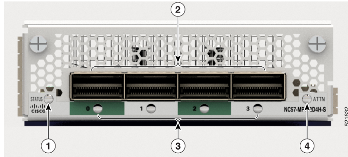
図 11: NCS57-MPA-2D4H-S モジュラポートアダプタ (MPA)
