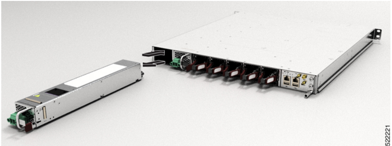
図 118: NCS-57D2 - DC 電源モジュールの取り付け
