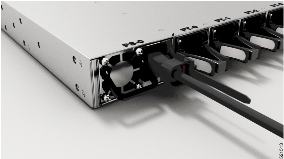
図 89: ケーブルクランプ: 例
