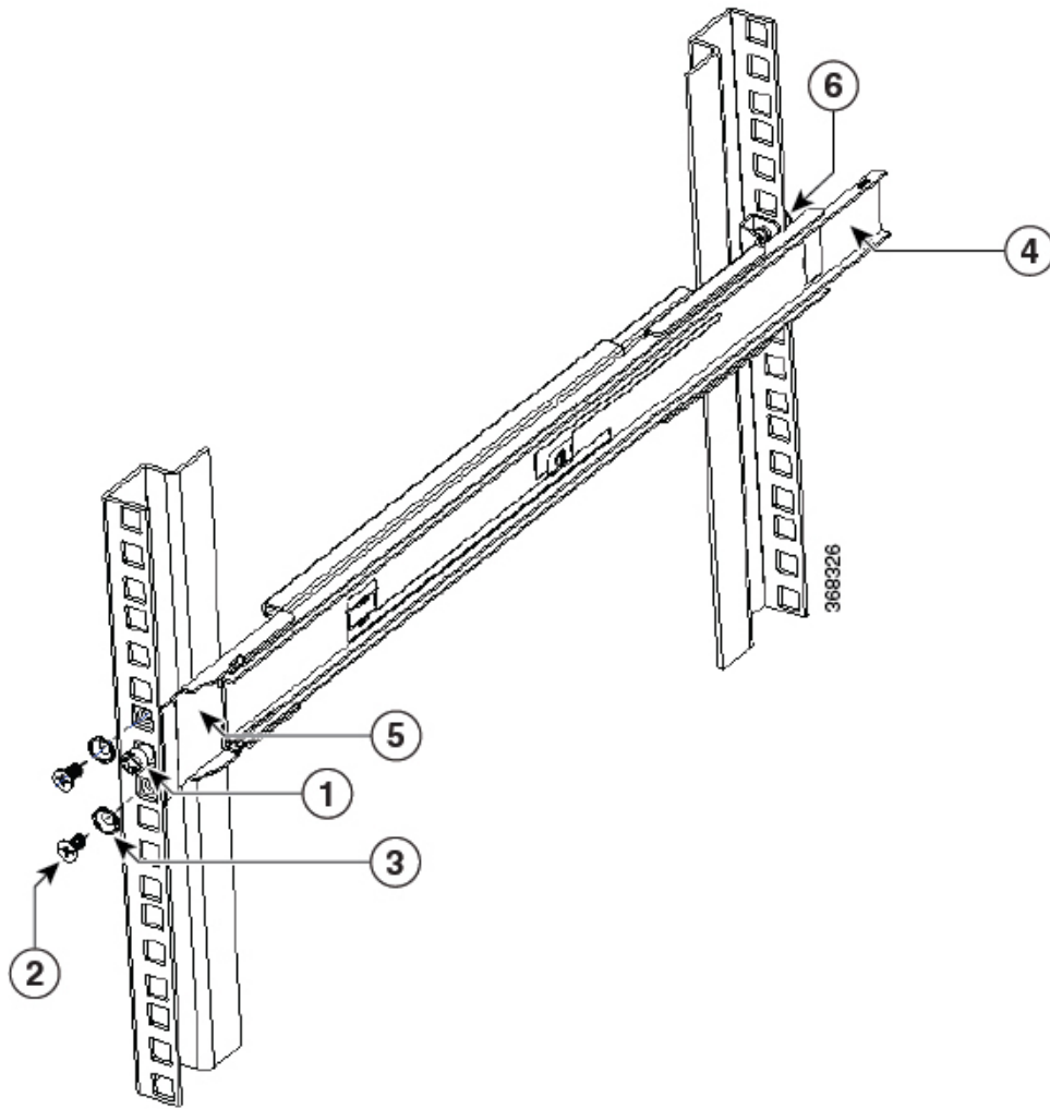
図 62: 外側スライダメンバのリアエンドおよびフロントエンド (NC55-2RU-ACC-SL2)
