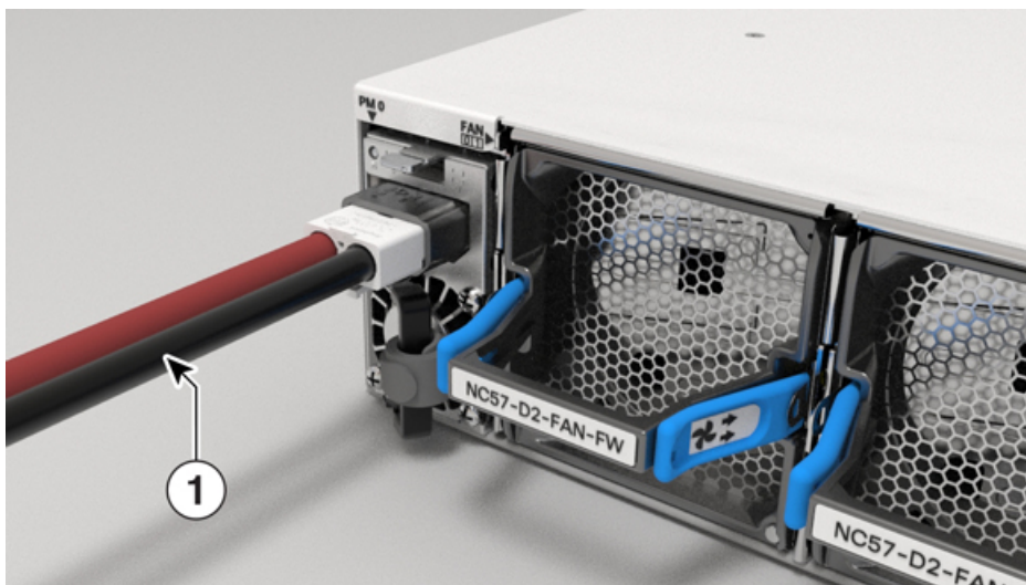
図 93: NCS-57D2 - DC 電源ケーブルの接続
