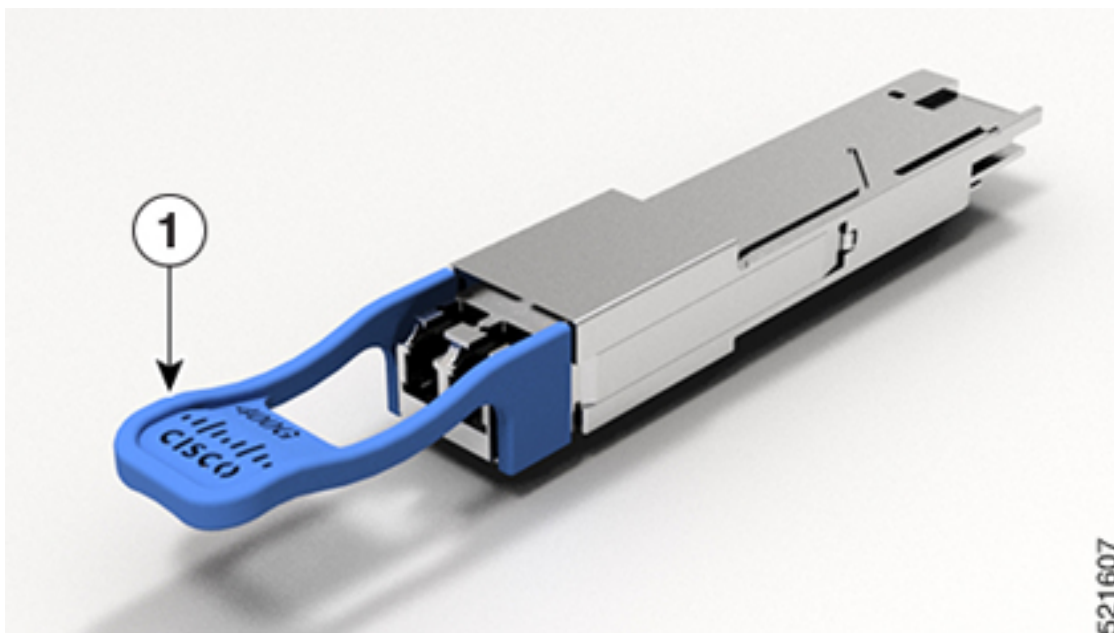
図 102: 400 ギガビット QSFP-DD トランシーバモジュール - 前面
