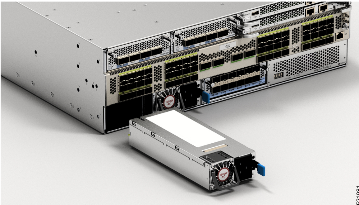
図 122: NCS-57D2 - AC 電源モジュールの取り付け
