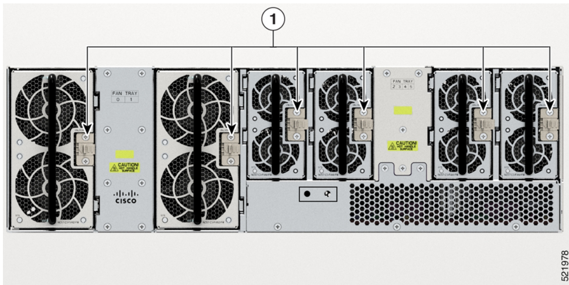
図 114: NCS-57C3-MOD シャーシからのファントレイの取り外し
