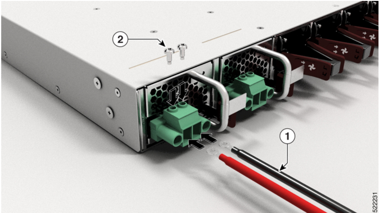
図 94: NCS-57C1 - DC 電源ケーブルの接続
