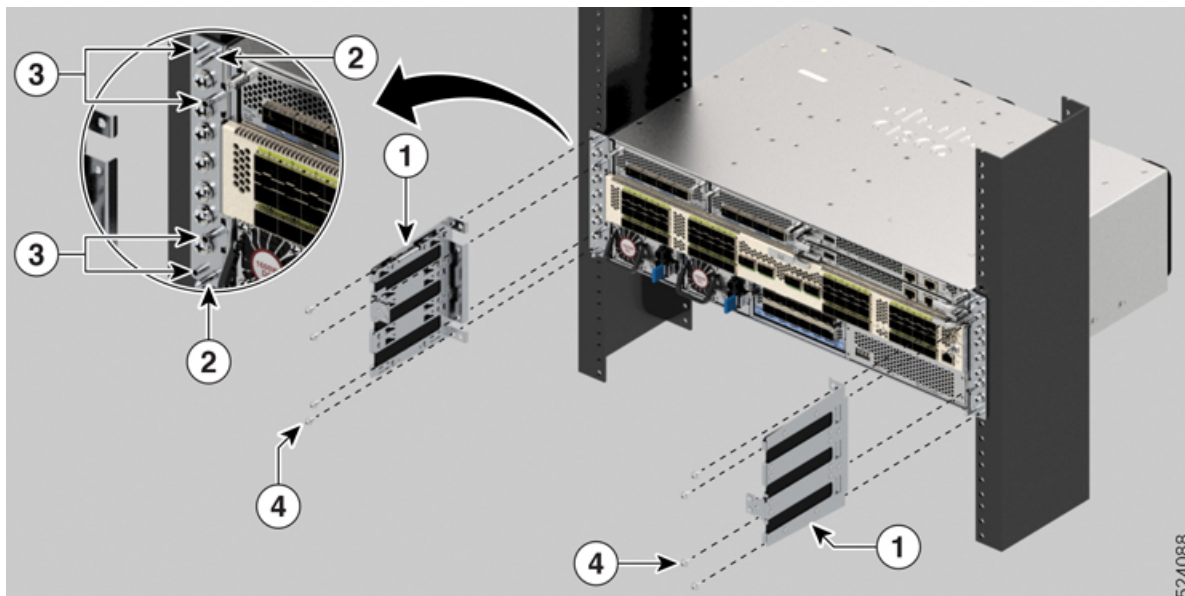
図 82: エア フィルタ サポート ブラケットの位置合わせと取り付け
