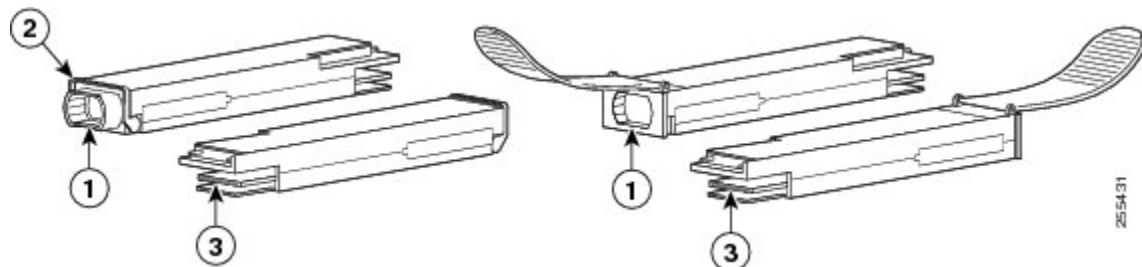
図 105: 40 ギガビット QSFP+ トランシーバモジュール (光ファイバ)
