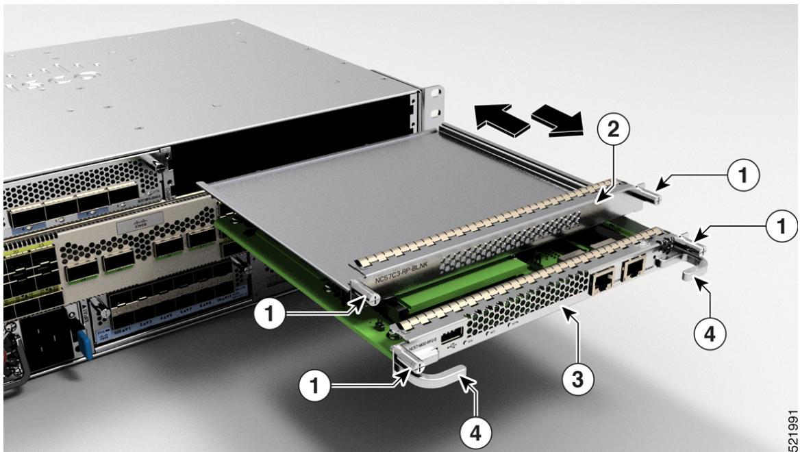
図 123: シャーシからの RP およびブランクの取り外し
