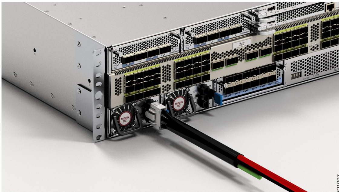
図 93: NCS-57D2 - DC 電源ケーブルの接続
