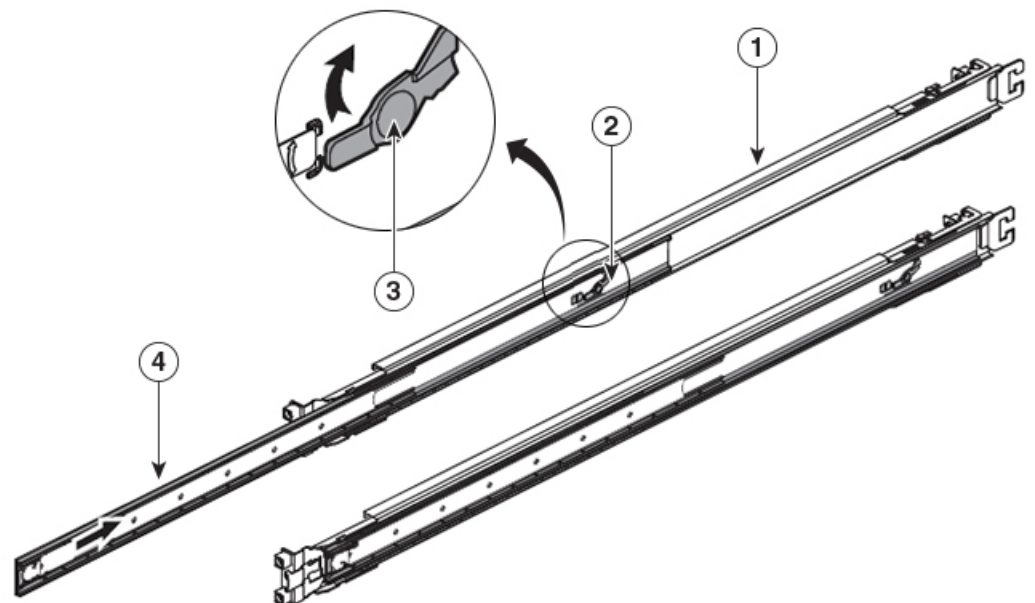
図 57: スライダアセンブリ
