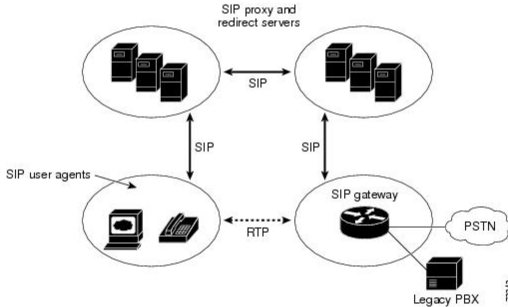
图 2: SIP 架构
