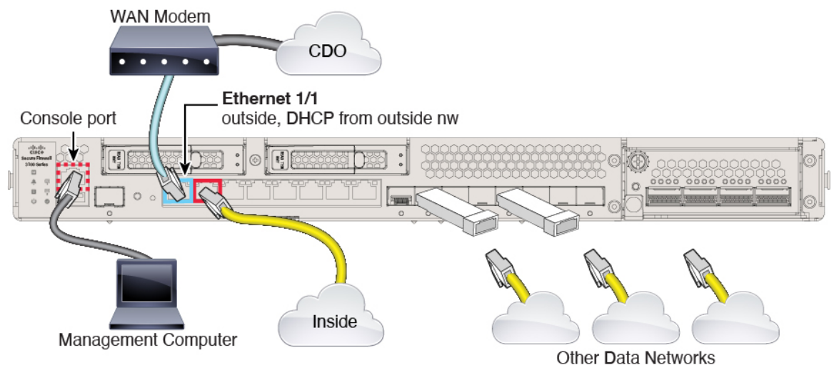
图 8: Secure Firewall 3100 布线
