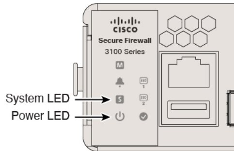
图 12: 系统和电源 LED
