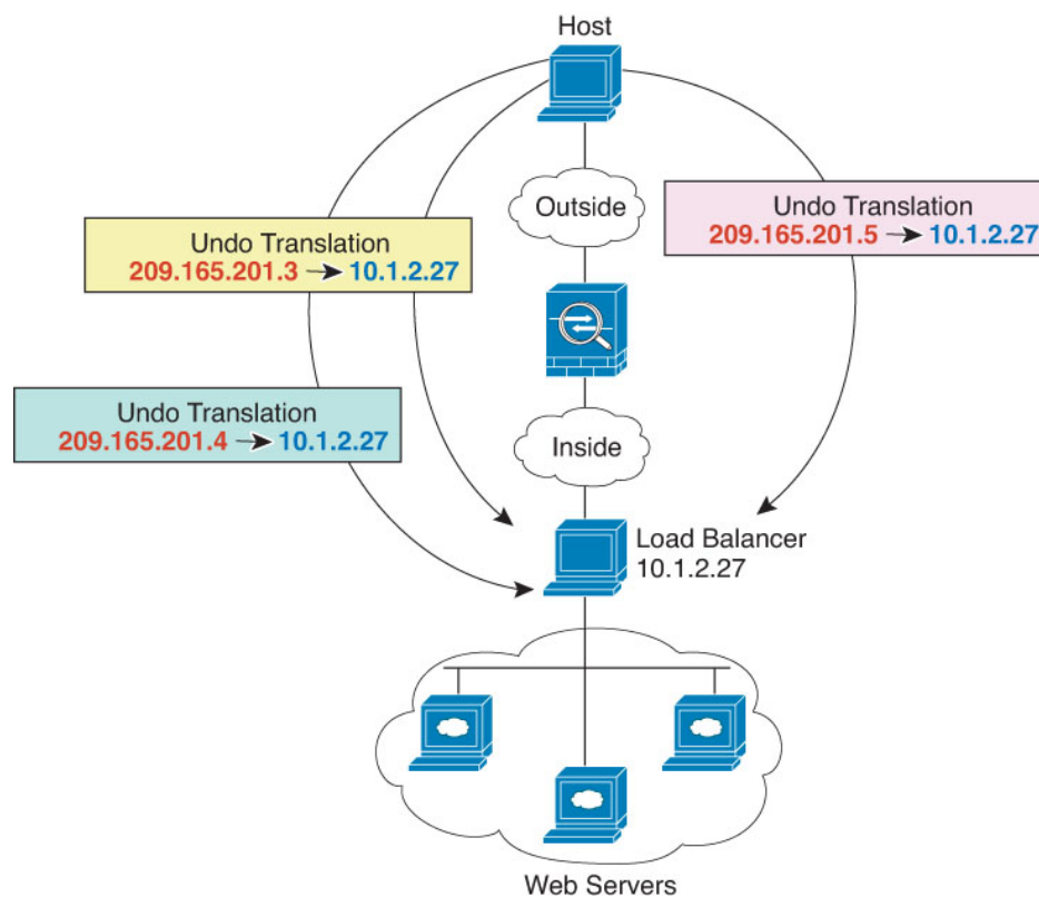
图 16: 内部负载均衡器的一对多静态 NAT
