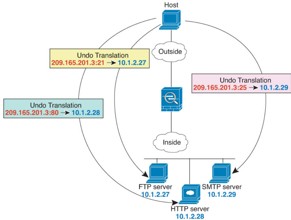
图 17: 支持端口转换的静态 NAT
