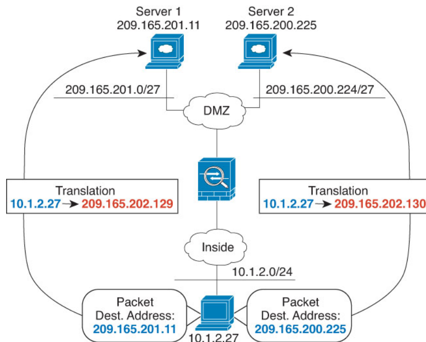
图 18: 具有不同目标地址的手动 NAT
