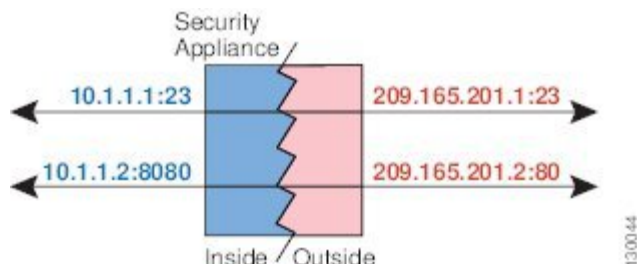
图 8: 支持端口转换的典型静态 NAT 场景
