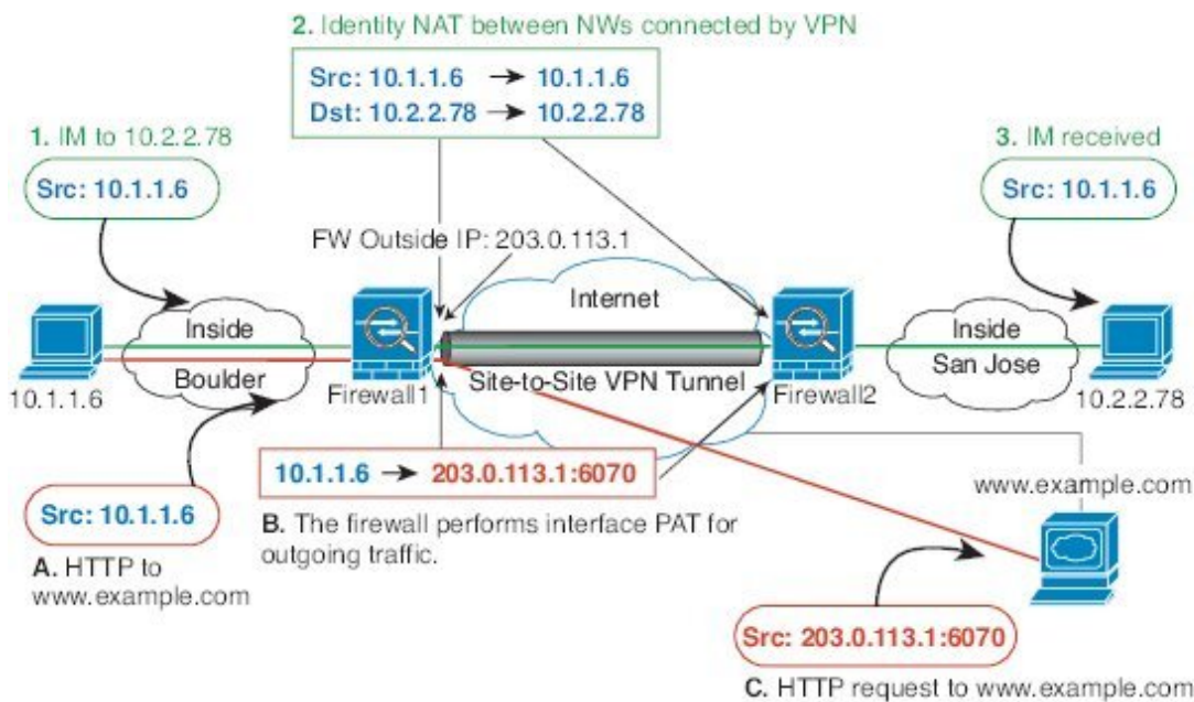
图 20: 用于站点间 VPN 的接口 PAT 和身份 NAT
