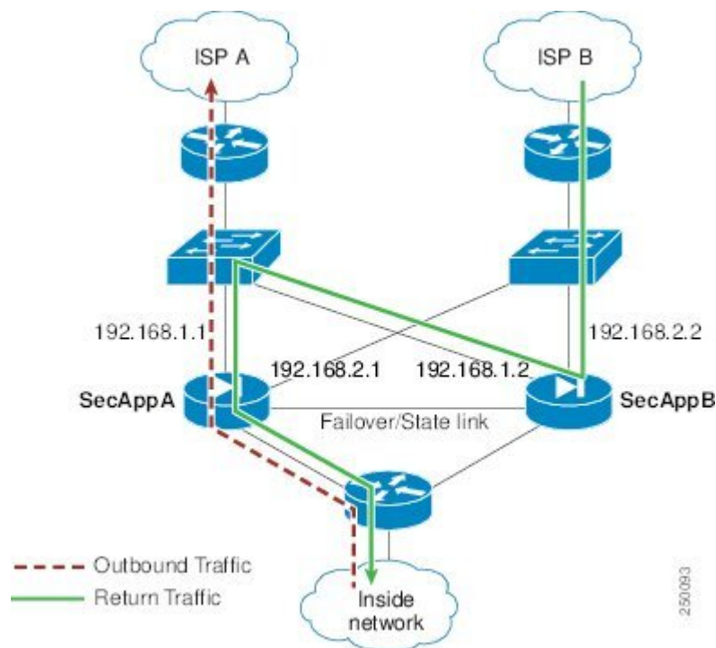
图 6: ASR 示例
