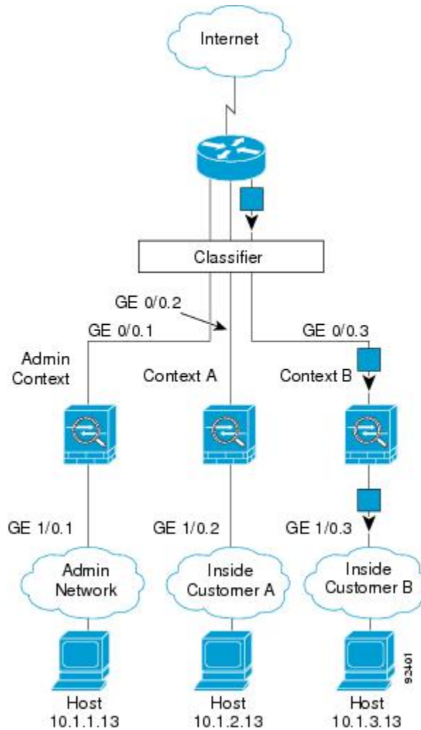
图 46: 透明防火墙情景
