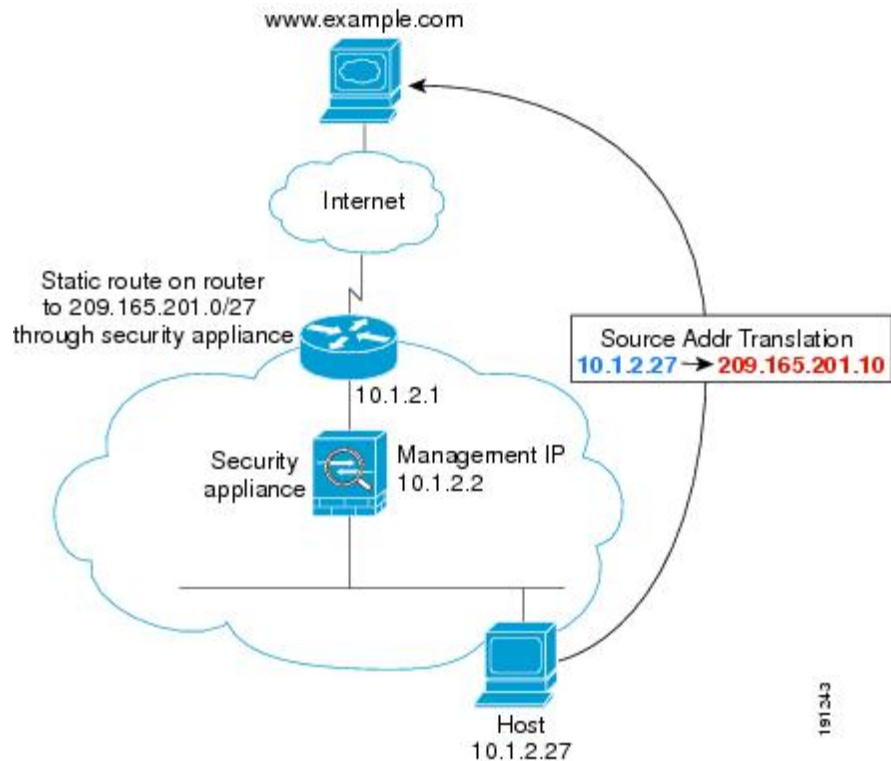
图 41: 使用 NAT 从内部到外部
