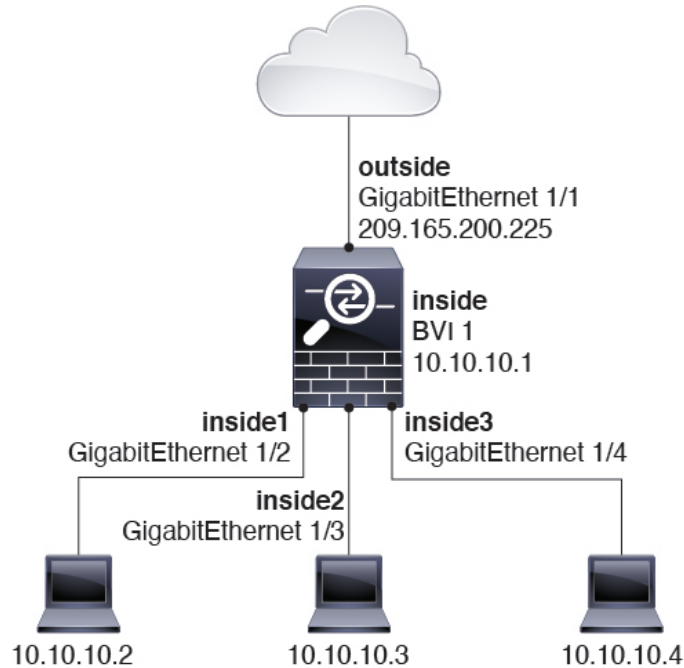
图 32: 具有内部网桥组和外部路由接口的路由防火墙网络
