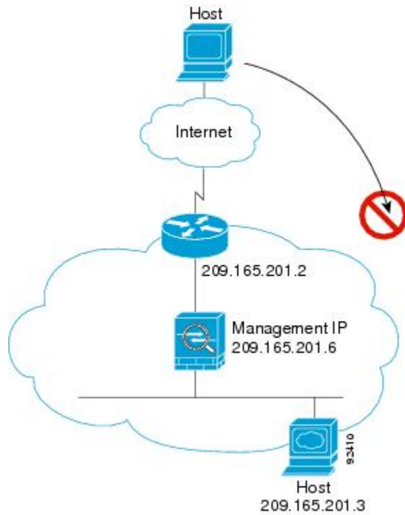
图 43: 从外部到内部
