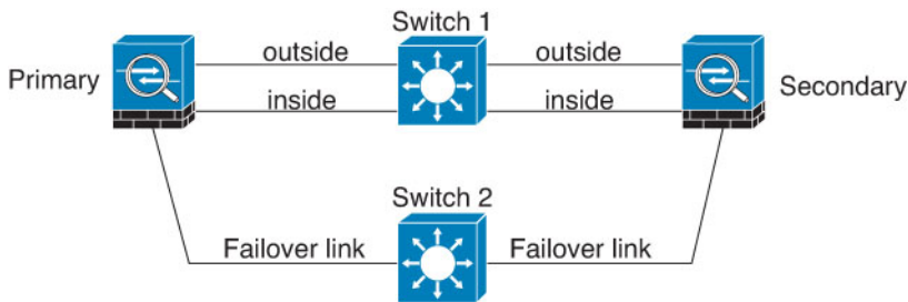
图 53: 使用其他交换机连接
