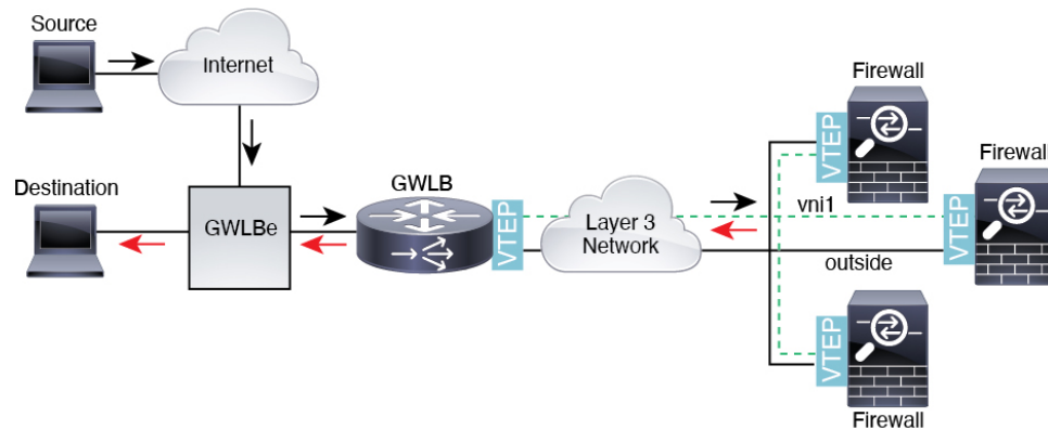
图 74: Geneve 单臂代理
