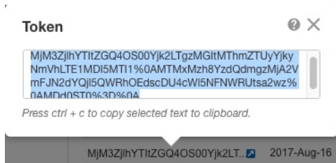
图 23: 复制令牌
