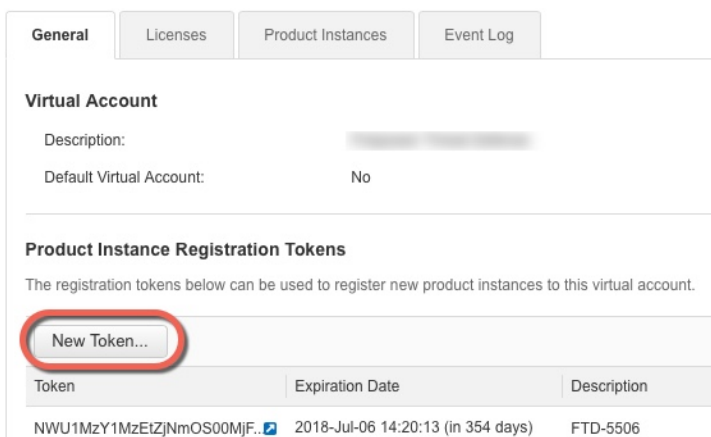
图 20: 新建令牌
