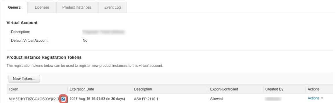
图 23: 复制令牌
