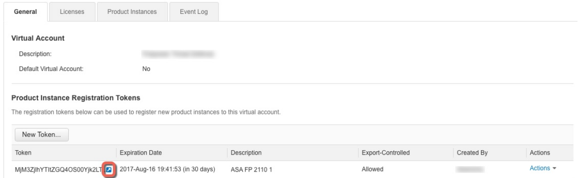
图 28: 复制令牌
