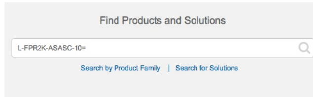
图 29: 许可证搜索
