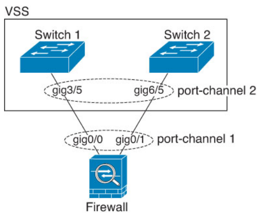
图 67: 连接至 VSS/vPC
