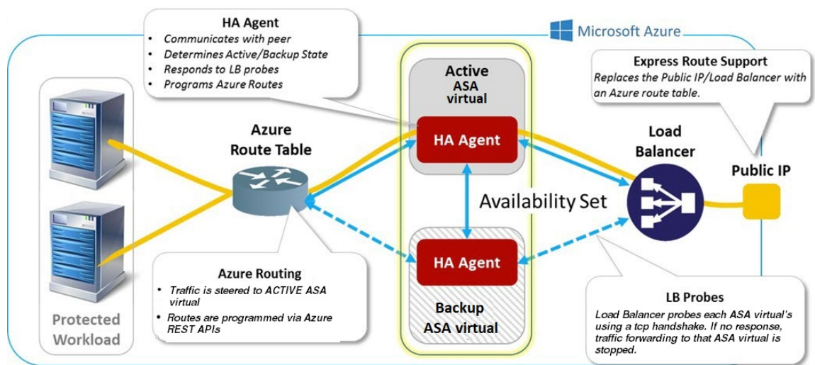
图 57: Azure 中的 ASA Virtual 高可用性部署
