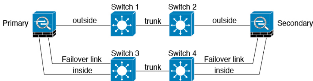
图 55: 使用安全交换机连接
