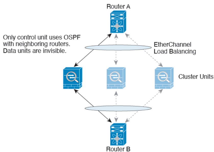
图 60: 动态路由
