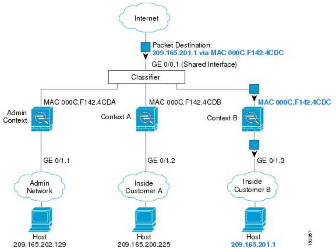
图 44: 使用 MAC 地址通过共享接口进行数据包分类
