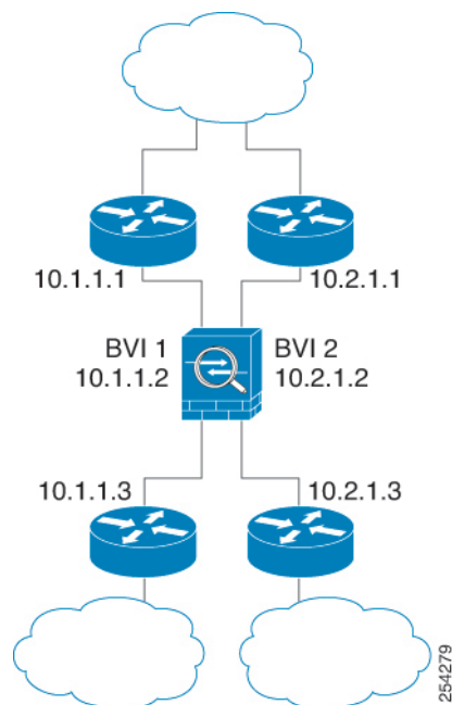
图 31: 具有两个网桥组的透明防火墙网络
