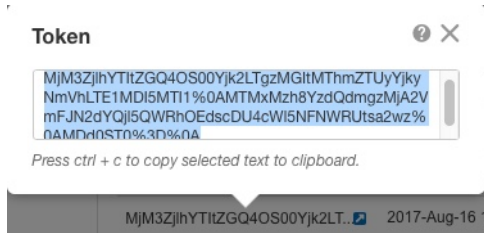
图 28: 复制令牌
