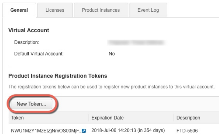
图 15: 新建令牌
