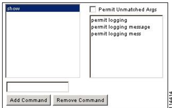
图 89: 指定缩写
