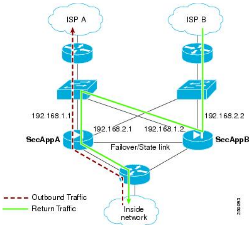
图 56: ASR 示例
