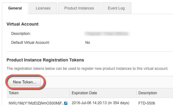
图 25: 新建令牌
