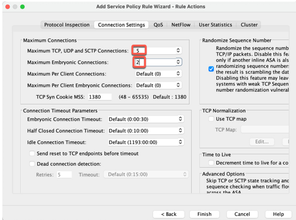
图 72: 规则操作
