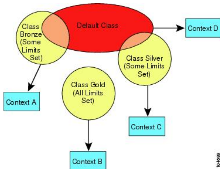
图 48: 资源类
