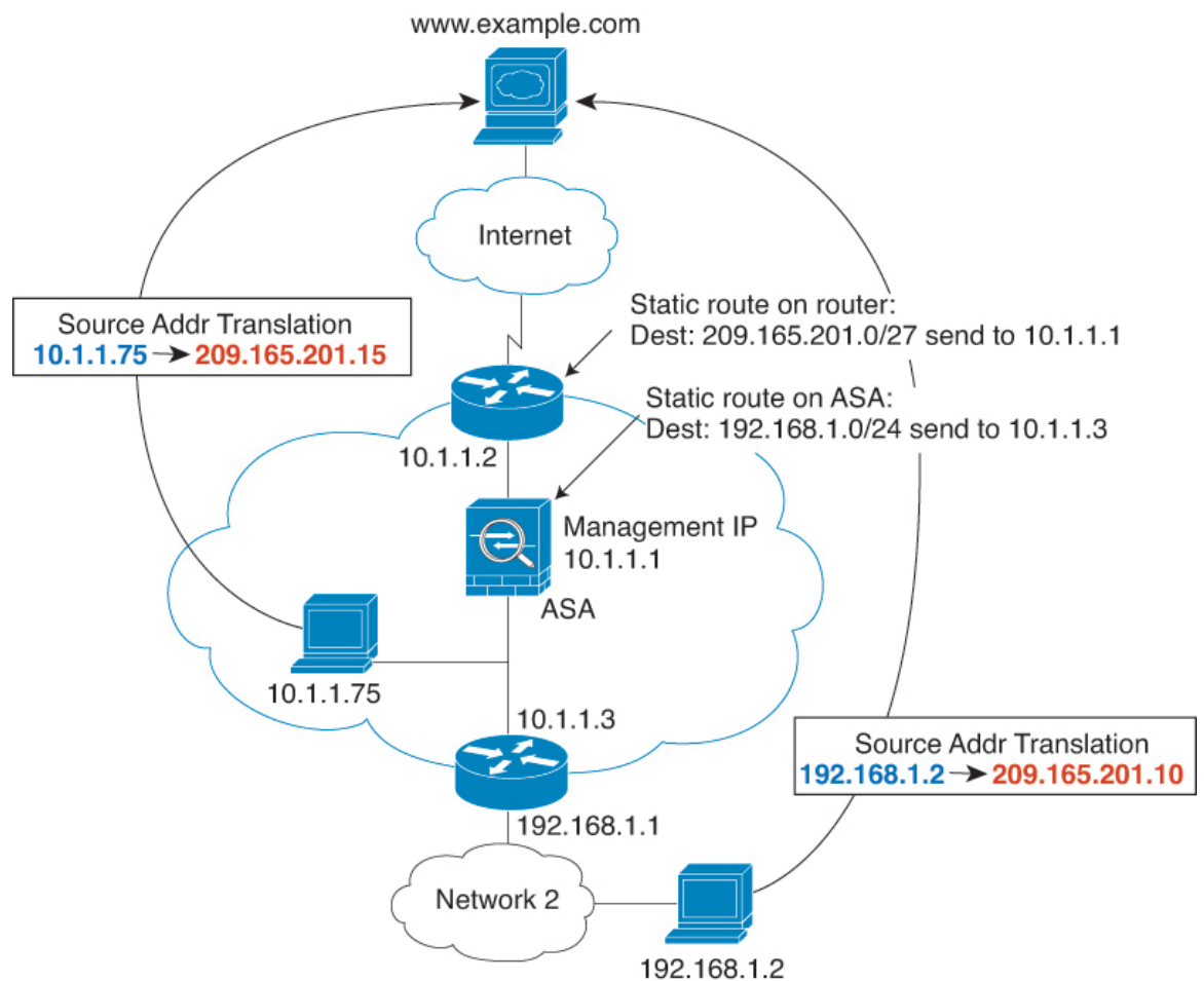
图 33: NAT 示例：网桥组中的 NAT
