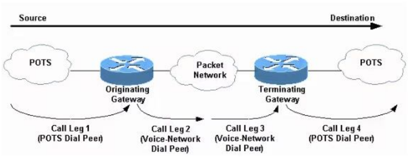
图 1.语音拨号对端/呼叫段收费绕路方案
