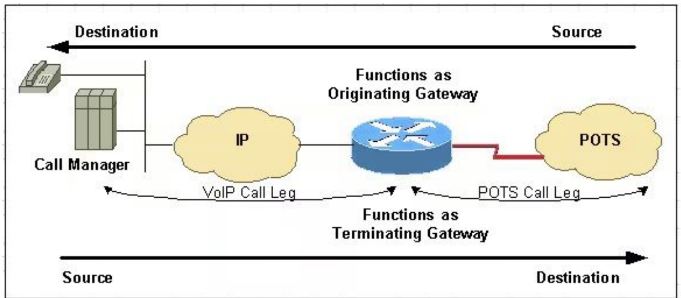
图 2.语音拨号对端/呼叫段：使用IOS网关方案的呼叫管理器系统
