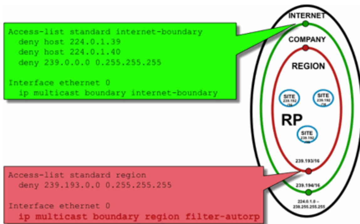
图12:自动RP过滤器/范围
