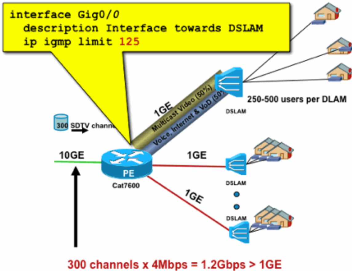
图20:使用每个接口的IGMP限制；Agg-DSLAM链路上的准入控制
