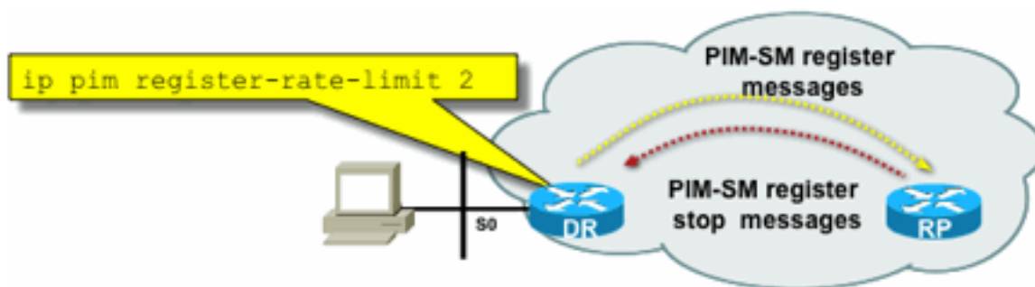
图8:PIM-SM寄存器隧道控制
