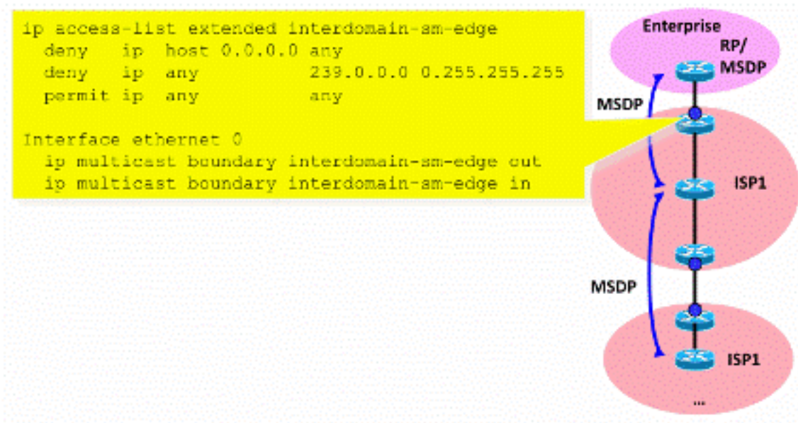
图13:域间(*,G)过滤器
