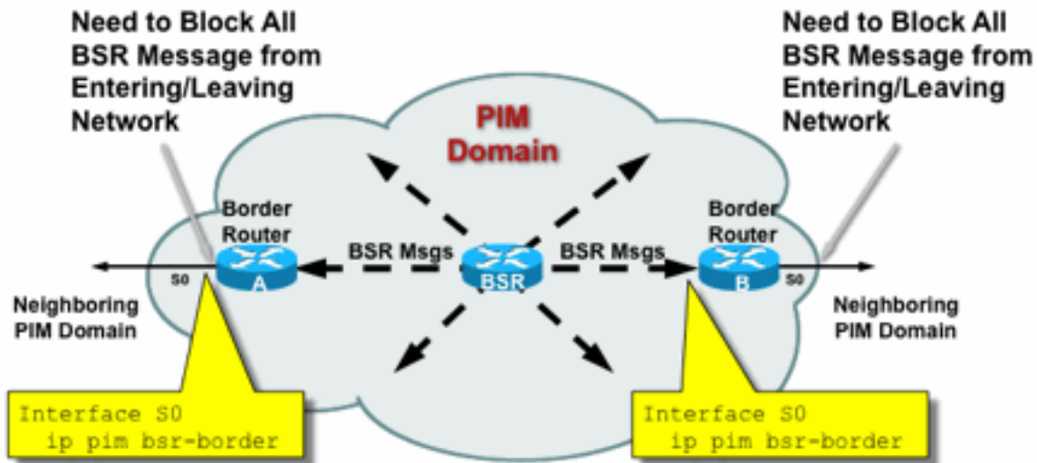
图11:BSR边界
