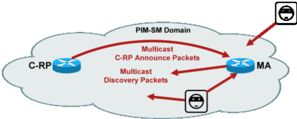
2_AutoRP_packets
