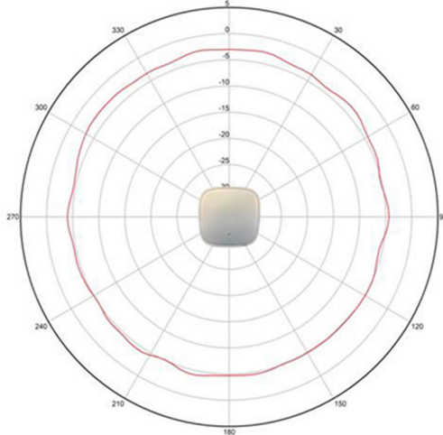
5 GHz 方位角
