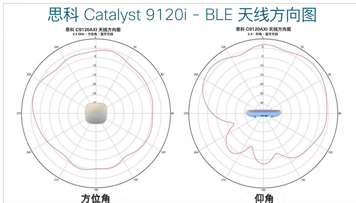
图 1. 天线辐射方向图
