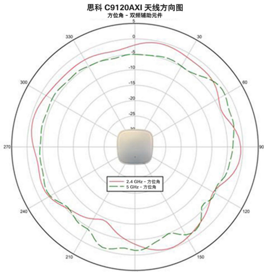
方位角
