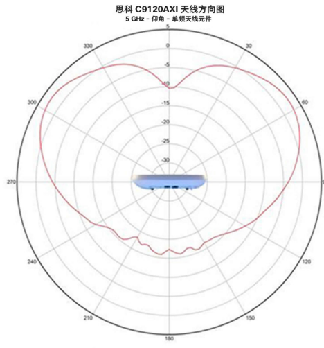
5 GHz 仰角
