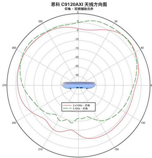
仰角
