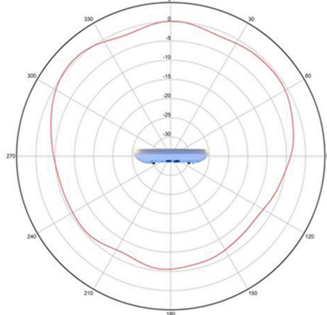
2.4 GHz 仰角
