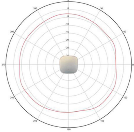
2.4 GHz 方位角
