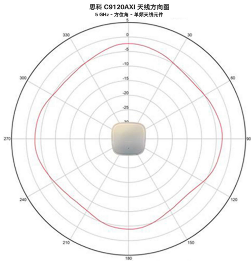
5 GHz 方位角
