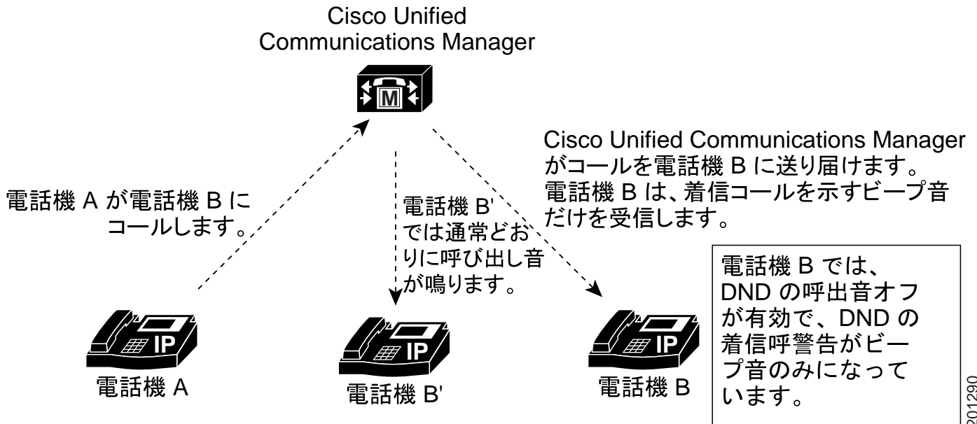
図 20-2 シェアドラインで DND の [呼出音オフ (Ringer Off)] が有効になっている場合の通常優先順位のコール
