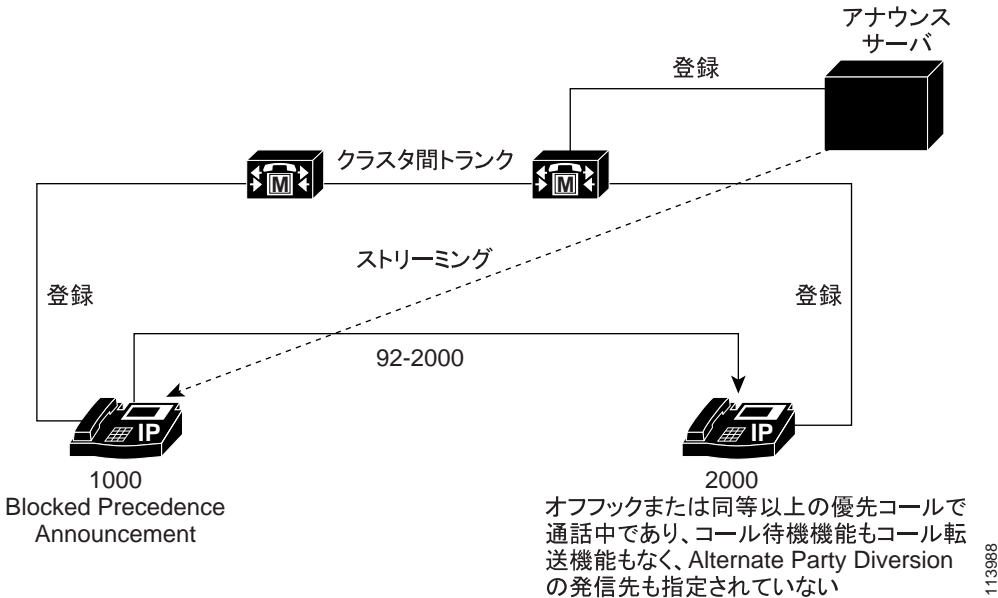
図 12-12 クラスタ間トランク上の MLPP アナウンスの例
