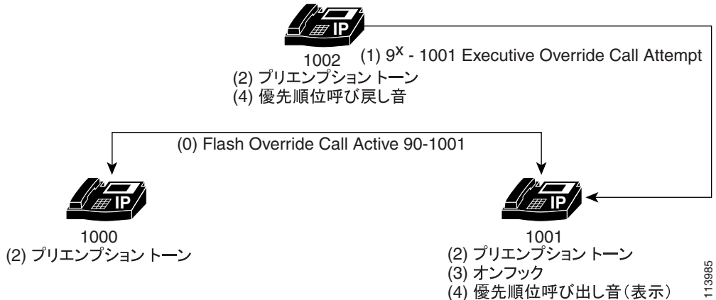
図 12-5 ユーザ アクセス プリエンプションの例
