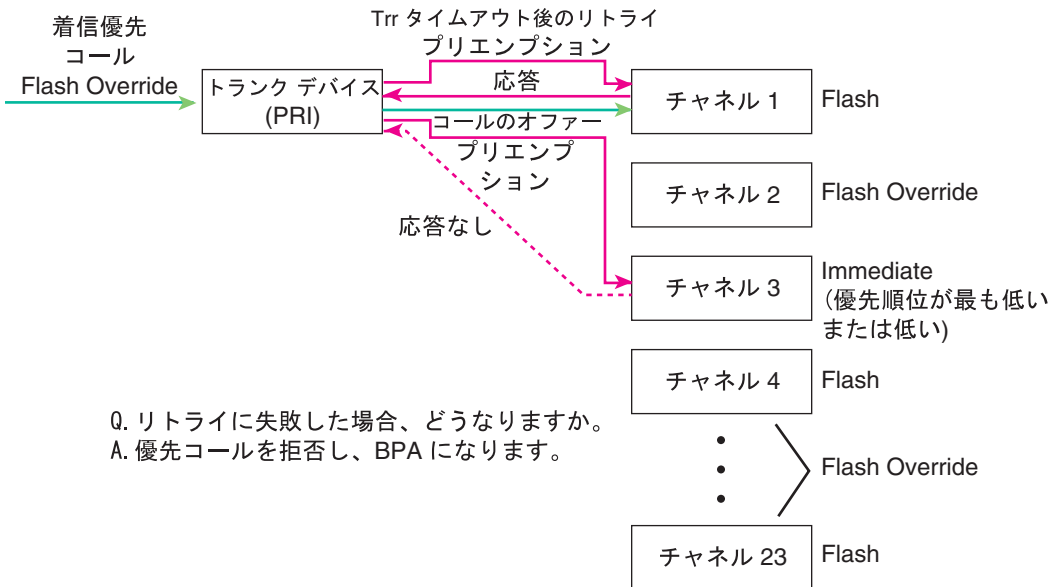
図 12-7 リトライ タイマー Trr のある共通ネットワーク ファシリティ プリエンプション
