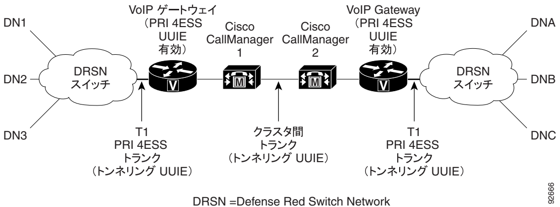
図 12-16 PRI 4ESS インターフェイスおよびクラスタ間トランクを経由する優先コール
