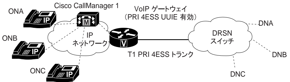
図 12-15 Cisco CallManager クラスタ内で PRI 4ESS インターフェイスを経由する優先コール
