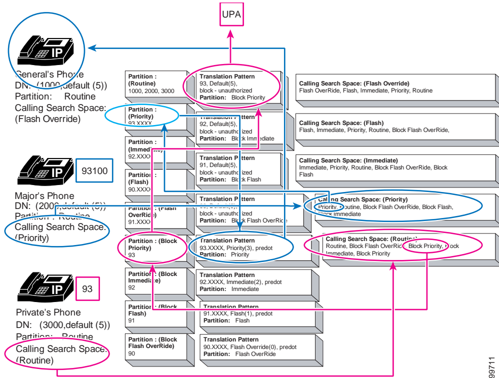
図 12-13 優先順位パターン用の MLPP 番号計画アクセス制御の例
