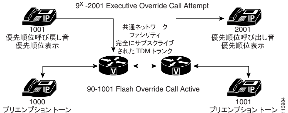
図 12-6 共通ネットワーク ファシリティ プリエンプションの例
