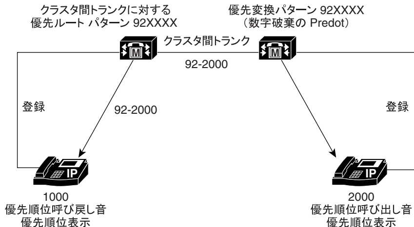
図 12-3 クラスタ間トランクの間での優先コールの設定例
