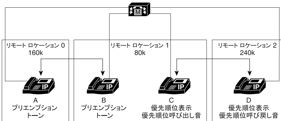
図 12-8 別のデバイスにおけるロケーションベースのプリエンブション
