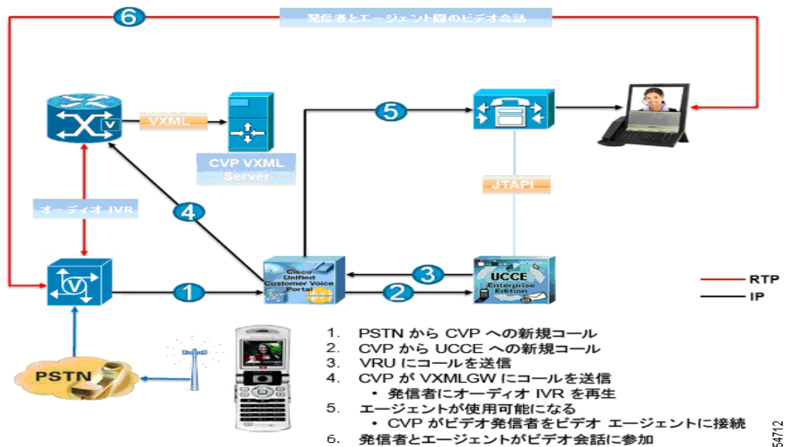
図 7-1 Cisco Integrated 3G-H324M ビデオ ゲートウェイ トポロジとコール フロー
