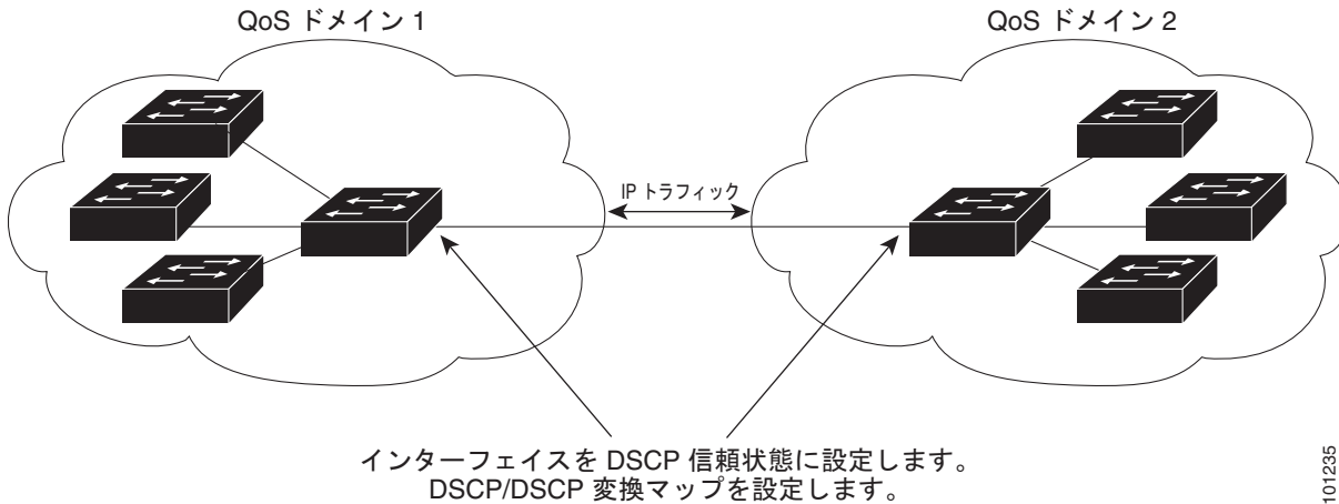
図 35-12 別の QoS ドメインとの境界ポートの DSCP 信頼状態 ポート上に DSCP trusted ステートを設定して、DSCP/DSCP 変換マップを変更するには、特権 EXEC
