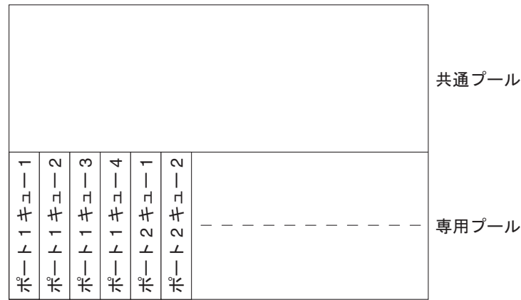
図 35-10 出力キューのバッファ割り当て
