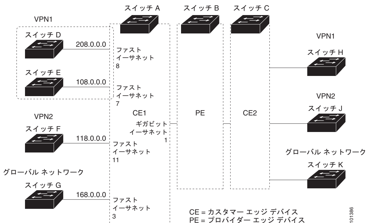
図 41-7 Multi-VRF CE の設定例
