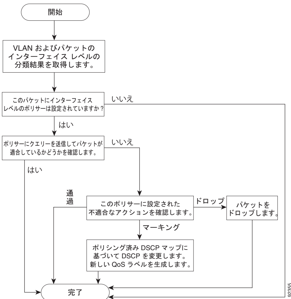
図 39-5 SVI のポリシー およびマーキング フローチャート
