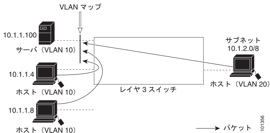
図 38-5 他 VLAN 上のサーバへのアクセス拒否
