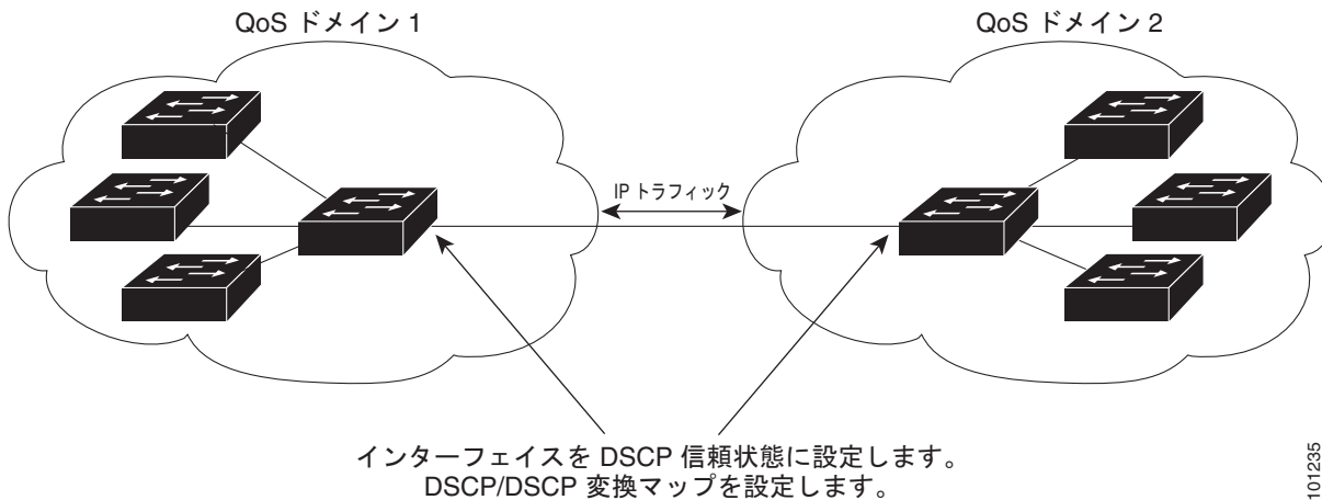
図 39-13 別の QoS ドメインとの境界ポートの DSCP 信頼状態
