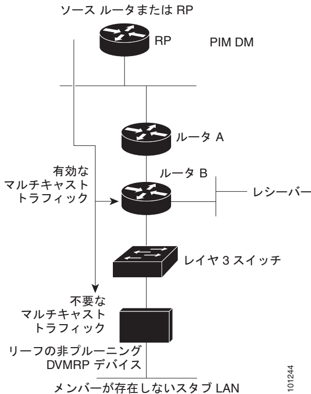
図 50-8 リーフの非プルーニング DVMRP ネイバー
