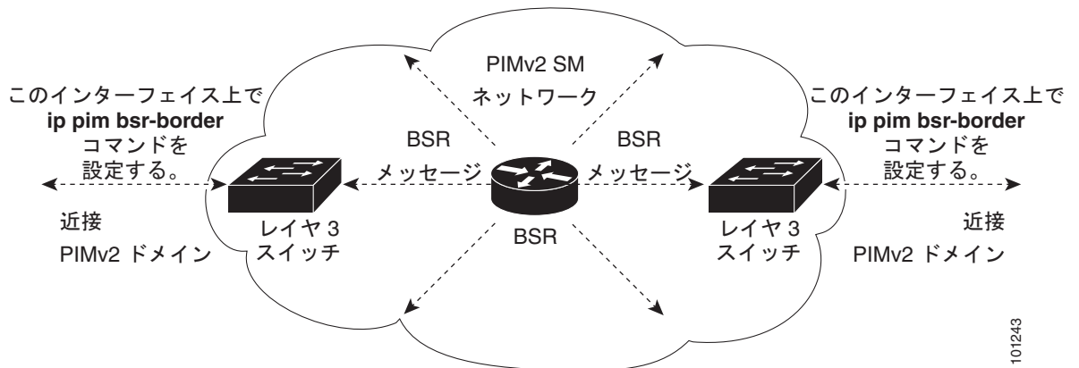
図 50-5 PIMv2 BSR メッセージの抑制
