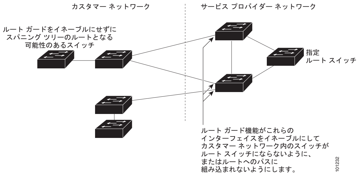
図 23-8 サービス プロバイダー ネットワークのルート ガード
