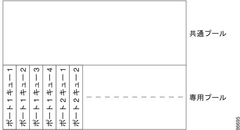
図 39-10 出力キューのバッファ割り当て
