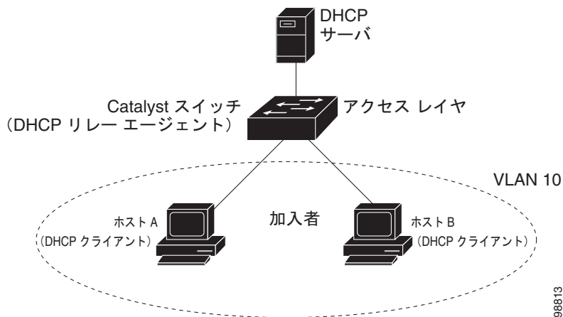
図 26-1 メトロポリタンイーサネットネットワークにおける DHCP リレー エージェント
