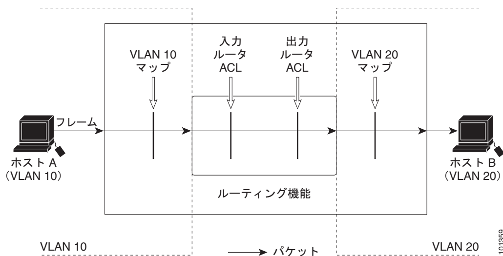
図 38-8 ルーテッド パケットへの ACL の適用
