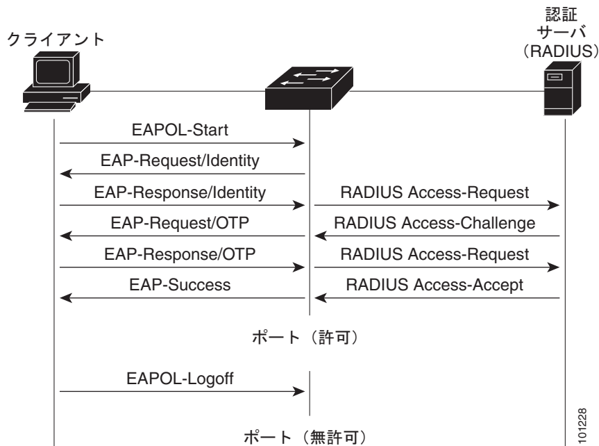
図 12-3 メッセージ交換
