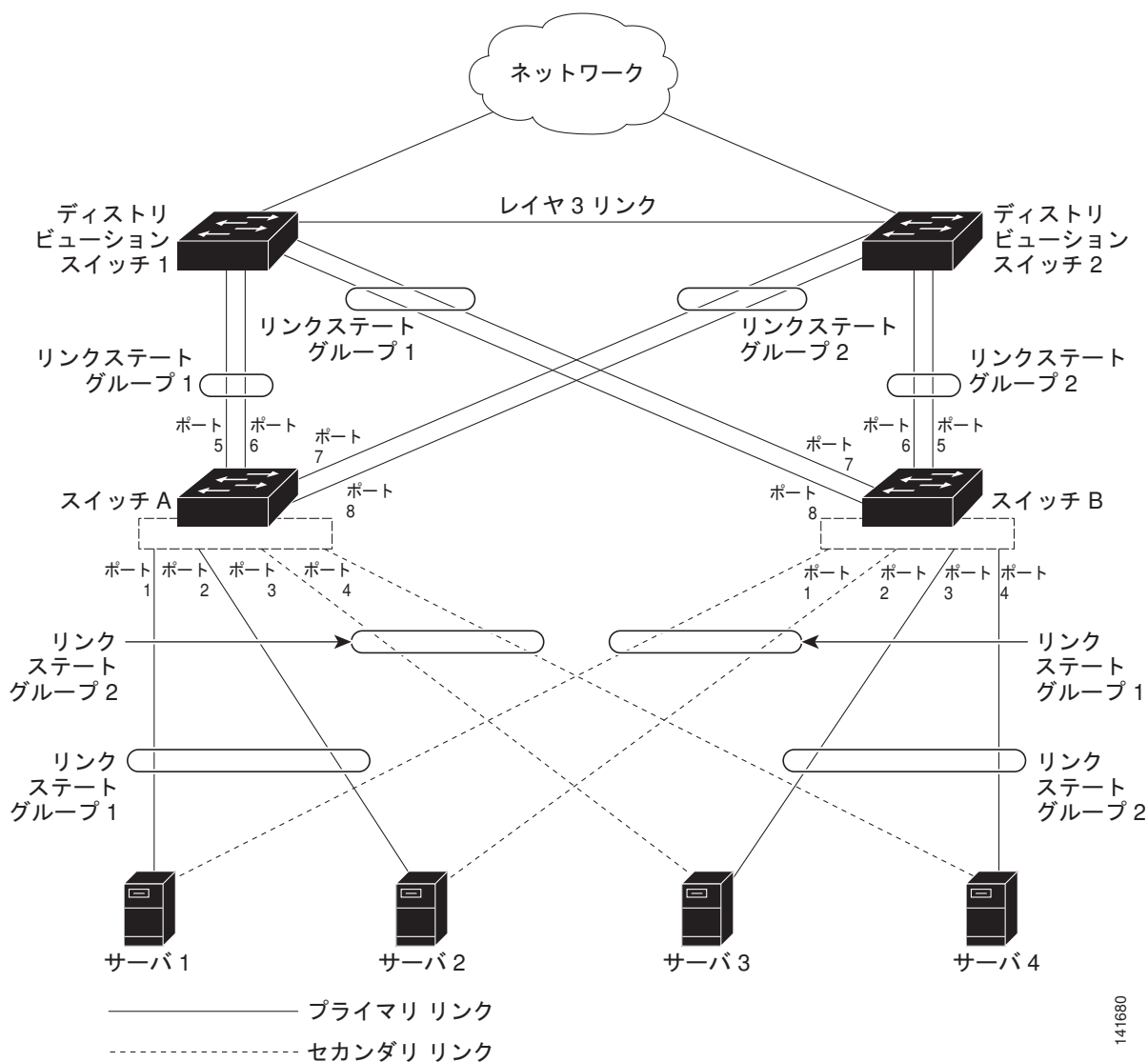
図 40-4 一般的なリンクステートトラッキングの設定
