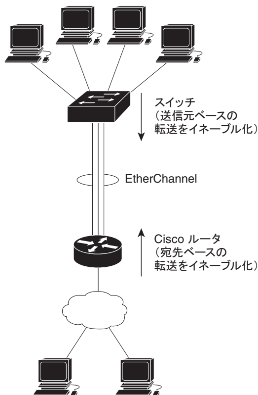
図 40-3 負荷の分散および転送方式
