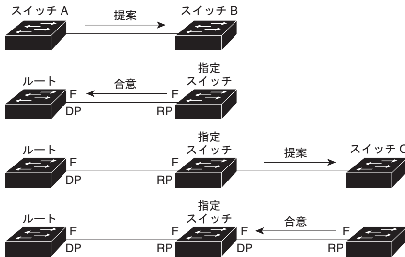
図 22-4 高速コンバージェンスの提案と合意のハンドシェイク
