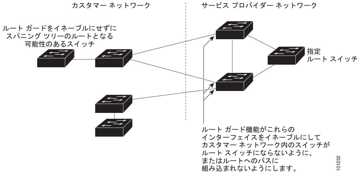
図 21-8 サービス プロバイダー ネットワークのルート ガード
