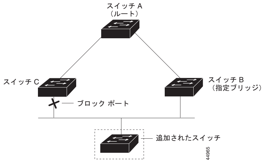
図 21-7 メディア共有型トポロジにおけるスイッチの追加
