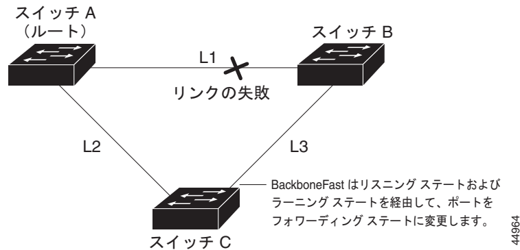
図 21-6 間接リンク障害発生後の BackboneFast の例
