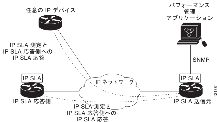
図 45-1 Cisco IOS IP SLA 動作
