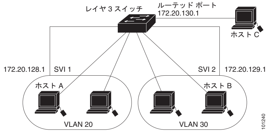
図 50-1 フォールバックブリッジネットワークの例
