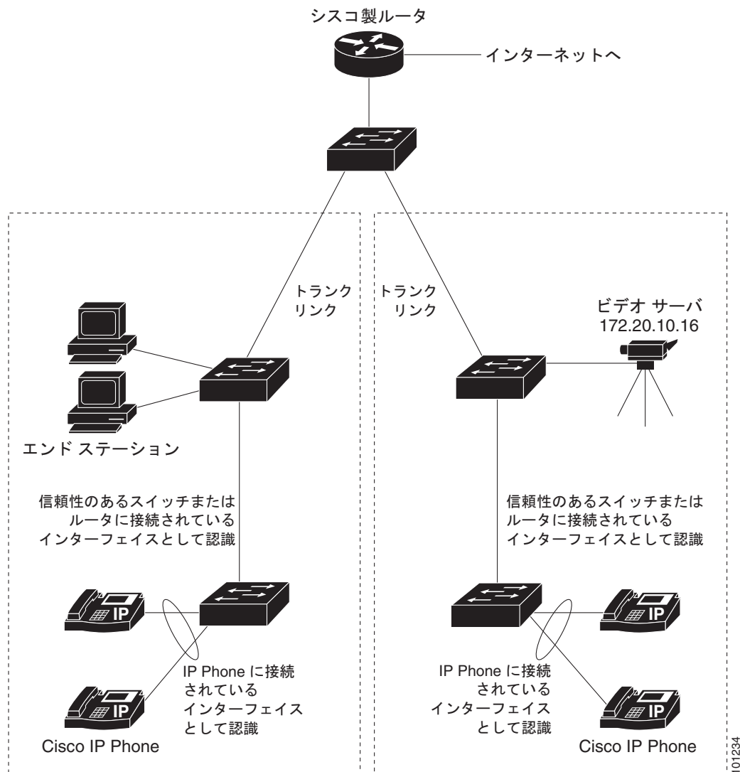
図 37-11 ネットワークでの自動 QoS の設定例
