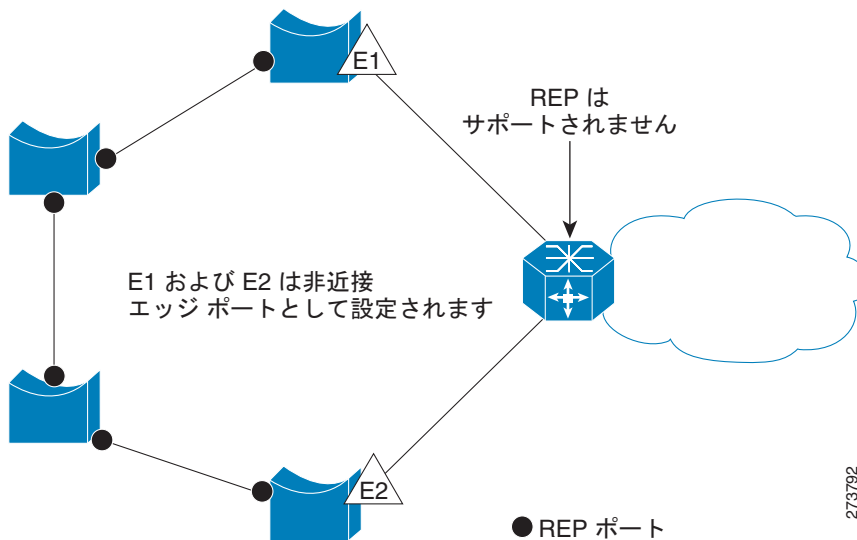
図 22-3 非ネイバー エッジ ポート
