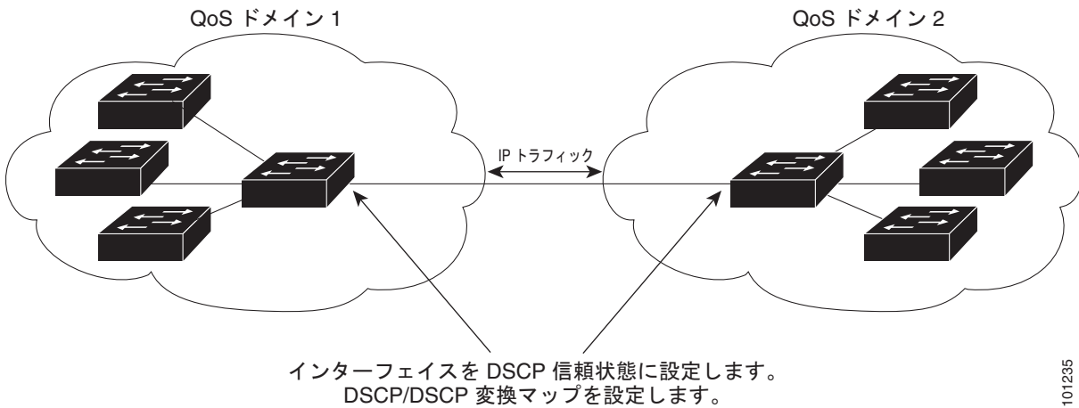
図 37-13 別の QoS ドメインとの境界ポートの DSCP 信頼状態
