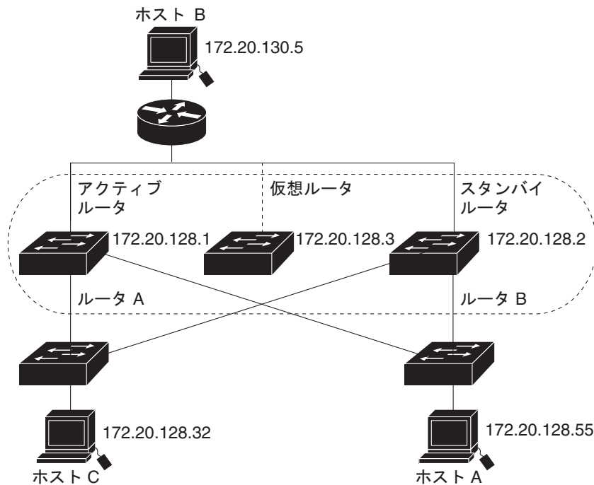
図 44-1 HSRP の一般的な構成
