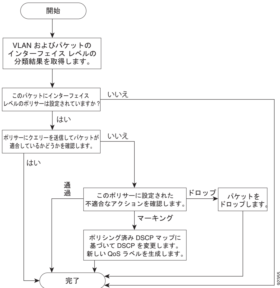
図 37-5 SVI のポリシーおよびマーキング フローチャート
