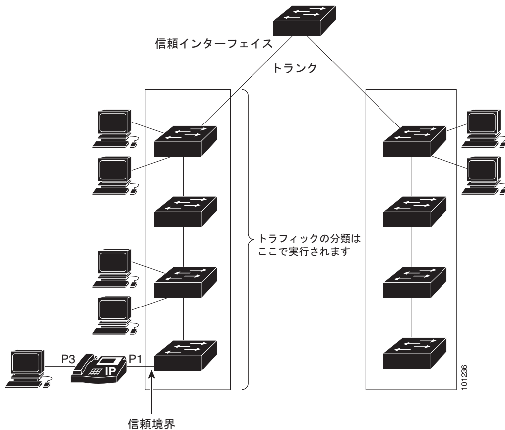
図 37-12 QoS ドメイン内のポートの信頼状態
