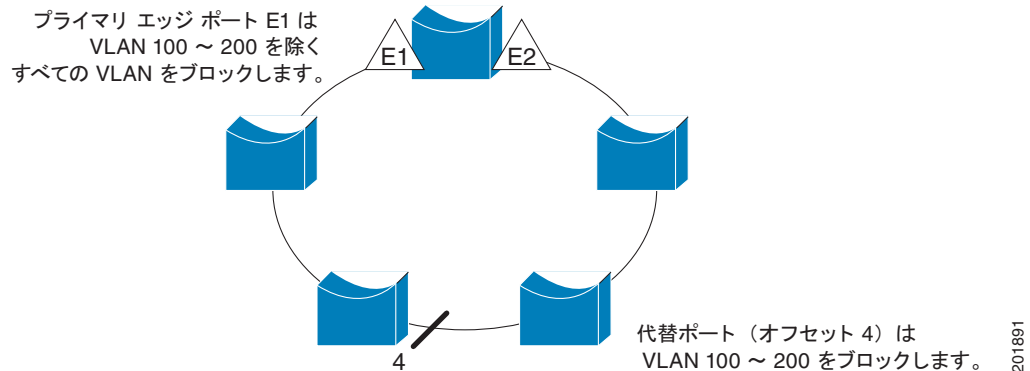
図 22-5 VLAN ブロッキングの例
