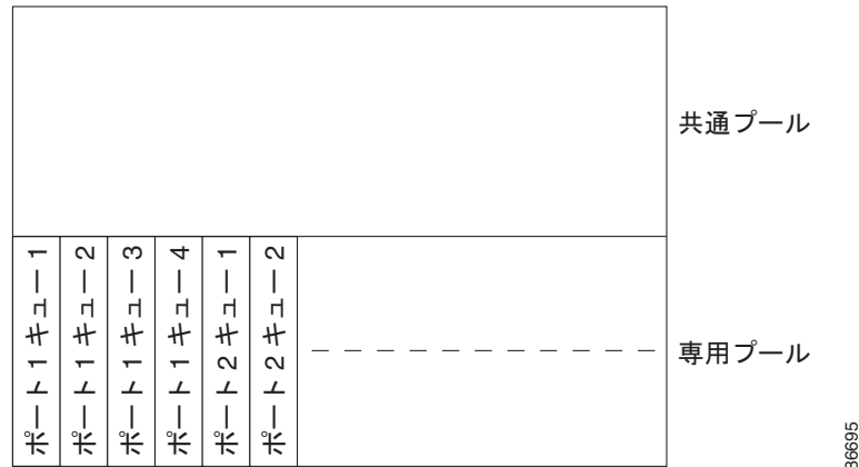
図 37-10 出力キューのバッファ割り当て
