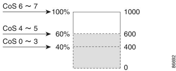
図 37-7 WTD およびキューの動作
