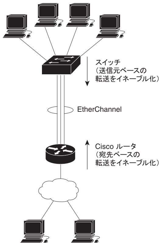
図 38-3 負荷の分散および転送方式
