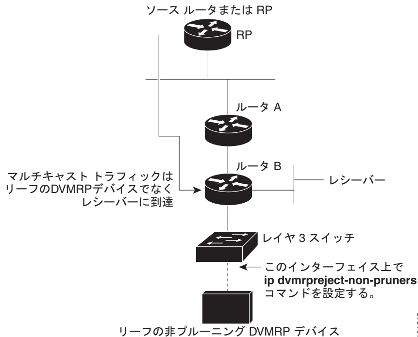
図 48-9 ルータが非ブルーニング DVMRP ネイバーを拒否する例
