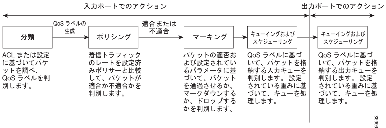
図 37-2 QoS の基本モデル
