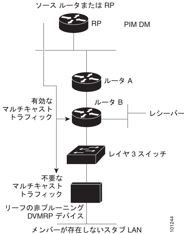
図 48-8 リーフの非プルーンング DVMRP ネイバー
