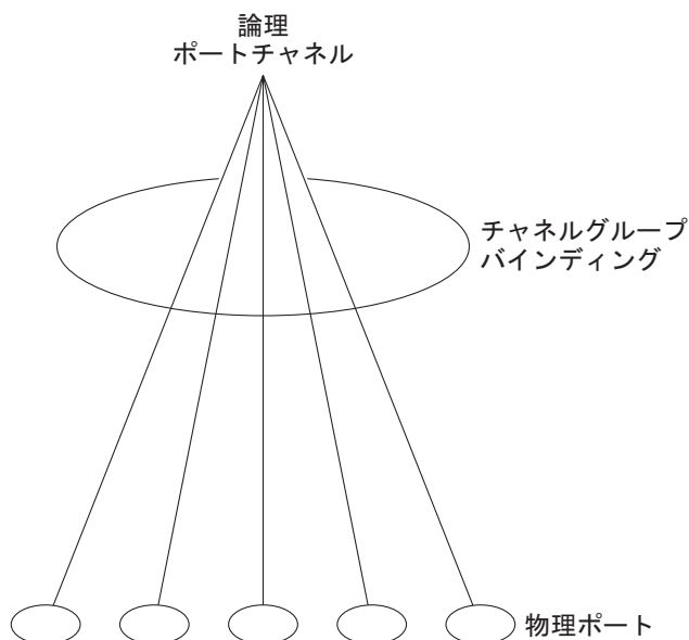
図 38-2 物理ポート、論理ポートチャネル、およびチャネル グループの関係
