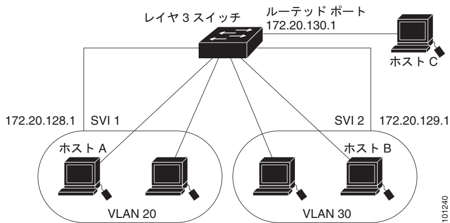
図 50-1 フォールバック ブリッジング ネットワークの例
