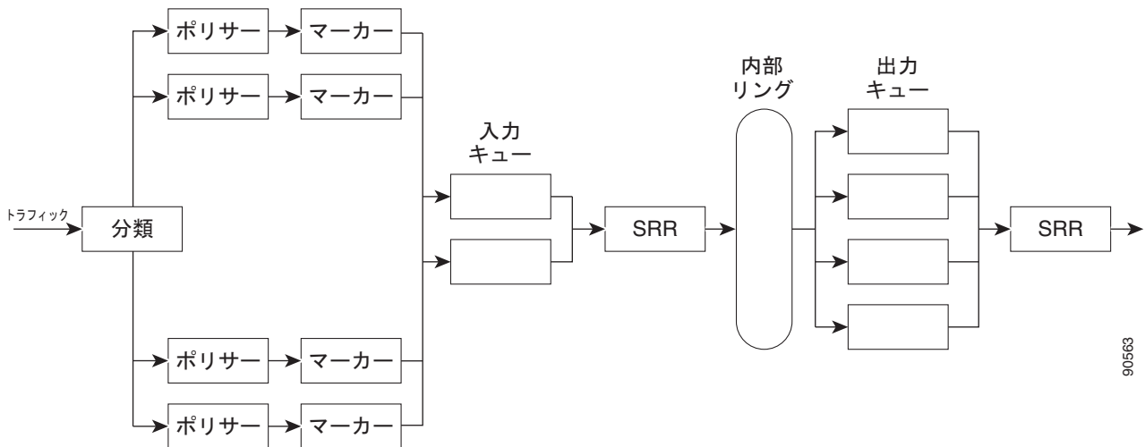
図 37-6 入力および出力キューの位置
