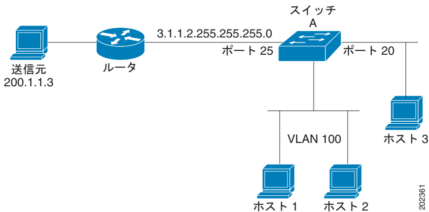
図 48-2 PIM スタブ ルータ設定
