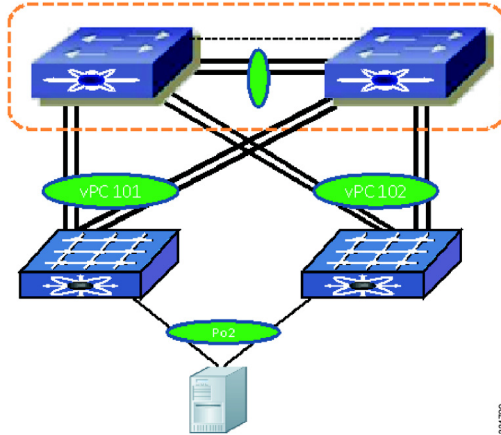
図 5-1 拡張 vPC トポロジ
