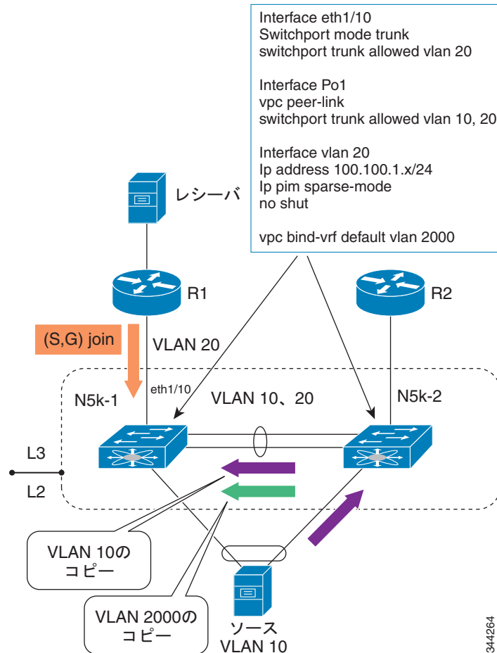
図 2-13 機能しないトポロジ：VLAN トランク ポートを使用したルータの接続
