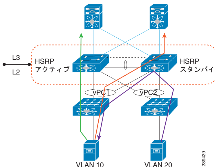
図 2-1 vPC および FHRP
