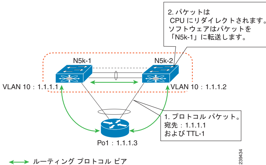
図 2-6 vPC トポロジでの制御トラフィックの転送
