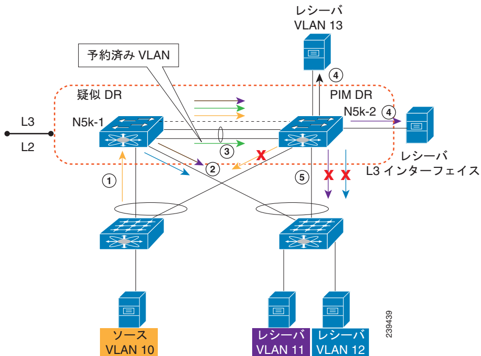
図 2-10 マルチキャスト データの転送
