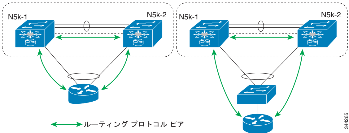
図 2-14 機能しないトポロジ : vPC 上のルーティング ピアリング
