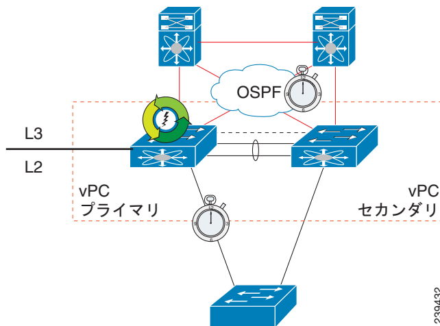
図 2-4 vPC の遅延復元
