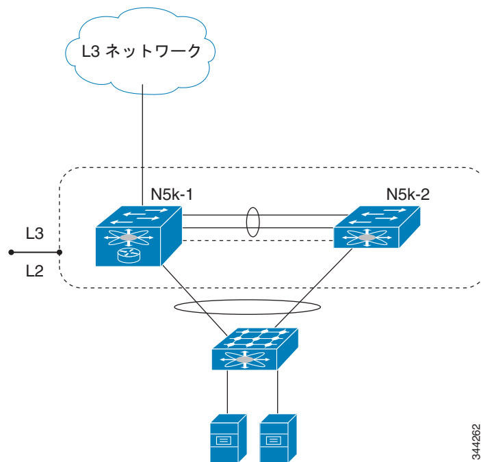
図 2-11 機能しないトポロジ：レイヤ 3 を 1 台の vPC スイッチのみでイネーブル
