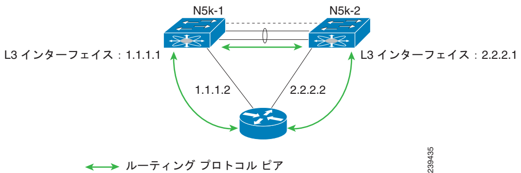
図 2-7 レイヤ 3 インターフェイスを使用したルータの vPC ドメインへの接続
