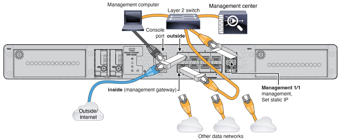
図 5: エッジ展開のケーブル配線
