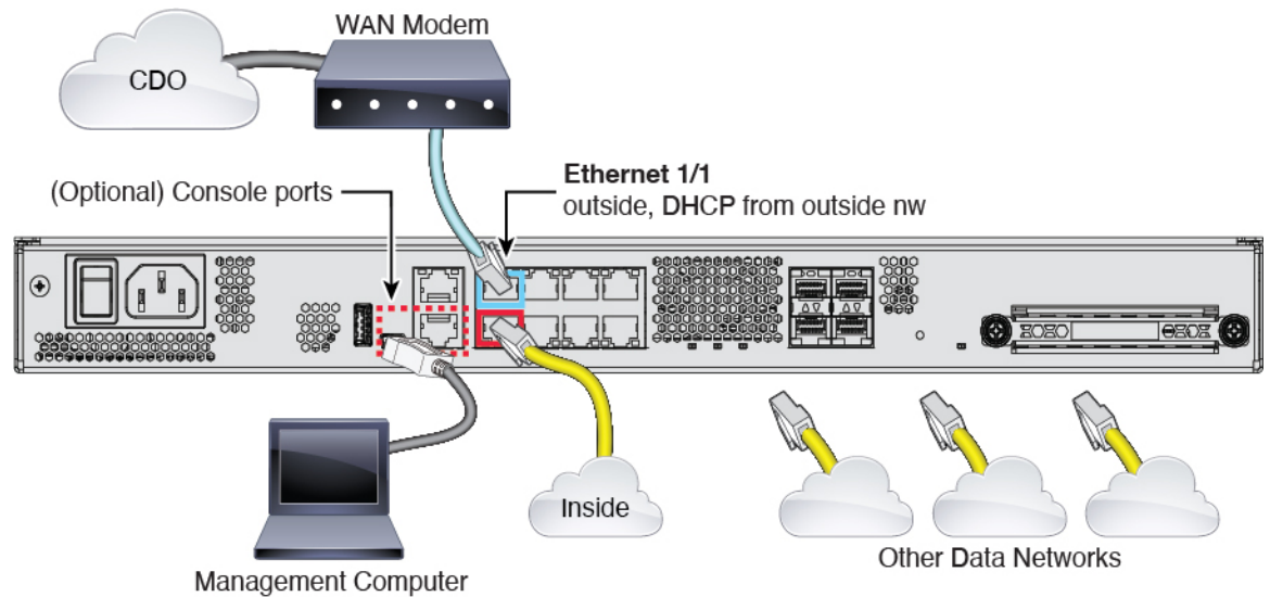
図 8: Firepower 1100 のケーブル配線
