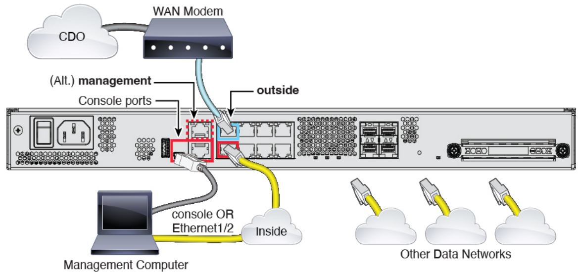
図 10: Firepower 1100 のケーブル配線
