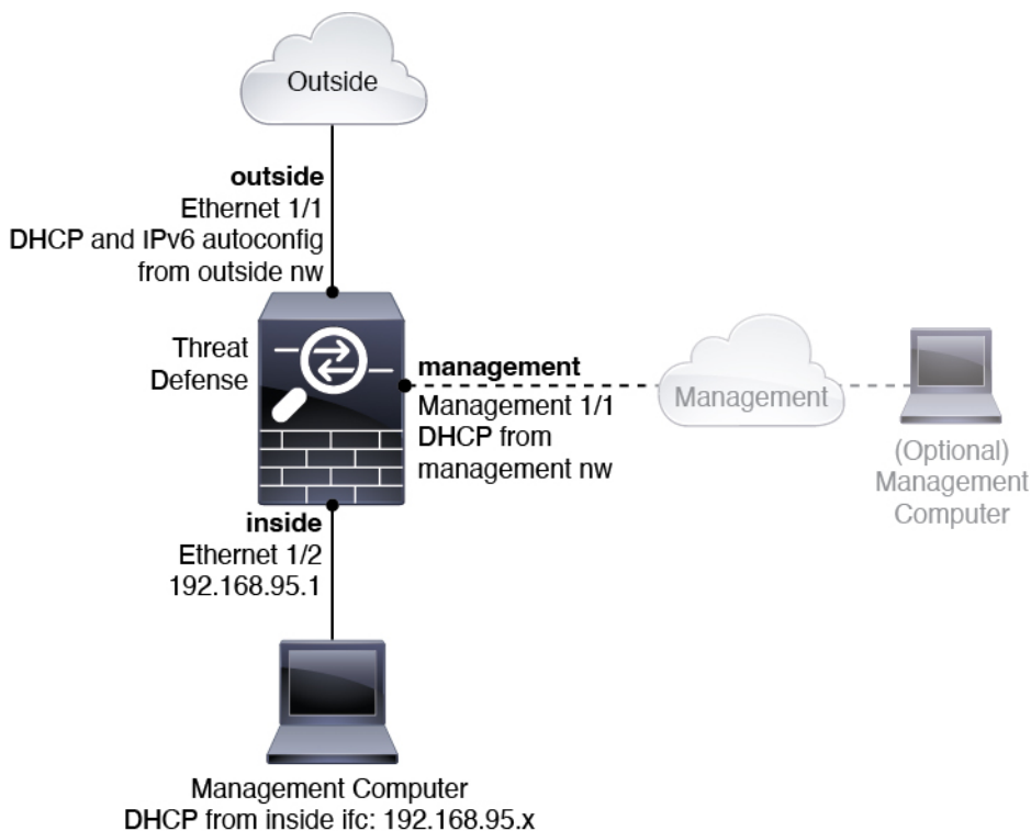
図 1: 推奨されるネットワーク配置
