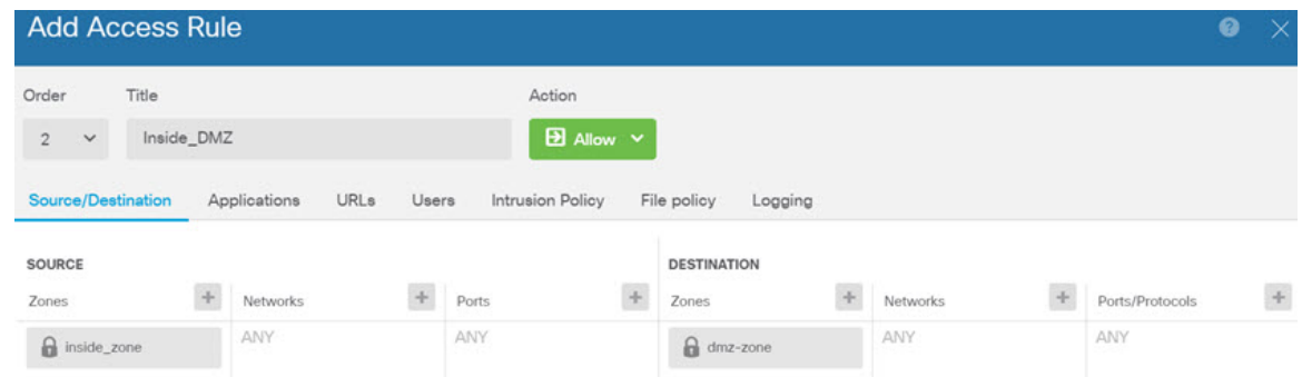
図 9: アクセスコントロールポリシー
