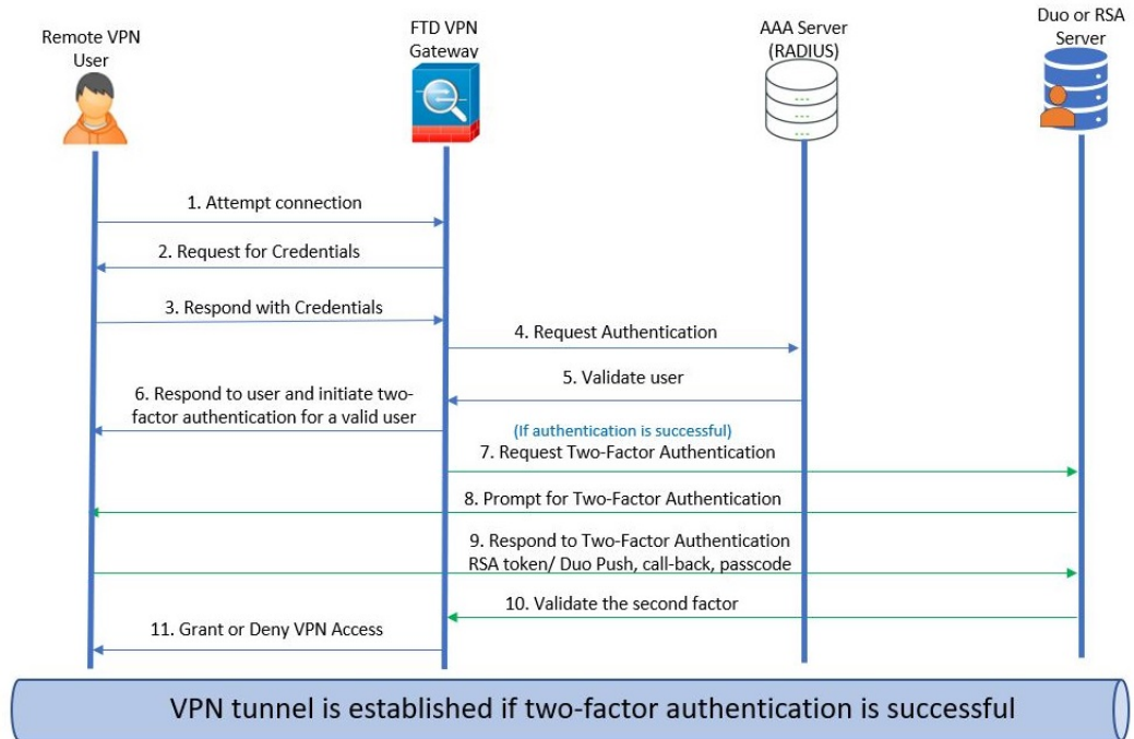
図 1: 二要素認証
