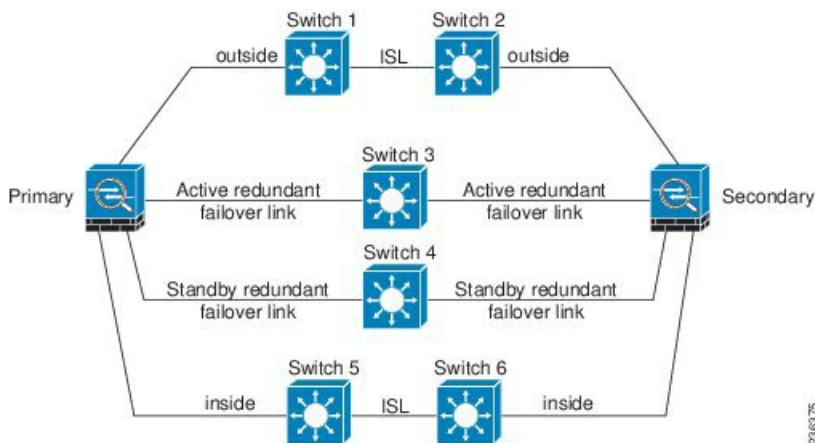
図 7: Inter-Switch Link (ISL) を使用した接続
