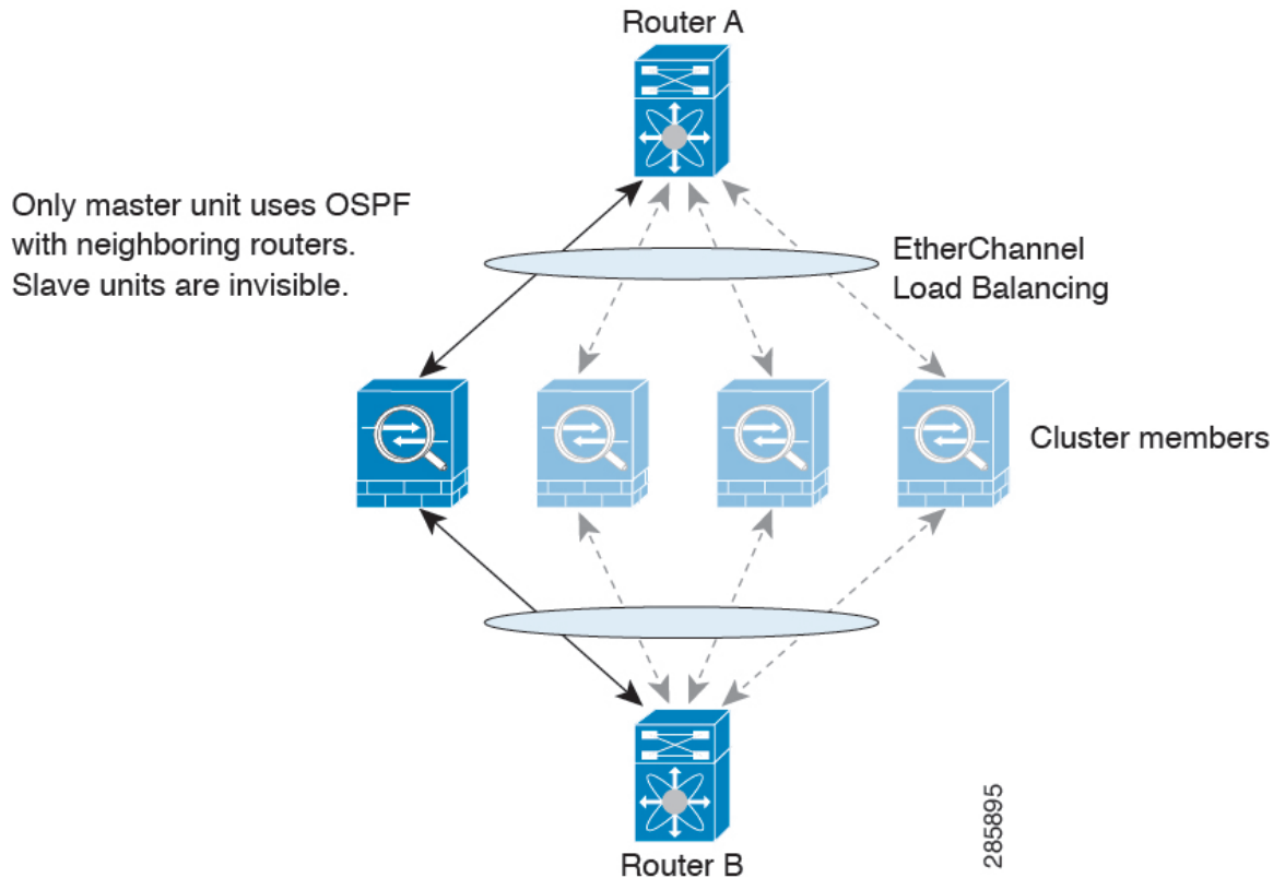
図 2: クラスタリングでのダイナミック ルーティング
