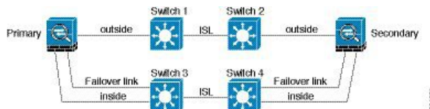
図 11: セキュアスイッチを使用した接続
