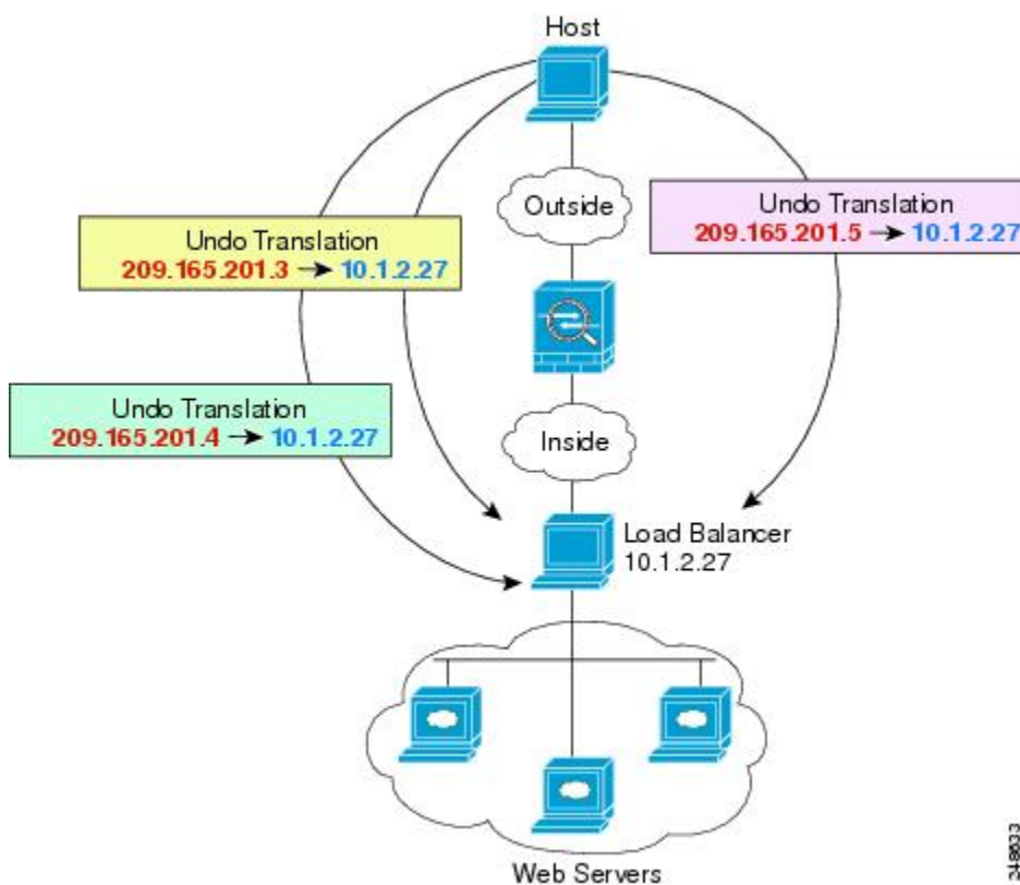
図 36: 内部ロードバランサのスタティック NAT (1対多)
