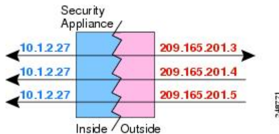
図 29: 一対多のスタティック NAT
