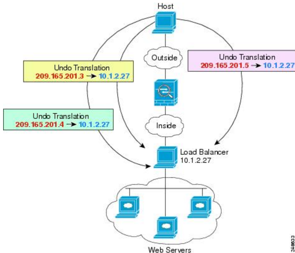
図 30: 一対多のスタティック NAT の例
