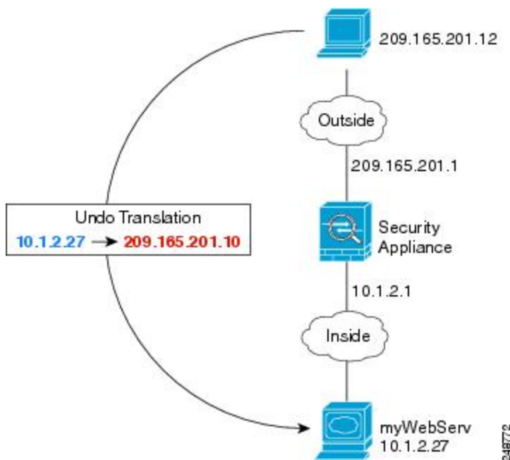
図 34: 内部 Web サーバのスタティック NAT
