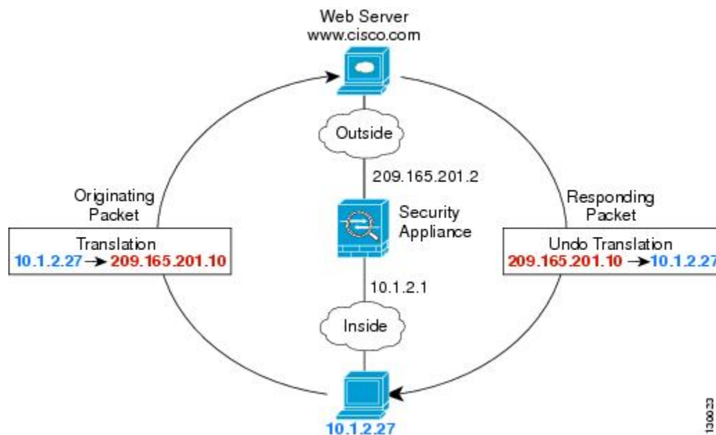
図 21: NAT の例: ルーテッドモード
