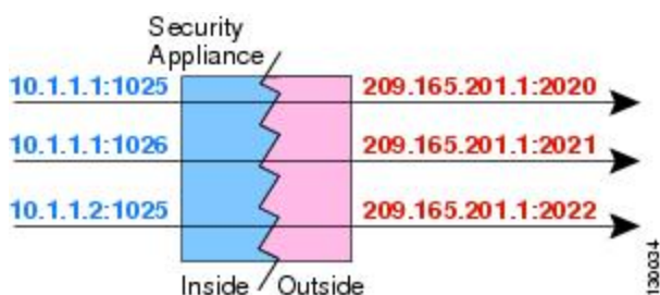
図 26: ダイナミック PAT
