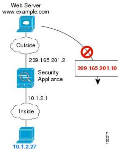
図 25: マッピングアドレスへの接続開始を試みているリモートホスト
