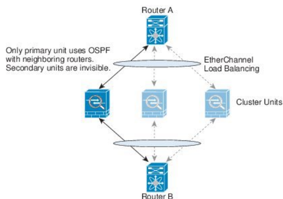
図 14: ダイナミック ルーティング
