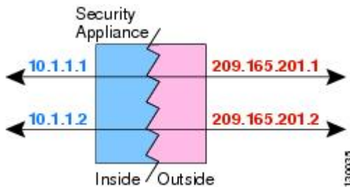
図 27:スタティック NAT
