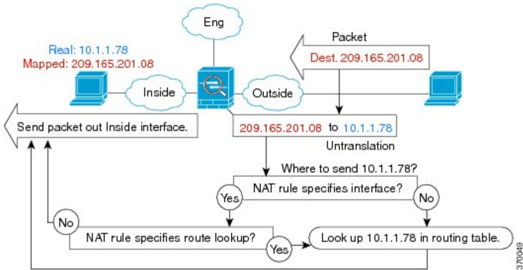
図 15: NATによるルーテッドモードでの出インターフェイスの選択
