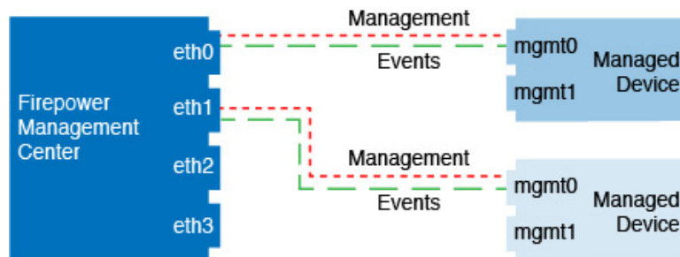
図 18: Firepower Management Center 上の複数の管理インターフェイスを使用する場合
