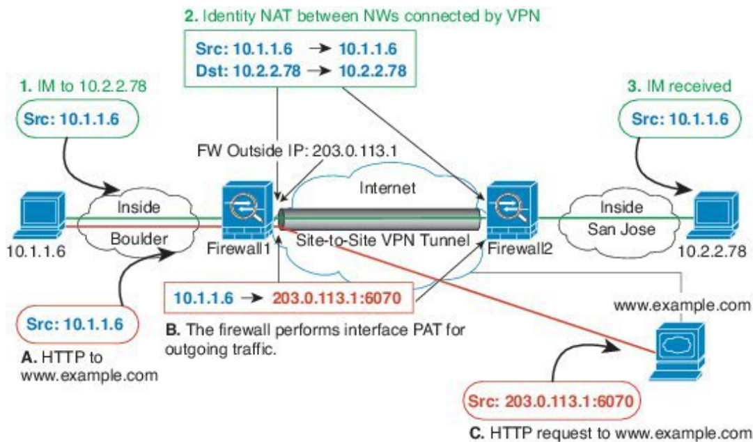
図 40: サイトツーサイト VPN のためのインターフェイス PAT およびアイデンティティ NAT
