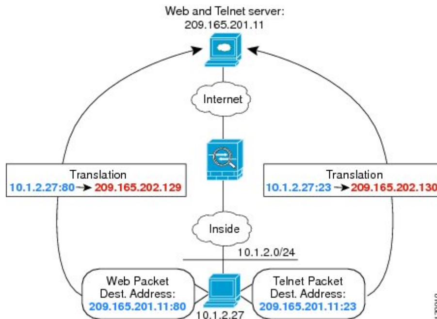
図 39:異なる宛先ポートを使用する手動 NAT
