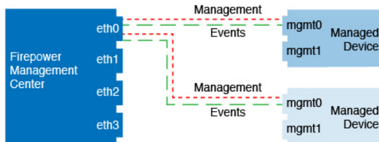
図 17: Firepower Management Center 上で単一の管理インターフェイスを使用する場合
