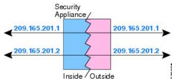
図 33: アイデンティティ NAT
