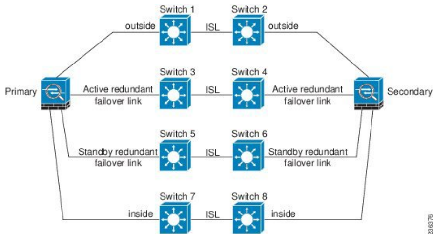
図 13: Inter-Switch Link (ISL) を使用した接続
