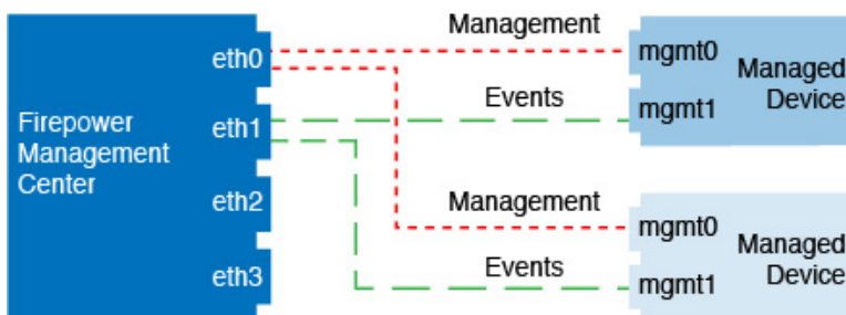
図 19: Firepower Management Center 上の個別のイベントインターフェイスと管理対象デバイスを使用する場合
