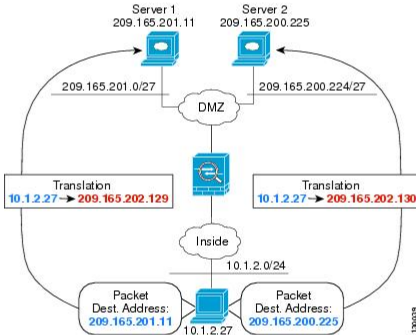
図 38:異なる宛先アドレスを使用する手動 NAT
