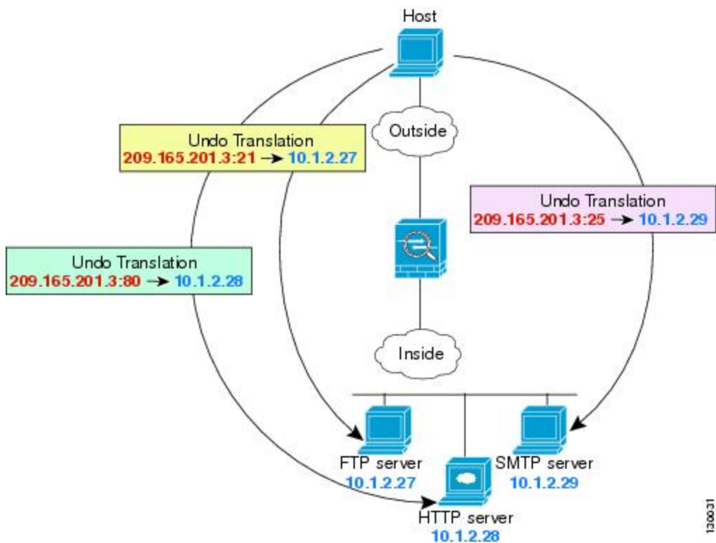
図 37: ポート変換を設定したスタティック NAT
