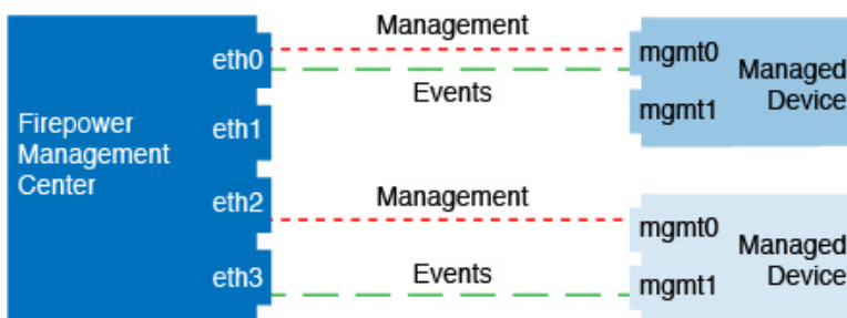
図 20: 管理インターフェイスとイベントインターフェイスを混在させて使用する場合
