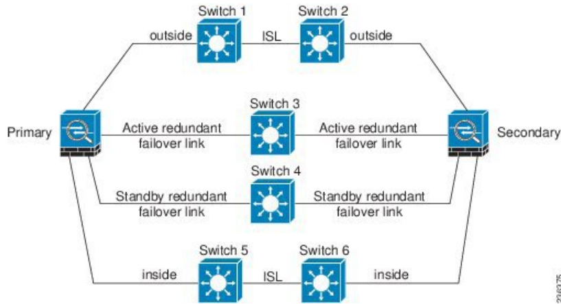
図 13: Inter-Switch Link (ISL) を使用した接続
