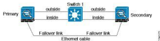
図 10: ケーブルを使用した接続
