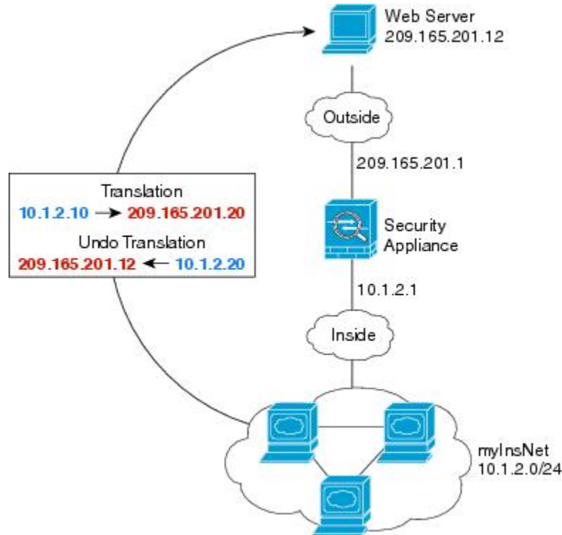
図 35: 内部の動的 NAT、外部 Web サーバの静的 NAT
