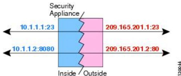
図 28: ポート変換を設定したスタティック NAT の一般的なシナリオ
