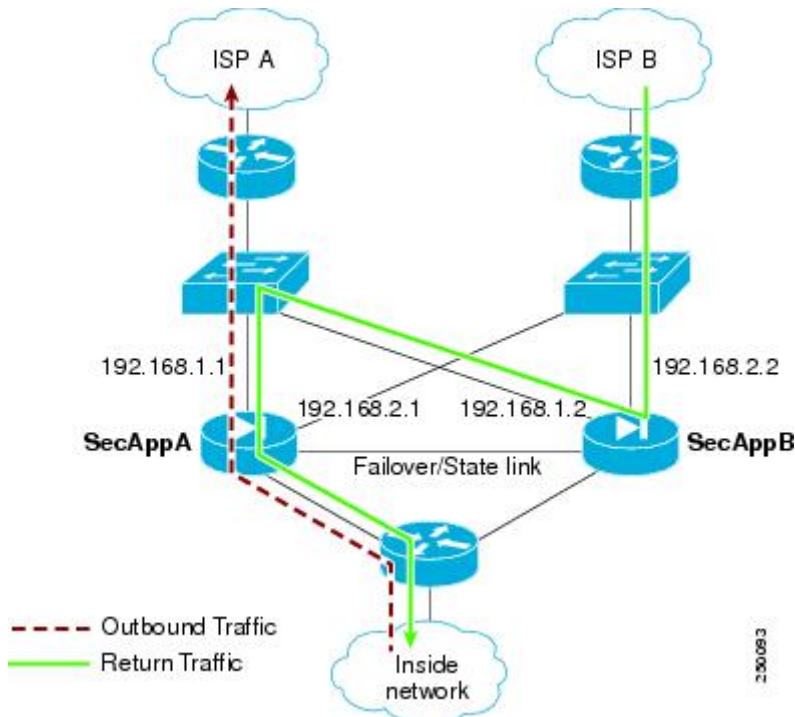
図 13: ASR の例
