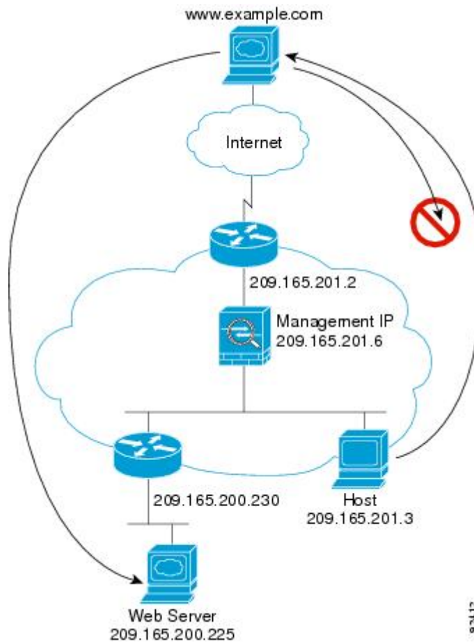
図 41: 一般的なトランスパレントファイアウォールのデータパス
