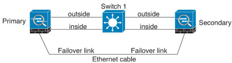
図 56: ケーブルを使用した接続
