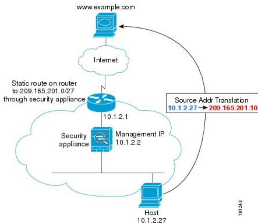
図 43: NAT を使用して内部から外部へ
