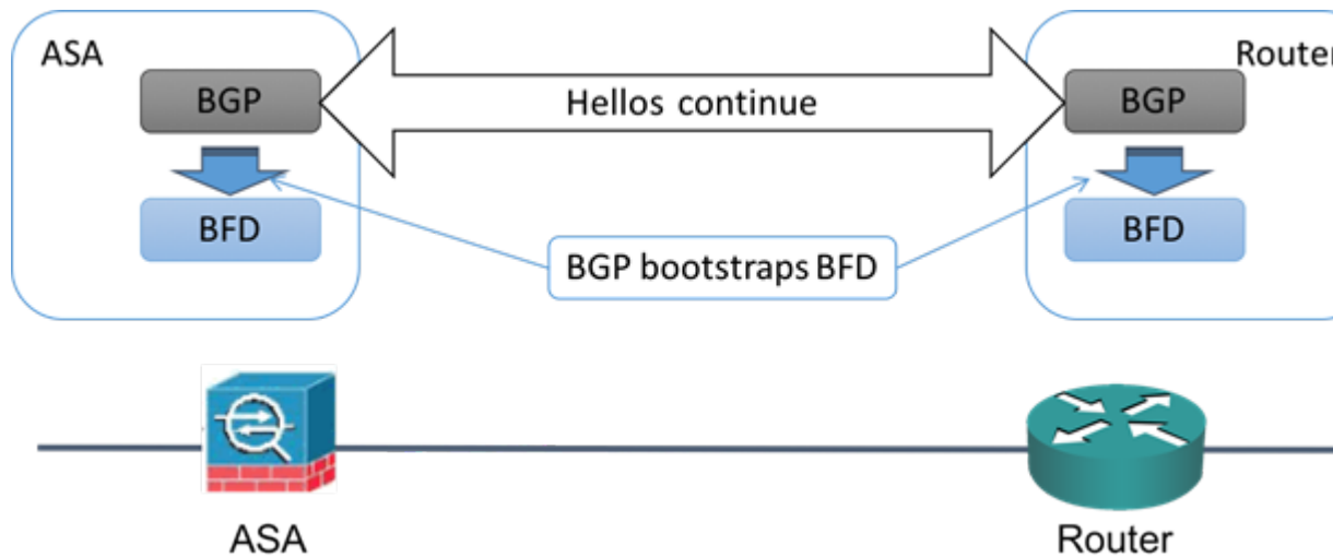
図 81: BFD セッションの確立
