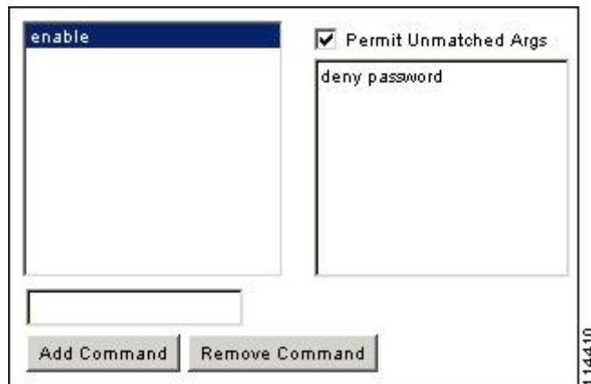
図 90: 引数の拒否
