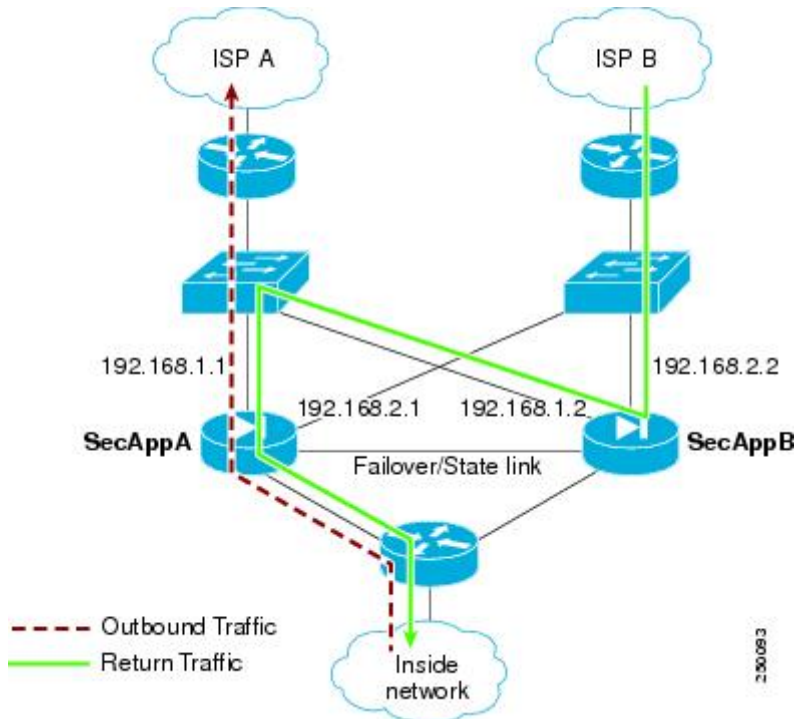
図 58: ASR の例
