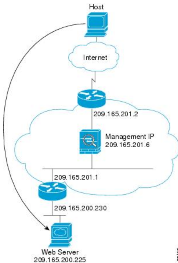
図 44: 外部から内部へ
