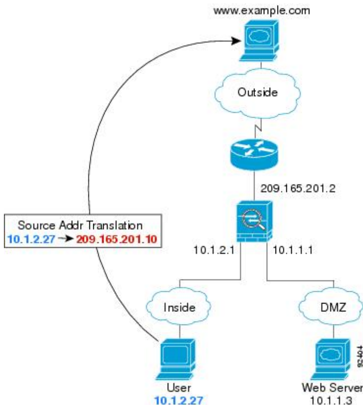
図 36: 内部から外部へ
