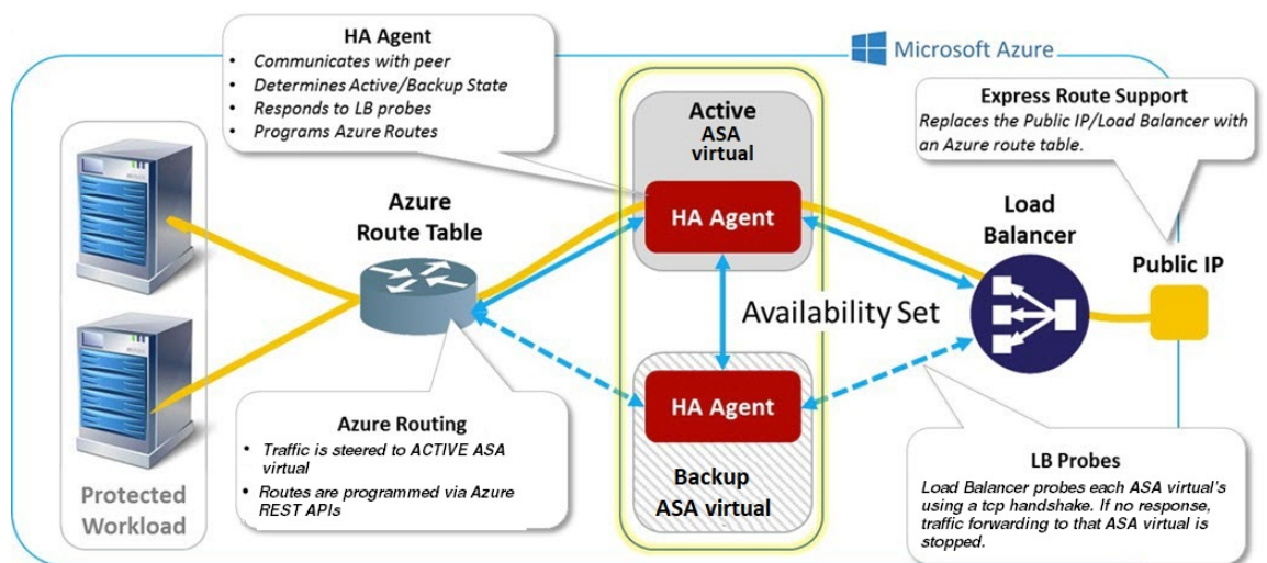
図 59: Azure での ASA 仮想 HA 展開
