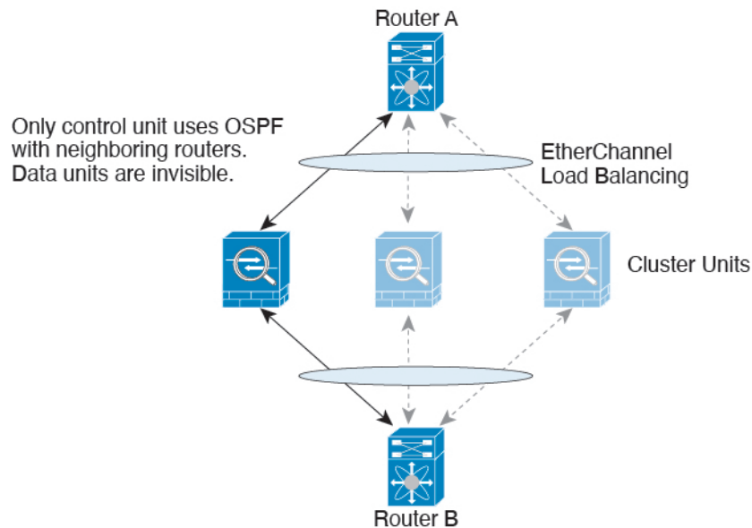
図 62: ダイナミックルーティング
