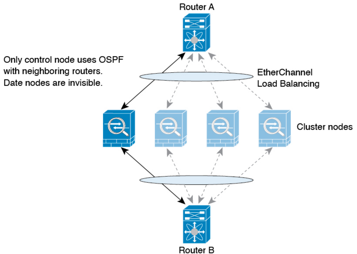
図 79: スパンド EtherChannel モードでのダイナミック ルーティング
