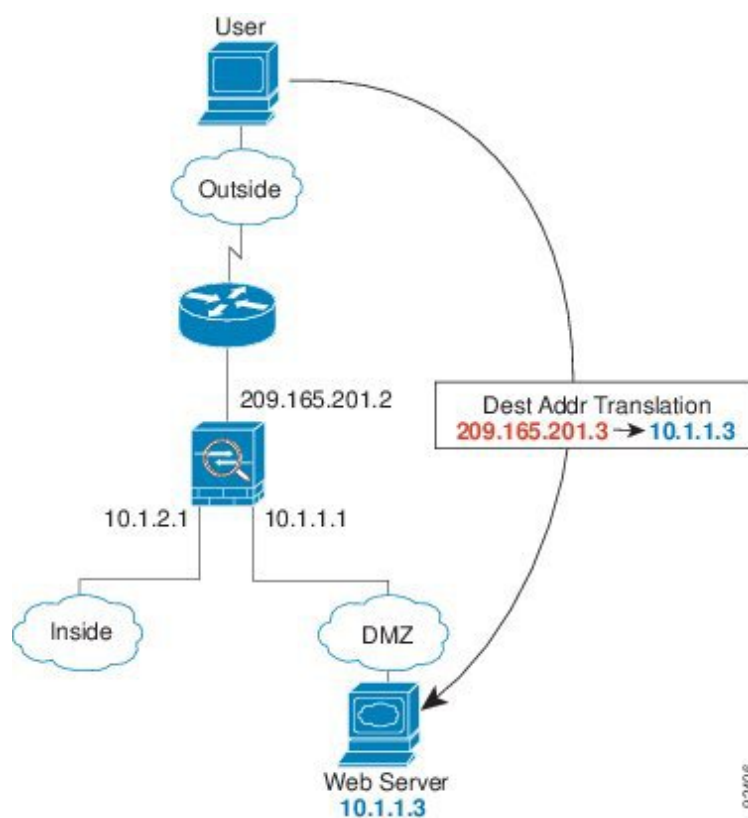
図 37: 外部から DMZ へ
