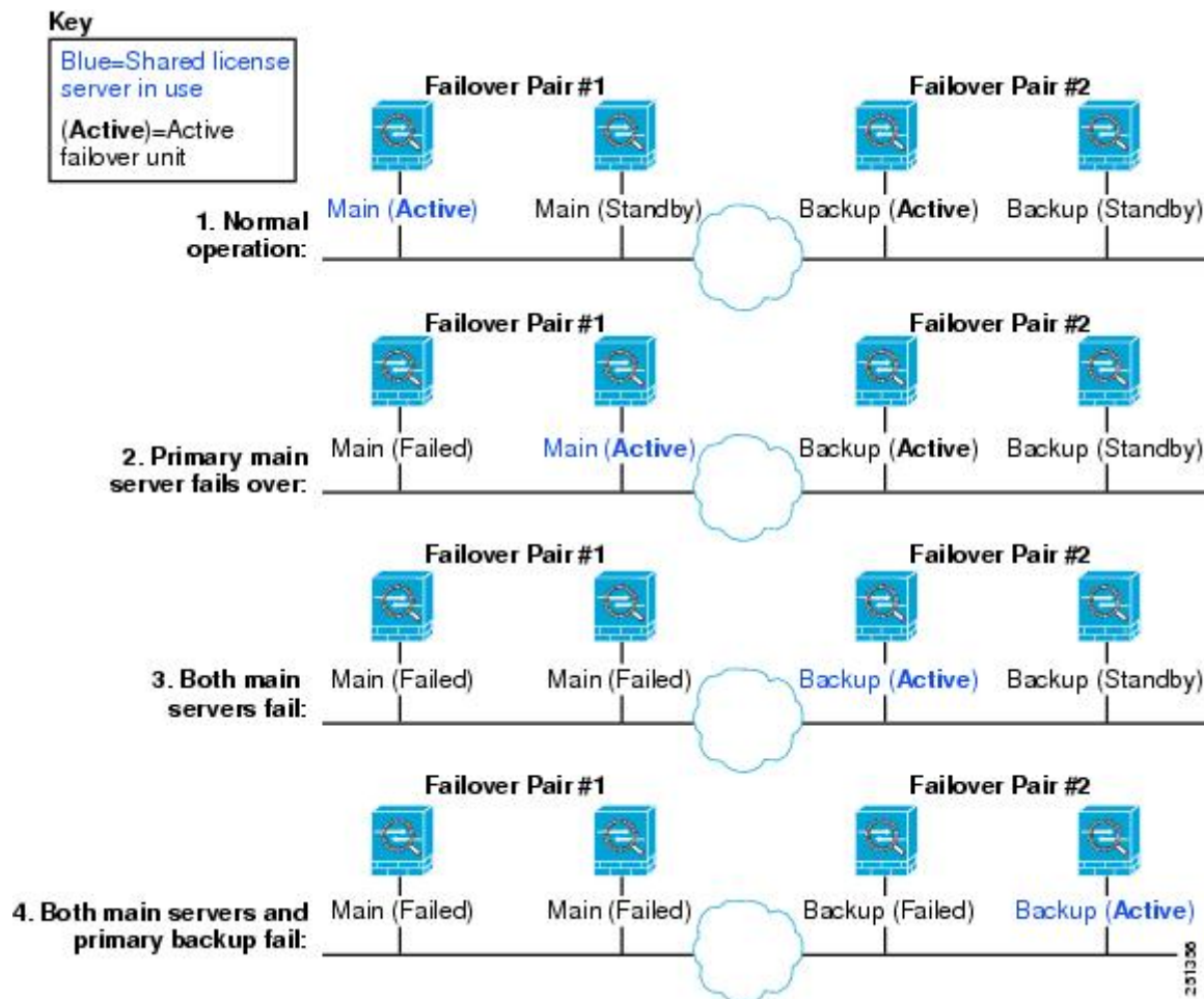
図 15: フェールオーバーと共有ライセンス サーバー
