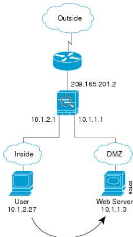
図 38: 内部から DMZ へ
