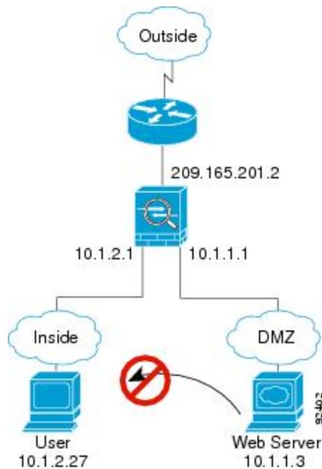
図 40: DMZ から内部へ
