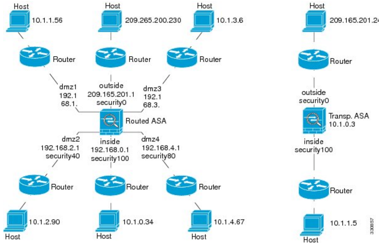
図 92: インターフェイス、ルータ、およびホストを含むネットワーク図
