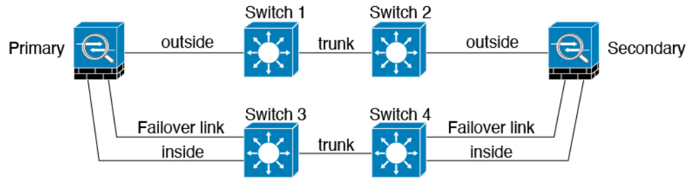
図 57: セキュアスイッチを使用した接続
