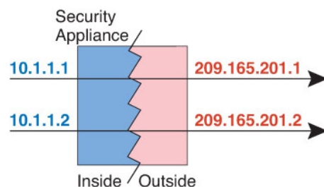
図 8: ダイナミック NAT
