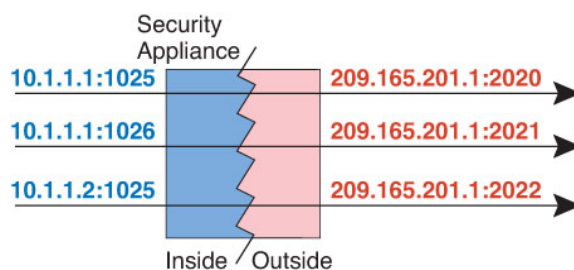
図 10: ダイナミック PAT
