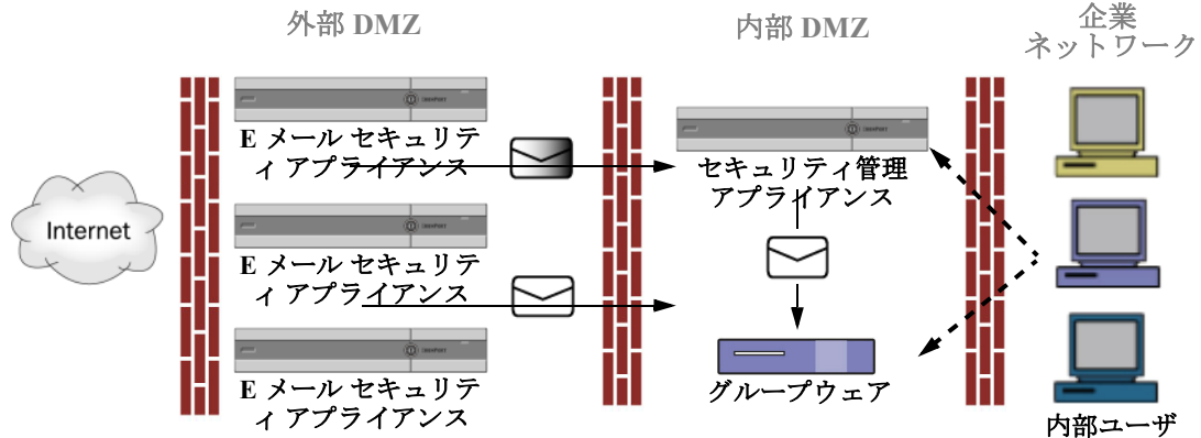
図 42-1 Cisco コンテンツ セキュリティ管理仮想アプライアンスによる一般的なネットワーク設定
