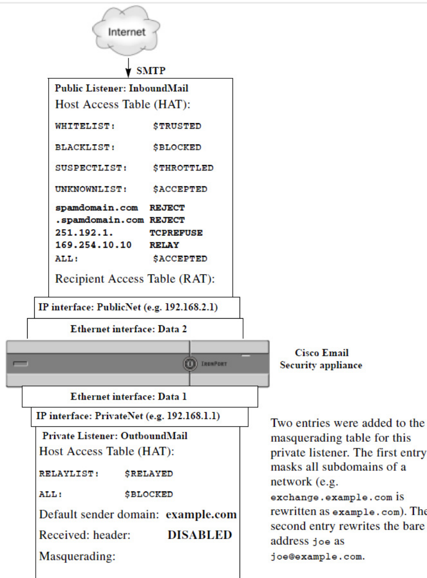
図 25-3 プライベート リスナー用に定義されたマスカレード
