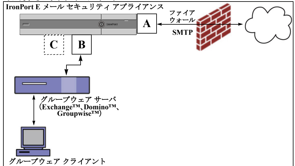
図 40-1 エンタープライズ ゲートウェイに対するブラック ホール リスナー
