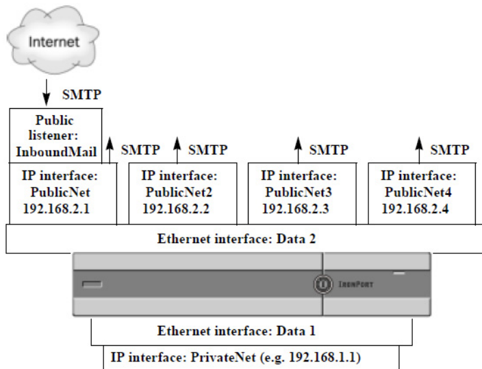
図 25-11 1つのイーサネット インターフェイス上にある4つの Virtual Gateway アドレス
