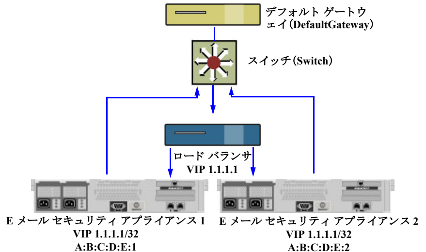
図 37-2 DSR を使用したスイッチ上の複数の E メール セキュリティ アプライアンス間でのロード バランス
