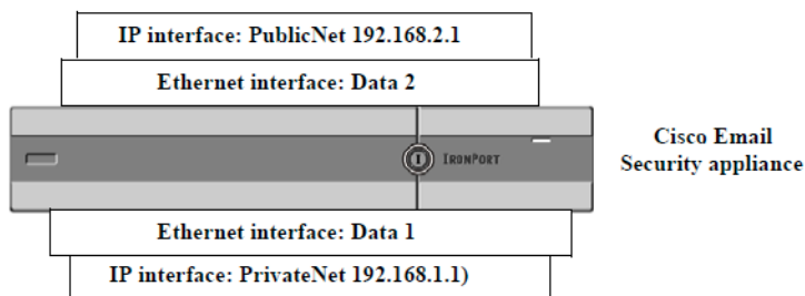
図 25-7 パブリック インターフェイスとプライベート インターフェイスの例
