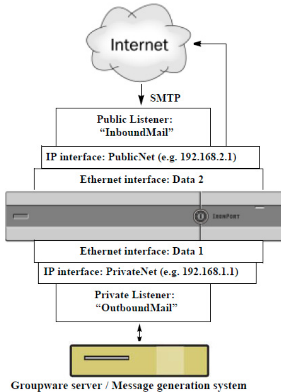
図 5-2 3 つ以上のイーサネット インターフェイスを持つアプライアンス モデル上のパブリックおよびプライベート リスナー
