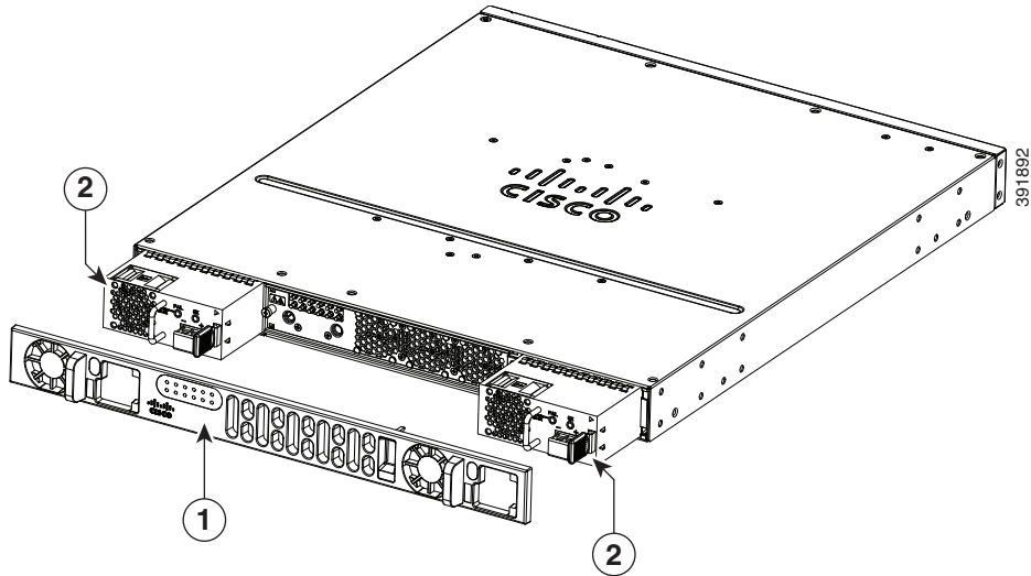
図 6-32 ベゼルの取り外し
