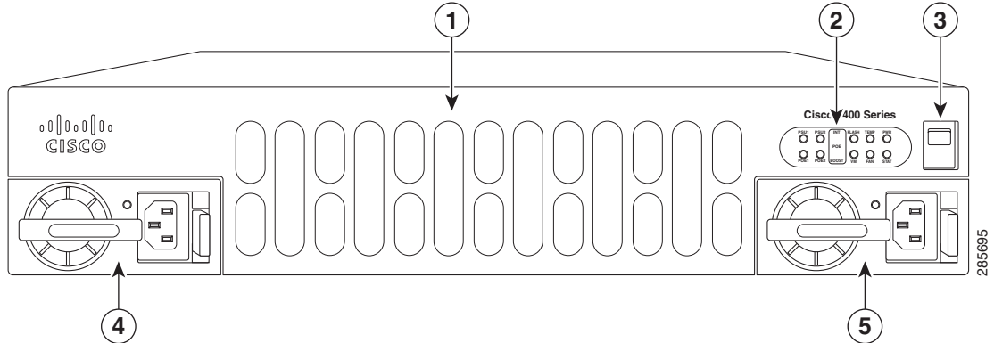
図 6-28 Cisco ISR 4451-X電源装置
