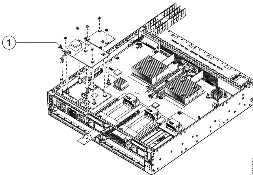
図 6-42 PoE ドーター カードの位置 (Cisco ISR 4451-X)
