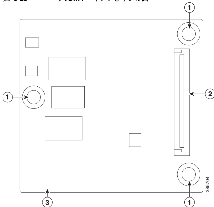
図 6-23 PVDM4 コネクタとネジの図
