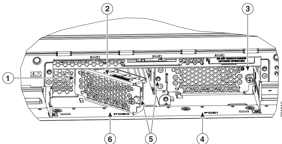
図 6-35 PoE フィラーの取り付けおよび取り外し
