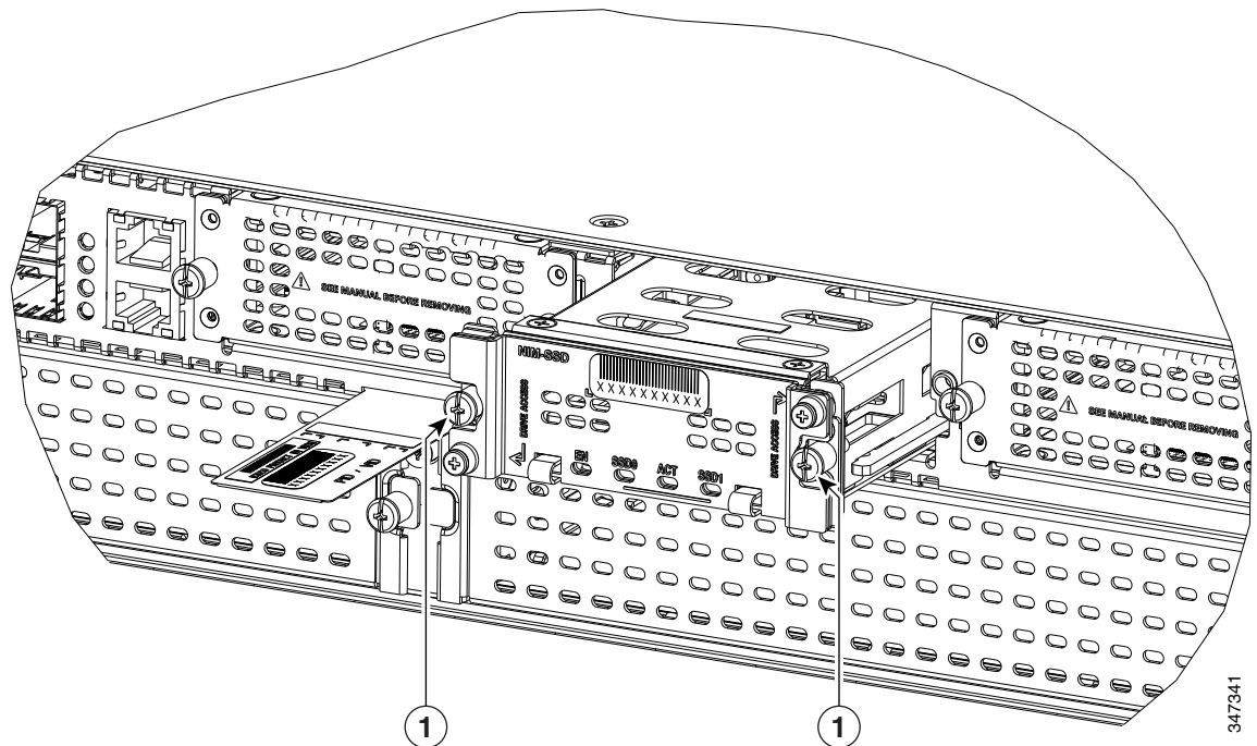
図 6-17 ルータからの NIM-SSD または NIM-HDD の取り外し
