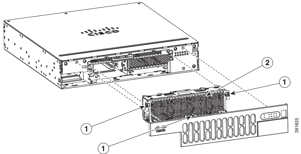
図 6-37 Cisco ISR4351 ファントレイ
