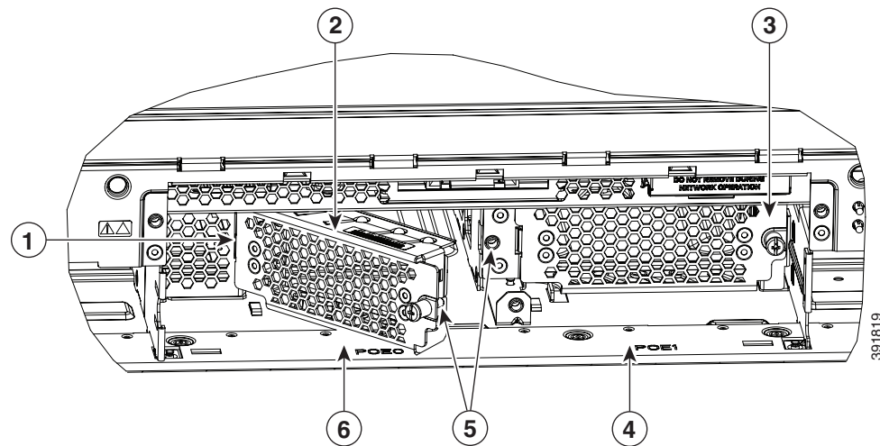
図 6-35 PoE フィラーの取り付けおよび取り外し
