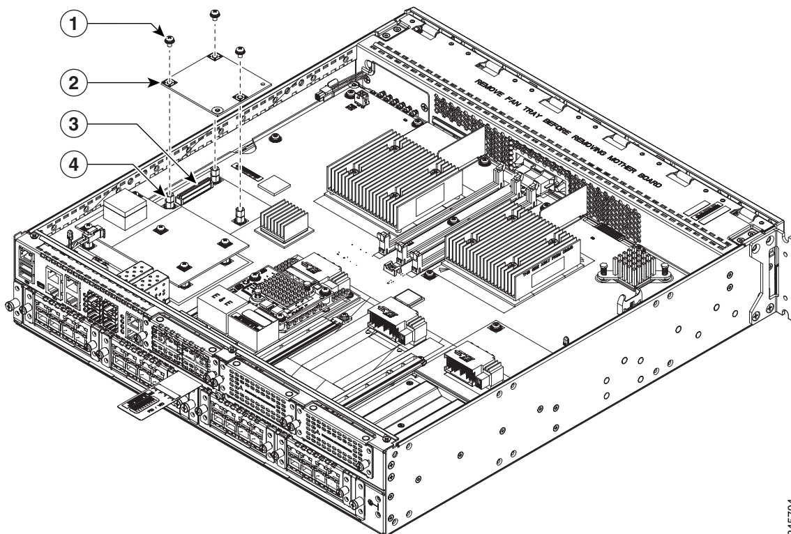
図 6-24 Cisco ISR 4451-X での PVDM4 の位置
