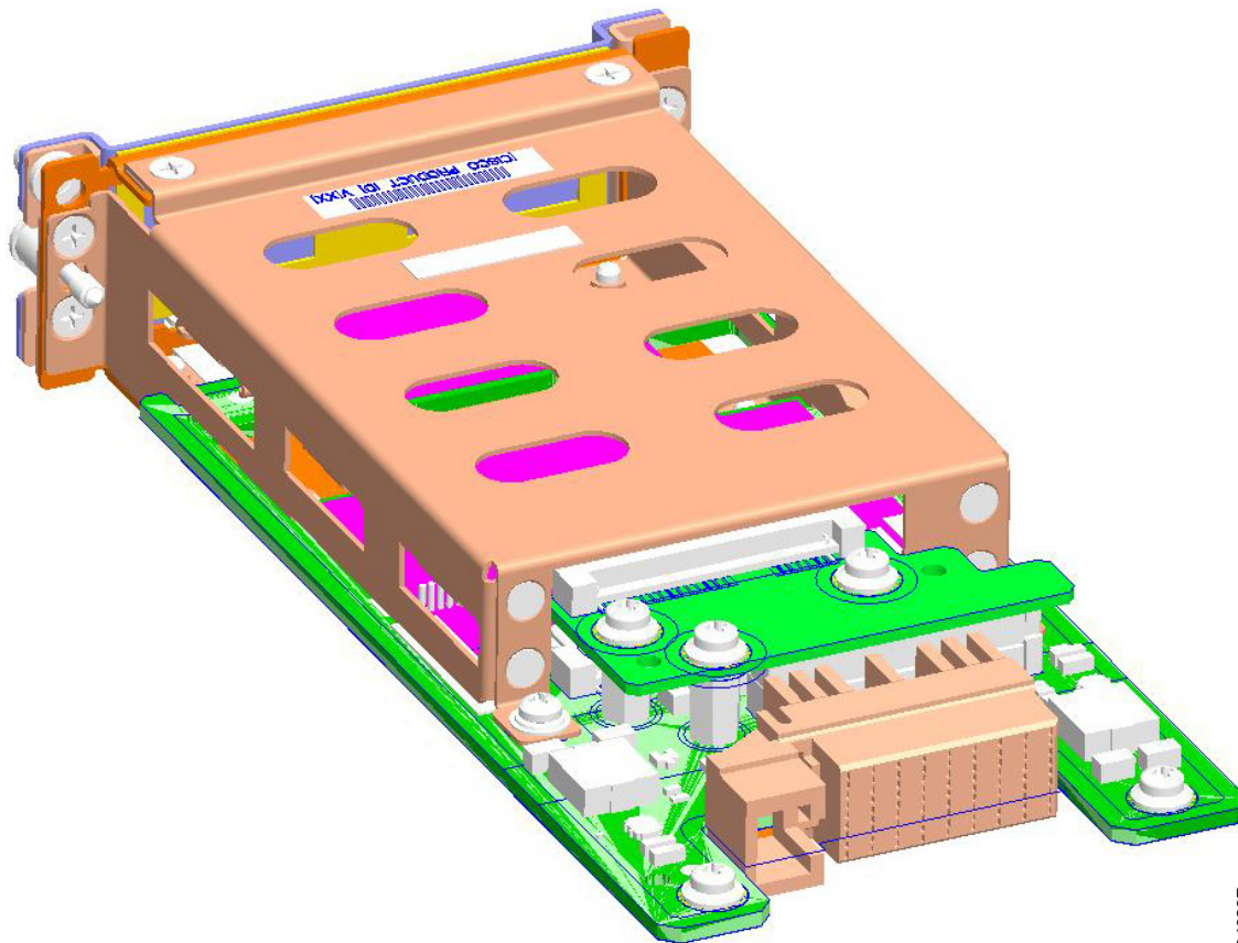
図 6-5 SSD キャリアカード NIM の背面図
