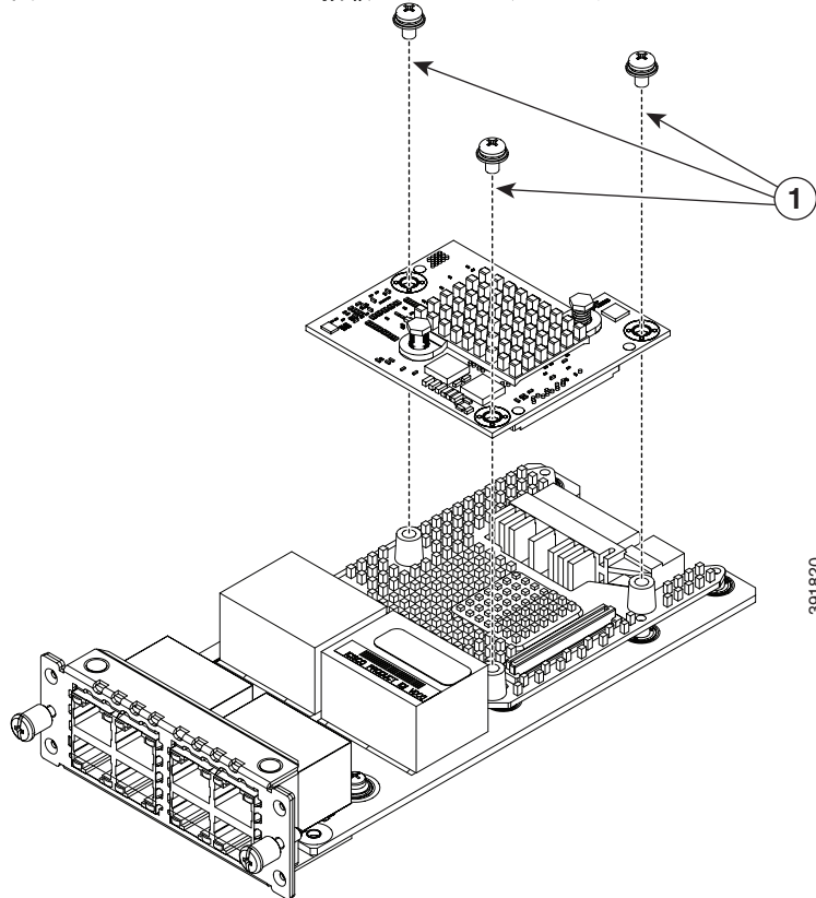
図 6-25 PVDM4 搭載ネットワーク インターフェイス モジュール
