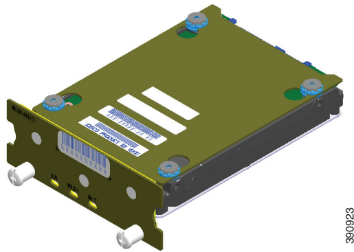
図 6-13 HDD カード
