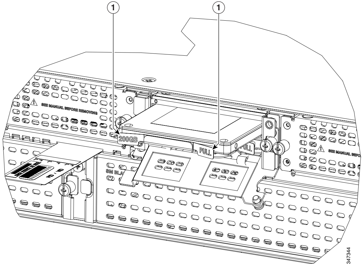
図 6-11 ソリッドステートドライブを引き出す
