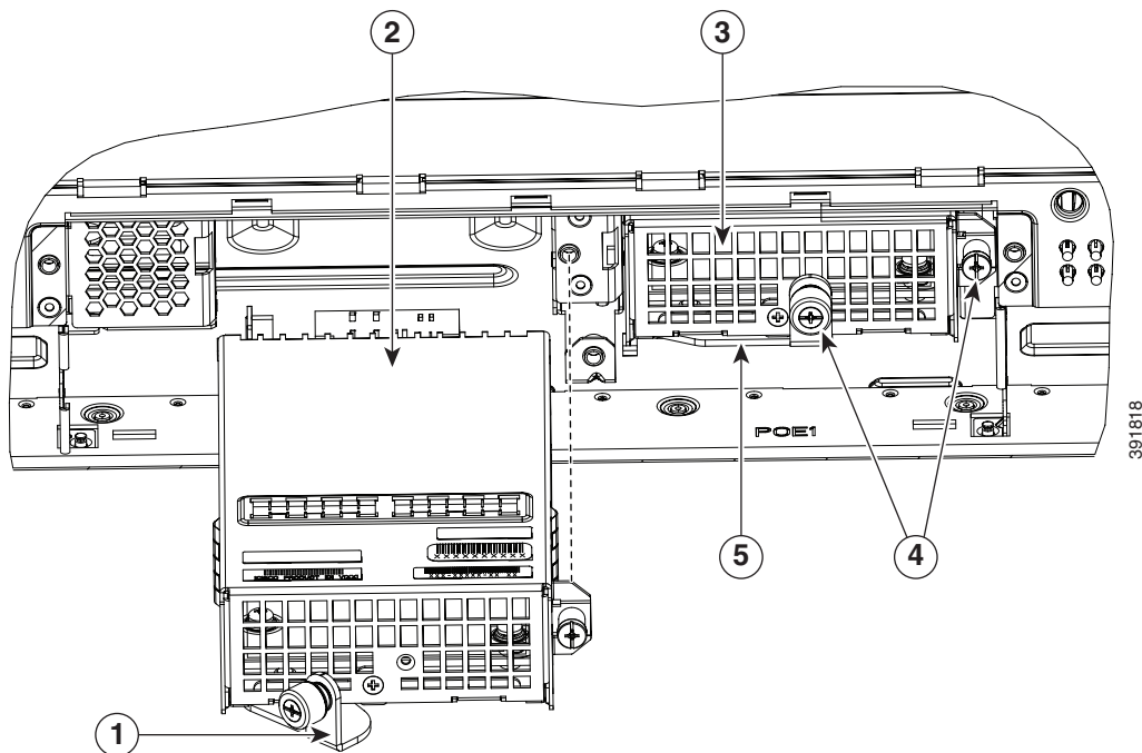
図 6-36 PoE コンバータ電源の取り付け
