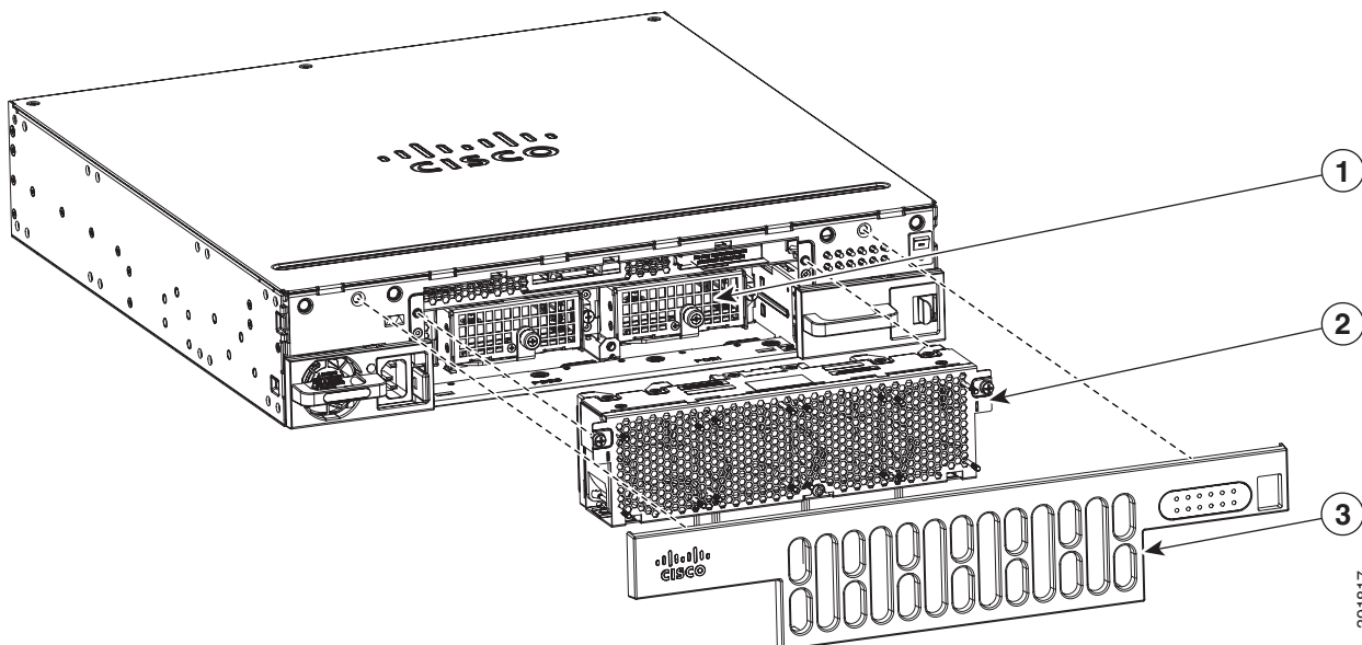
図 6-34 ベゼルおよびファントレイの取り外しと PoE スロットの位置の確認
