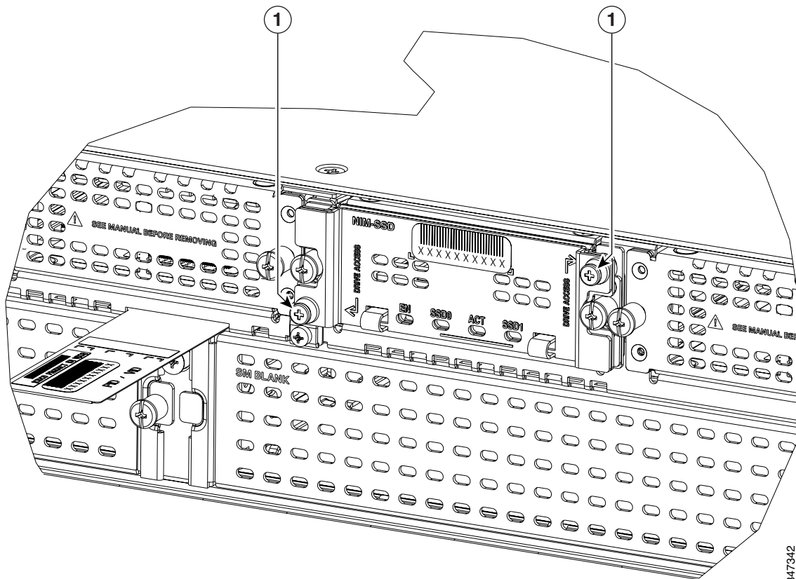
図 6-9 SSD スロット カバーを開く
