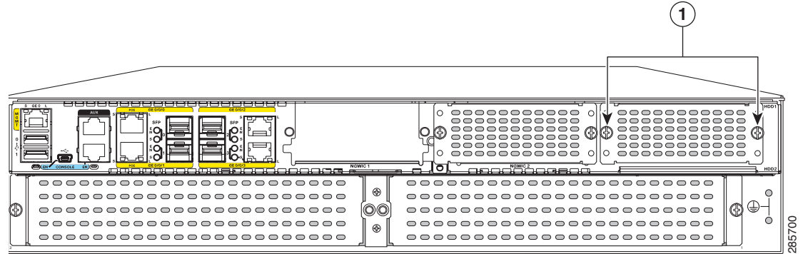
図 6-16 ルータからの NIM-SSD または NIM-HDD の取り外し
