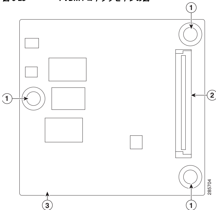
図 6-23 PVDM4 コネクタとネジの図
