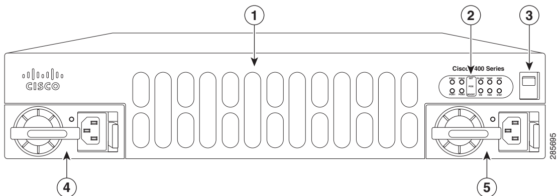
図 6-28 Cisco ISR 4451-X電源装置
