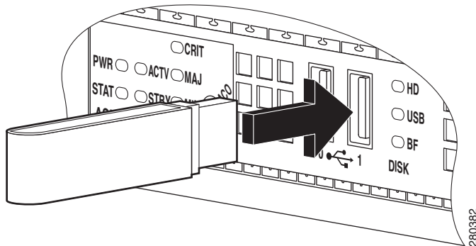
図 6-26 ルータ フラッシュ トークン メモリ スティック
