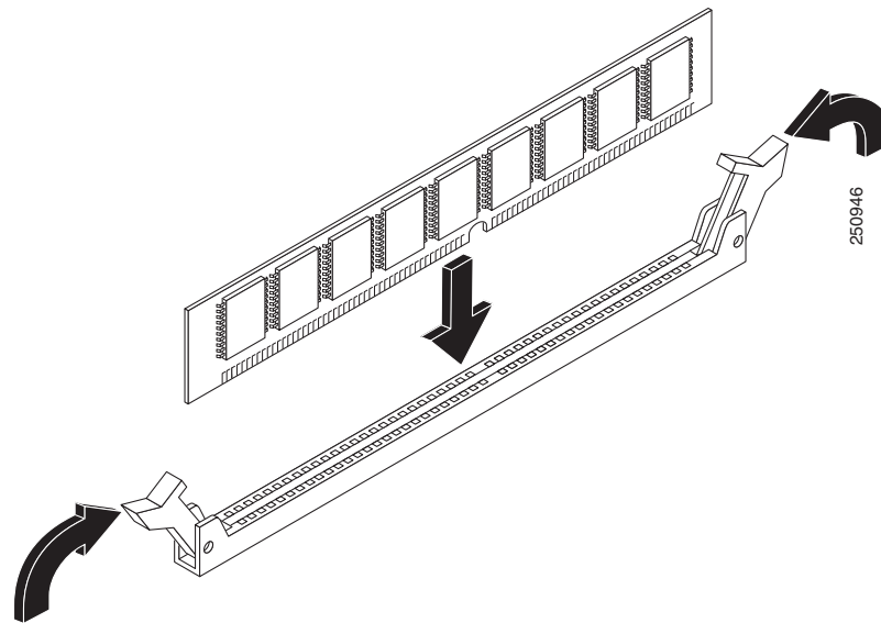
図 6-22 DIMM の取り付け
