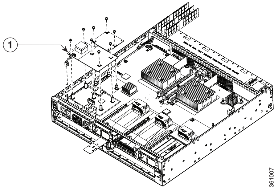
図 6-42 PoE ドーター カードの位置 (Cisco ISR 4451-X)
