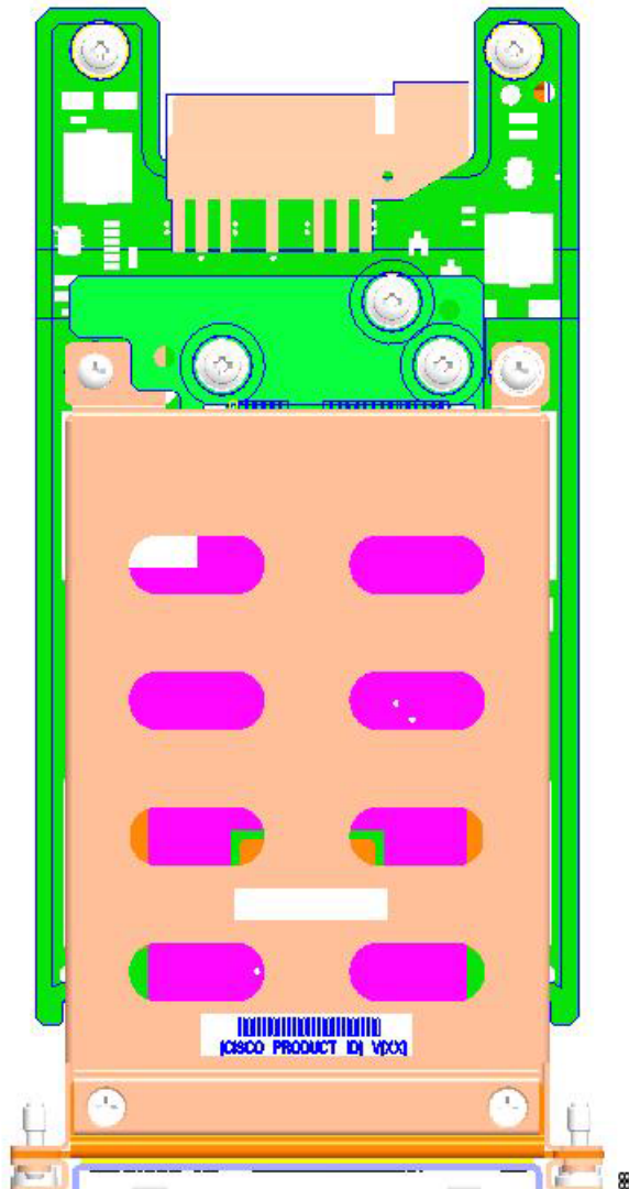
図 6-6 シリアルナンバーの付いた SSD キャリアカード NIM の上面図
