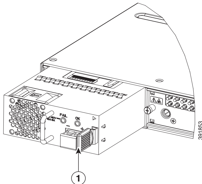
図 6-30 DC 電源の取り外し
