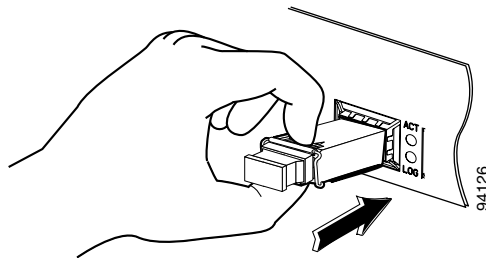
図 6-40 SFP モジュールの装着
