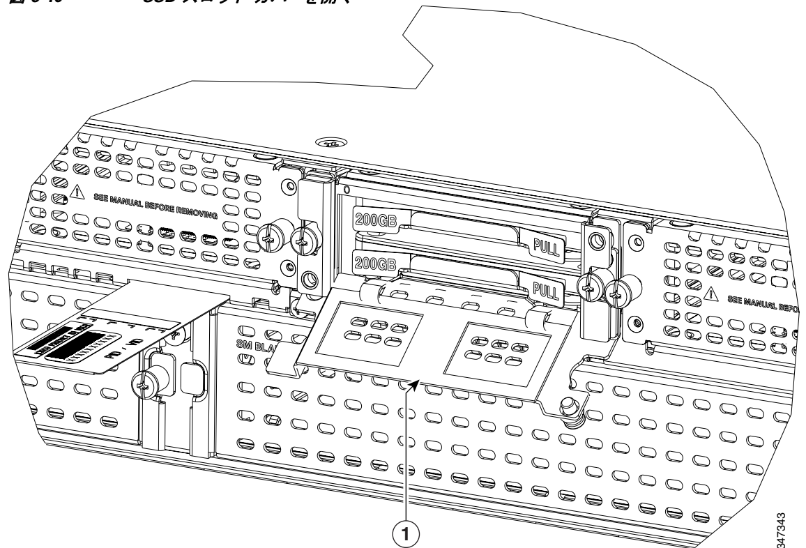
図 6-10 SSD スロット カバーを開く
