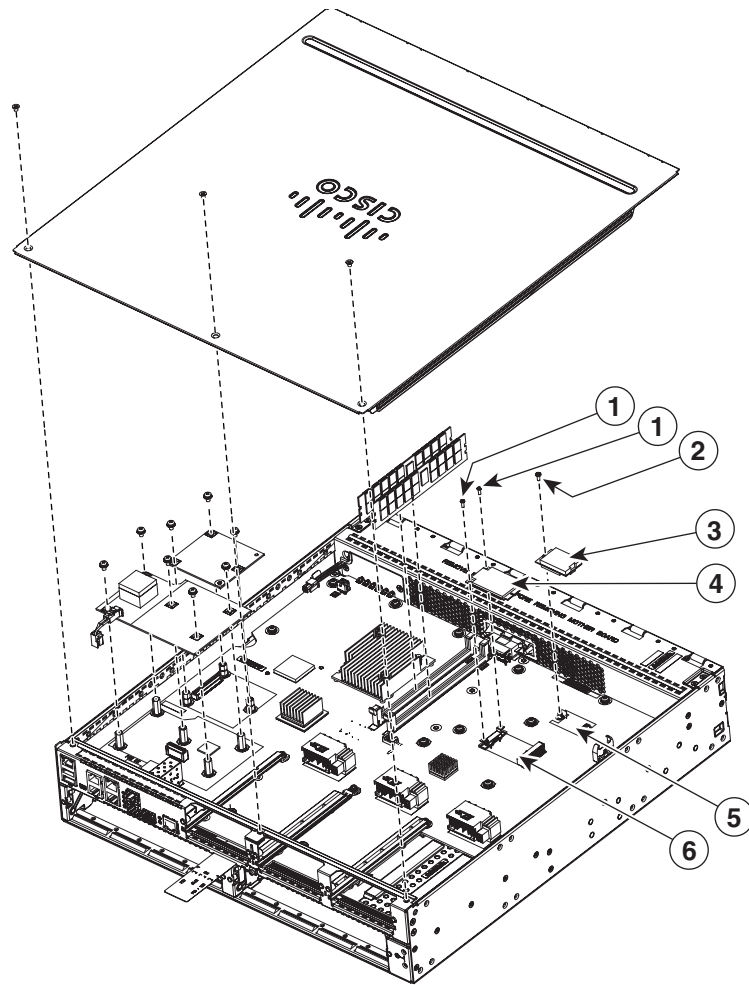
図 6-38 メモリカード
