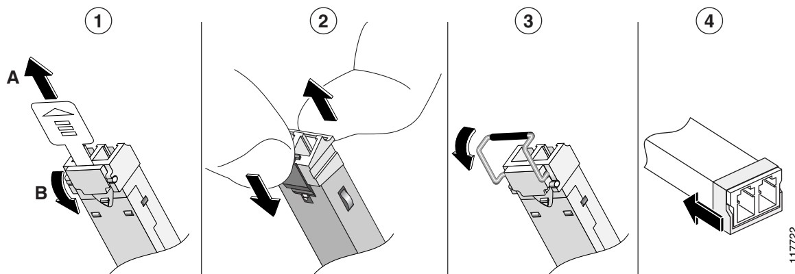
図 6-41 SFP ラッチ メカニズムの接続解除
