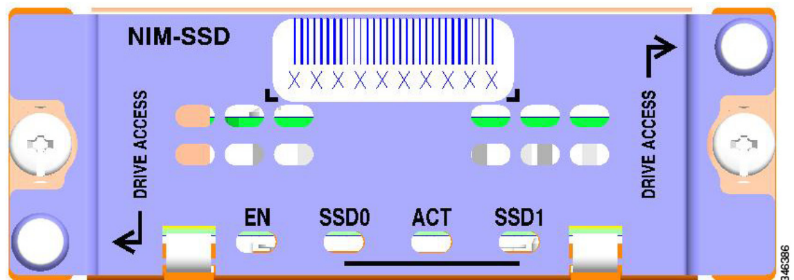
図 6-4 SSD キャリアカード NIM の前面パネル
