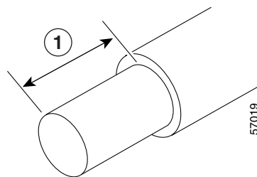
図 6-31 被覆を剥がした状態の DC 入力電源線
