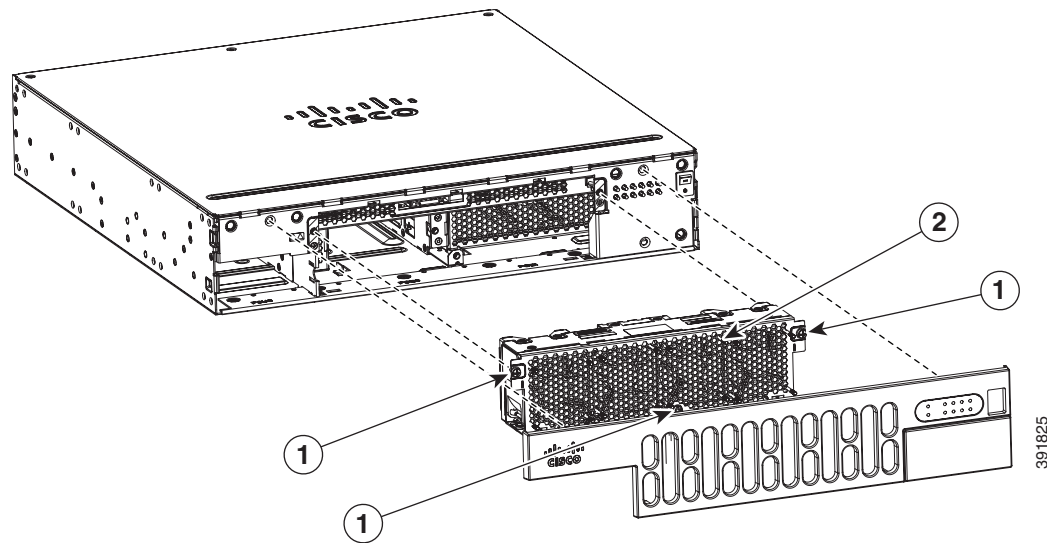
図 6-37 Cisco ISR4351 ファントレイ
