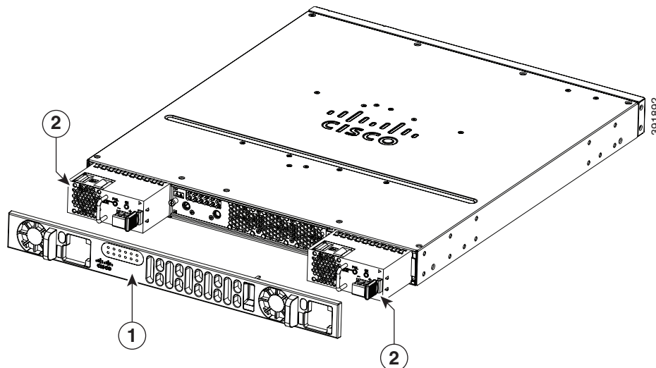
図 6-32 ベゼルの取り外し
