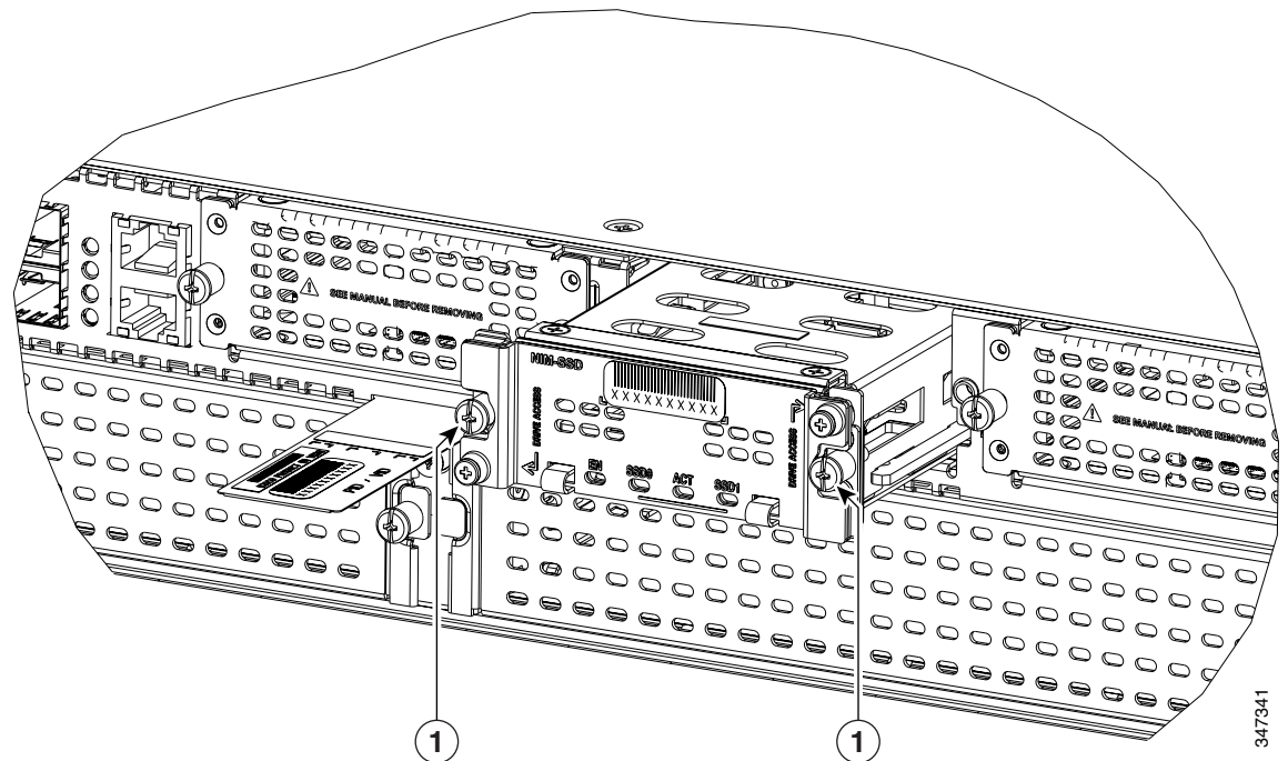
図 6-17 ルータからの NIM-SSD または NIM-HDD の取り外し
