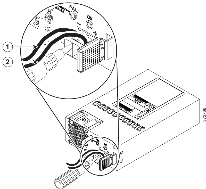
図 6-33 導線を使用する DC 電源
