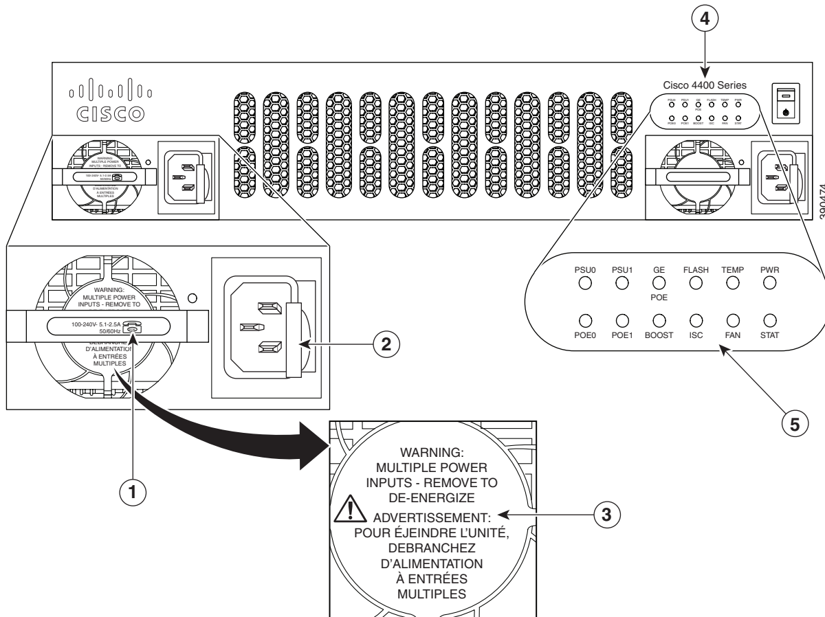
図 6-27 電源装置 (Cisco ISR4451-X)
