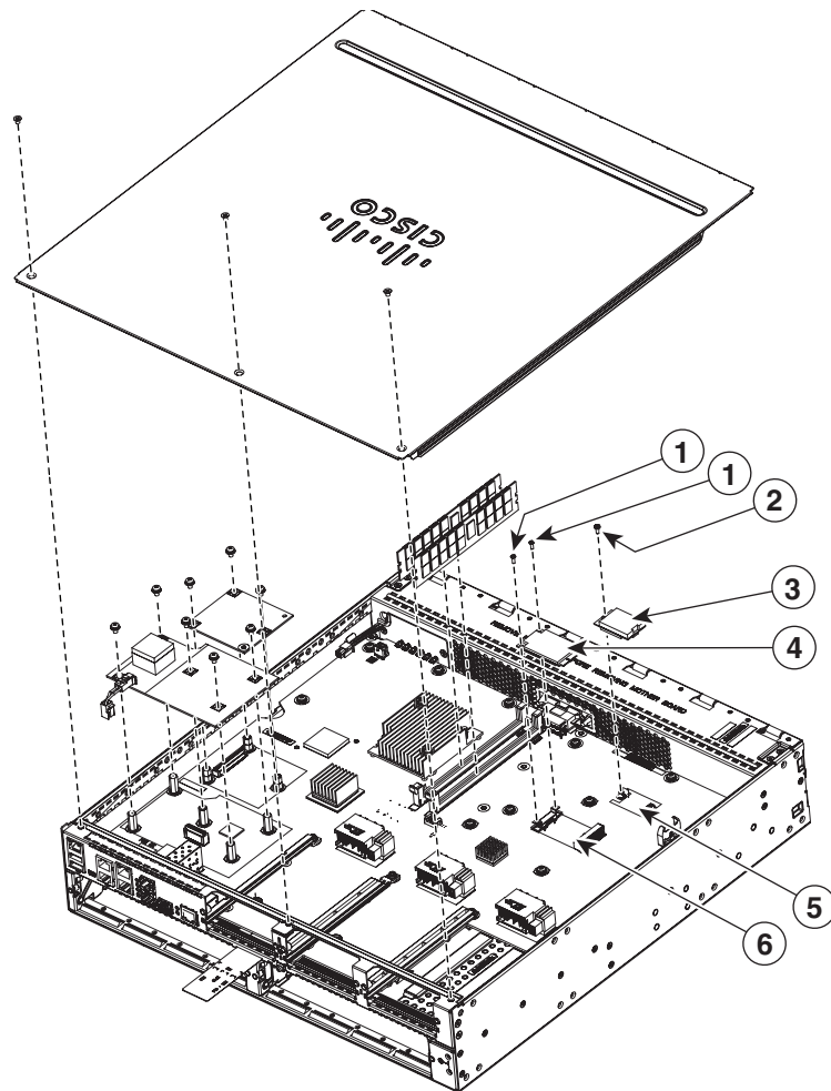
図 6-39 フラッシュ メモリ カードと SSD mSATA ストレージ デバイスの位置
