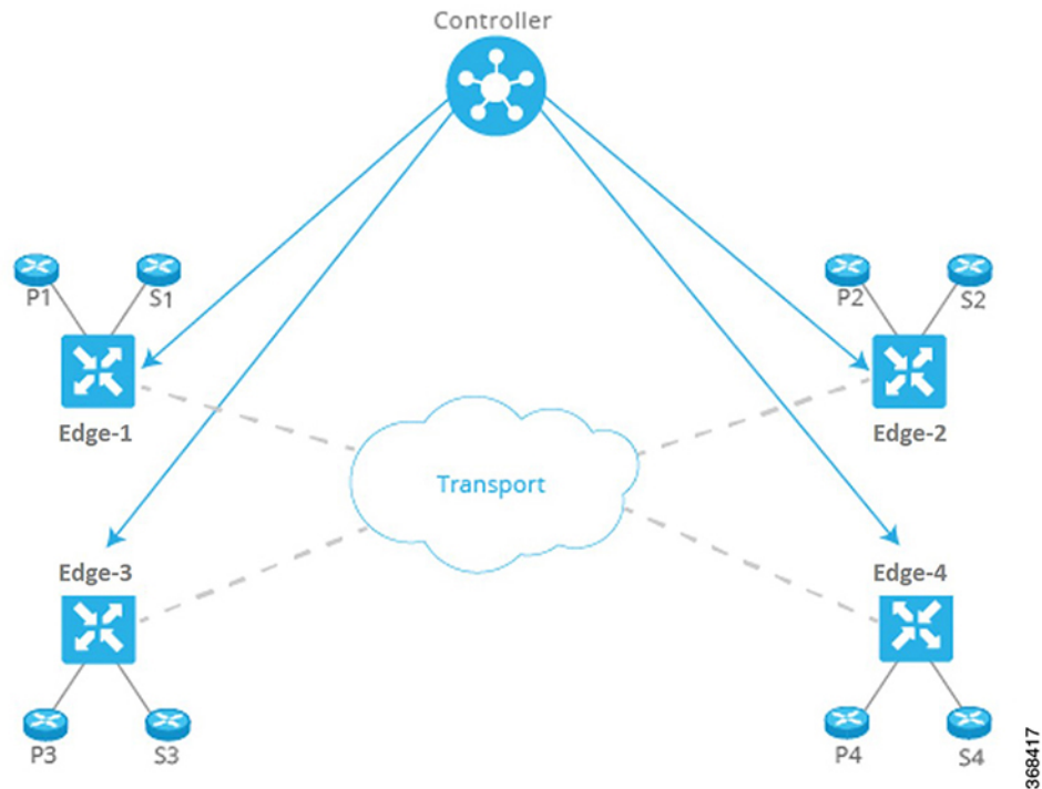
図 1: Cisco Catalyst SD-WAN ソリューションのコンポーネント
