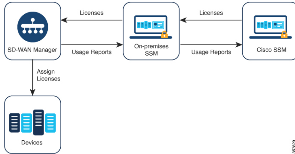
図 32: Cisco SSM オンプレミス ライセンス サーバーを使用する Cisco Catalyst SD-WAN Manager
