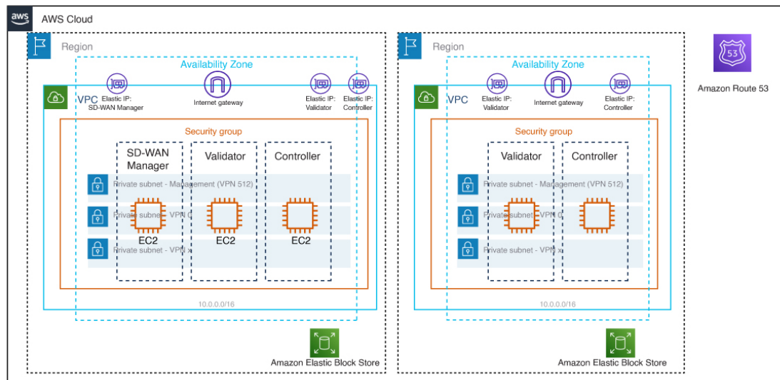
図 36: AWS での Cisco SD-WAN コントローラ
