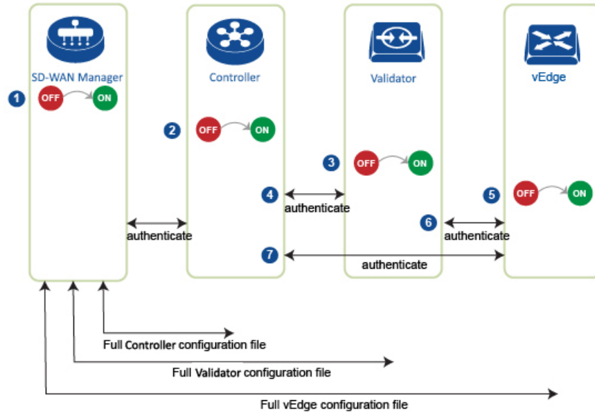
図 10: 稼働イベントシーケンス
