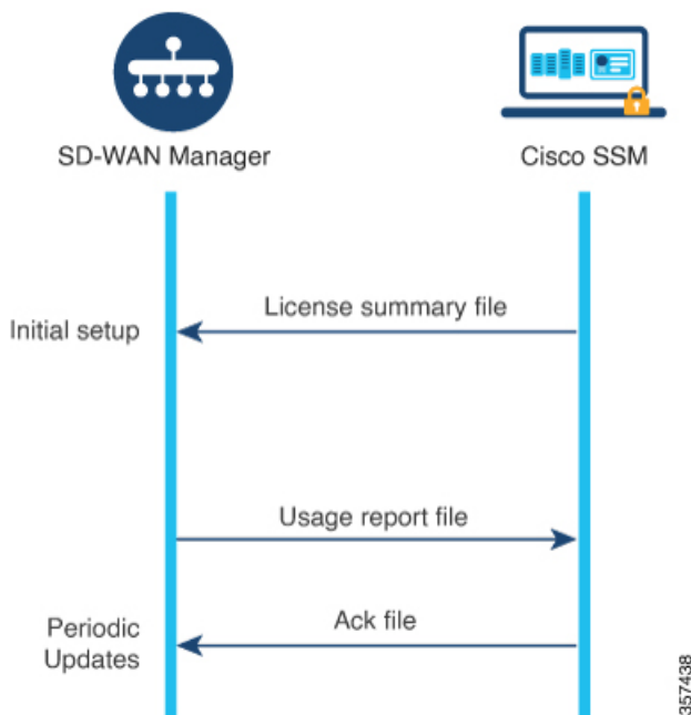
図 30 : Cisco SD-WAN Manager および Cisco SSM から確認応答ファイルをアップロードおよび受信する
