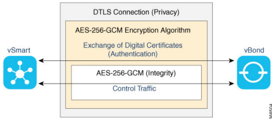
図 4: Cisco SD-WAN コントロールプレーンの概要
