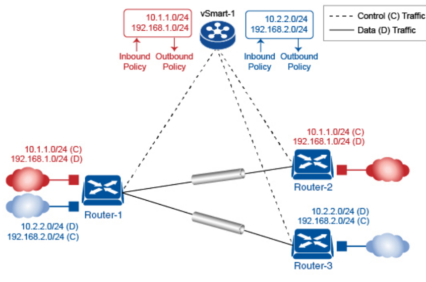
図 6: VRF 内のルーティング情報の伝播
