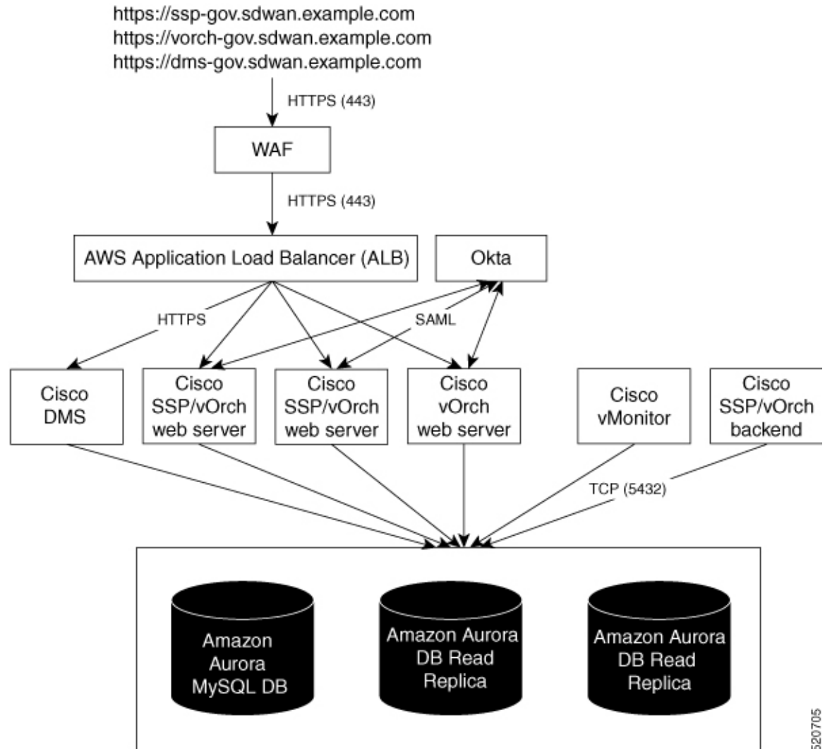
図 2: Cisco SD-WAN SSP の概要
