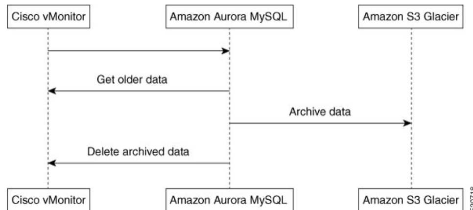
図 10: データ消去のワークフロー
