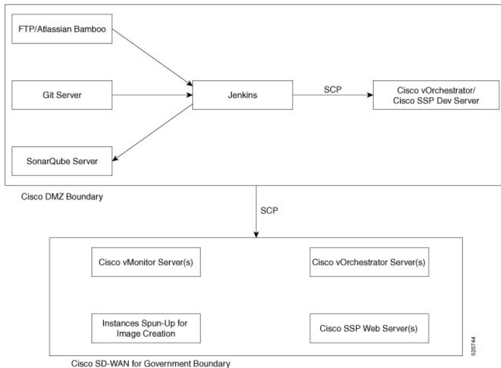
図 12 : Cisco SD-WAN 継続的統合および継続的導入パイプライン
