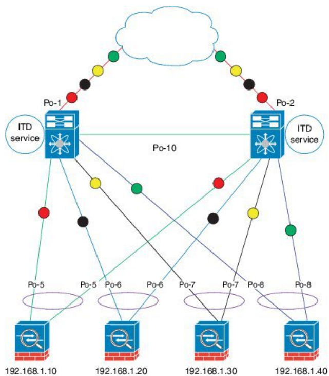
図 16: VPC でのワンアーム展開モード
