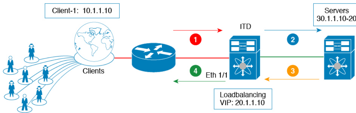
図 6: 仮想 IP アドレスによる NAT
