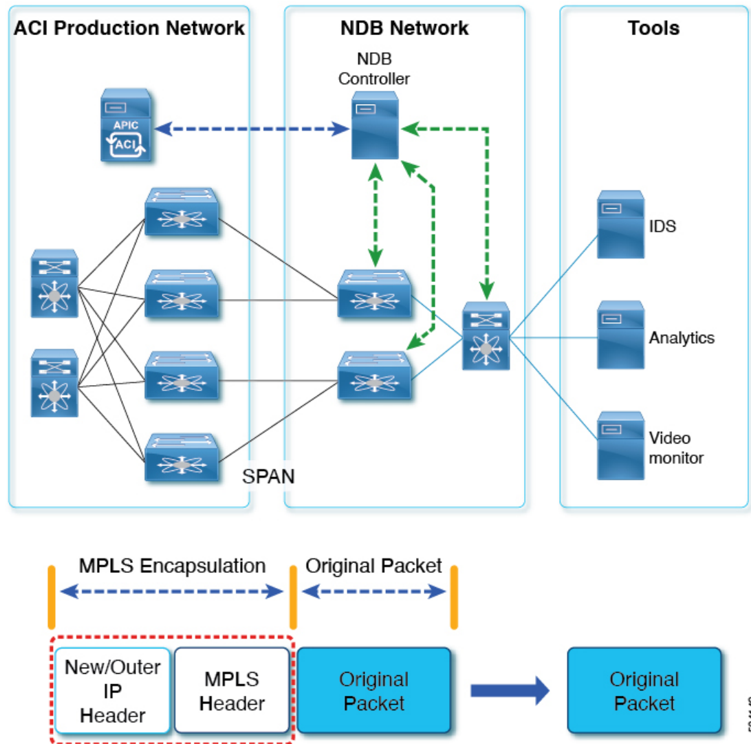
図 3: NDB MPLS ヘッダストリッピングソリューション
